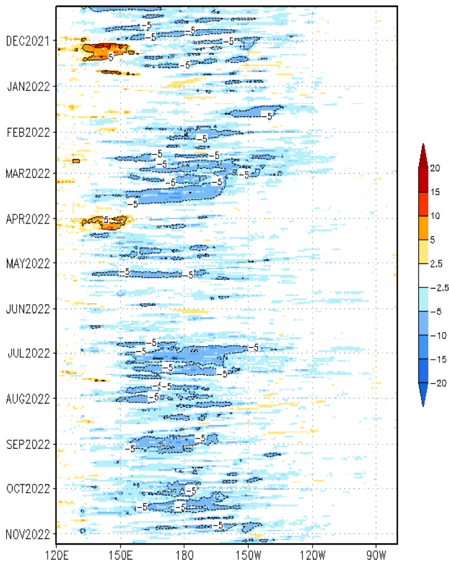
Figura 3. Diagrama longitud-tiempo de las anomalías del esfuerzo de viento zonal ecuatorial que se obtiene de los datos del producto ASCAT hasta el 08 de noviembre de 2022. Elaborado por el IGP.
