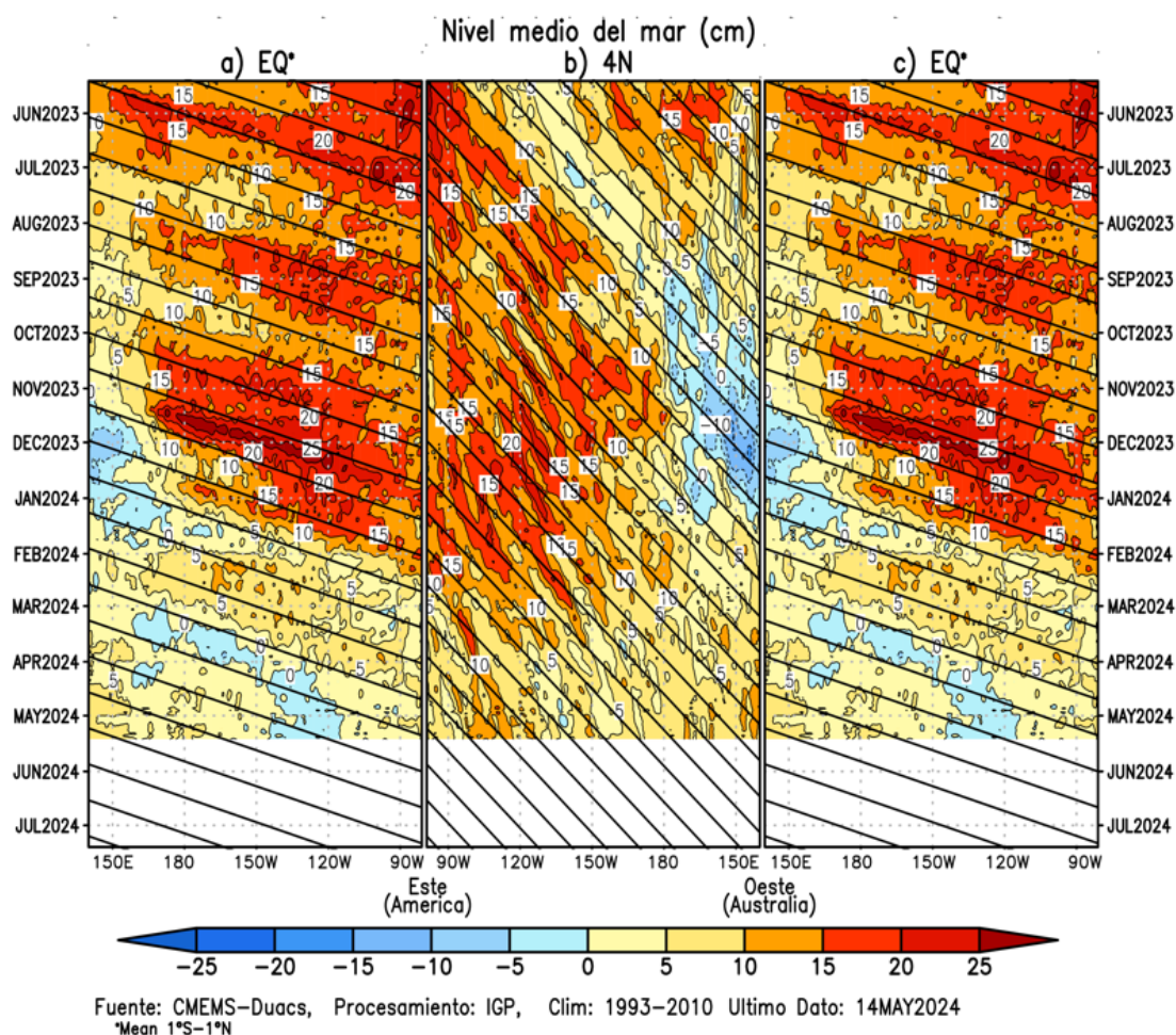
Figura 7. Diagramas longitud-tiempo de la anomalía del nivel medio del mar en el Pacífico ecuatorial usando el producto DUACS. Los paneles (a) y (c) son los mismos y representan la información a lo largo de la línea ecuatorial; mientras que (b), a lo largo de 4°N, pero con el eje zonal de este a oeste. Las líneas diagonales indican la trayectoria teórica de la onda de Kelvin (a y c) y Rossby (b) si tuvieran una velocidad aproximada de 2.6 m/s y 0.87 m/s, respectivamente. Elaborado por el IGP.
