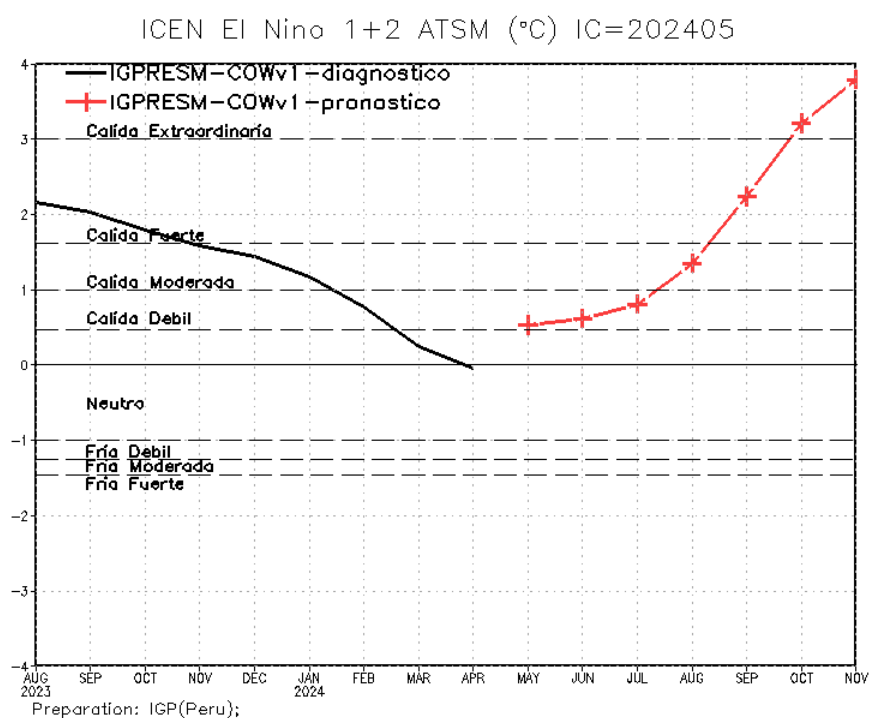
Figura 16. Pronóstico del ICEN de mayo a noviembre, generado por el Modelo Regional Earth System Model CROCO-OASIS-WRF v.1' (IGP RESM-COW v.1) con condiciones iniciales de mayo.
