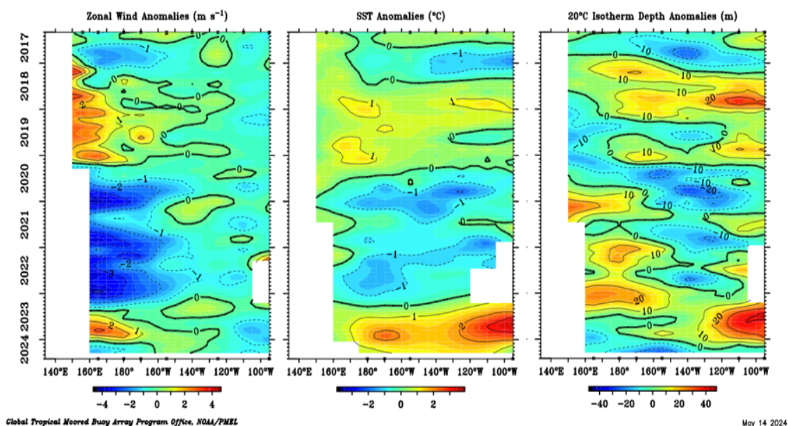
Figura 2. Promedio mensual de la anomalía del viento zonal (panel izquierdo), de la temperatura superficial del mar (panel central) y de la profundidad de la isoterma de 20 ^{\circ}C (panel derecho) y a lo largo de la franja ecuatorial del Pacífico (2°S-2°N). Esta imagen se elaboró de otras que se obtienen del proyecto TAO: www.pmel.noaa.gov/
