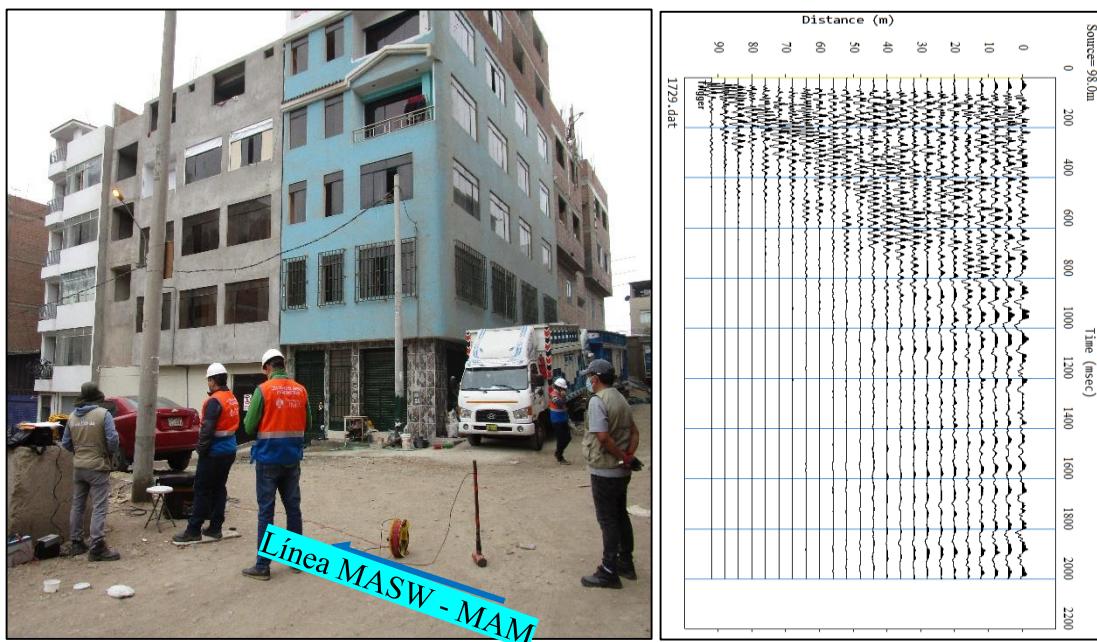
Figura 33. Disposición del equipo de adquisición de datos MASW y MAM, para la línea sísmica ubicada en el Condominio Pacasmayo y el registro obtenido.
