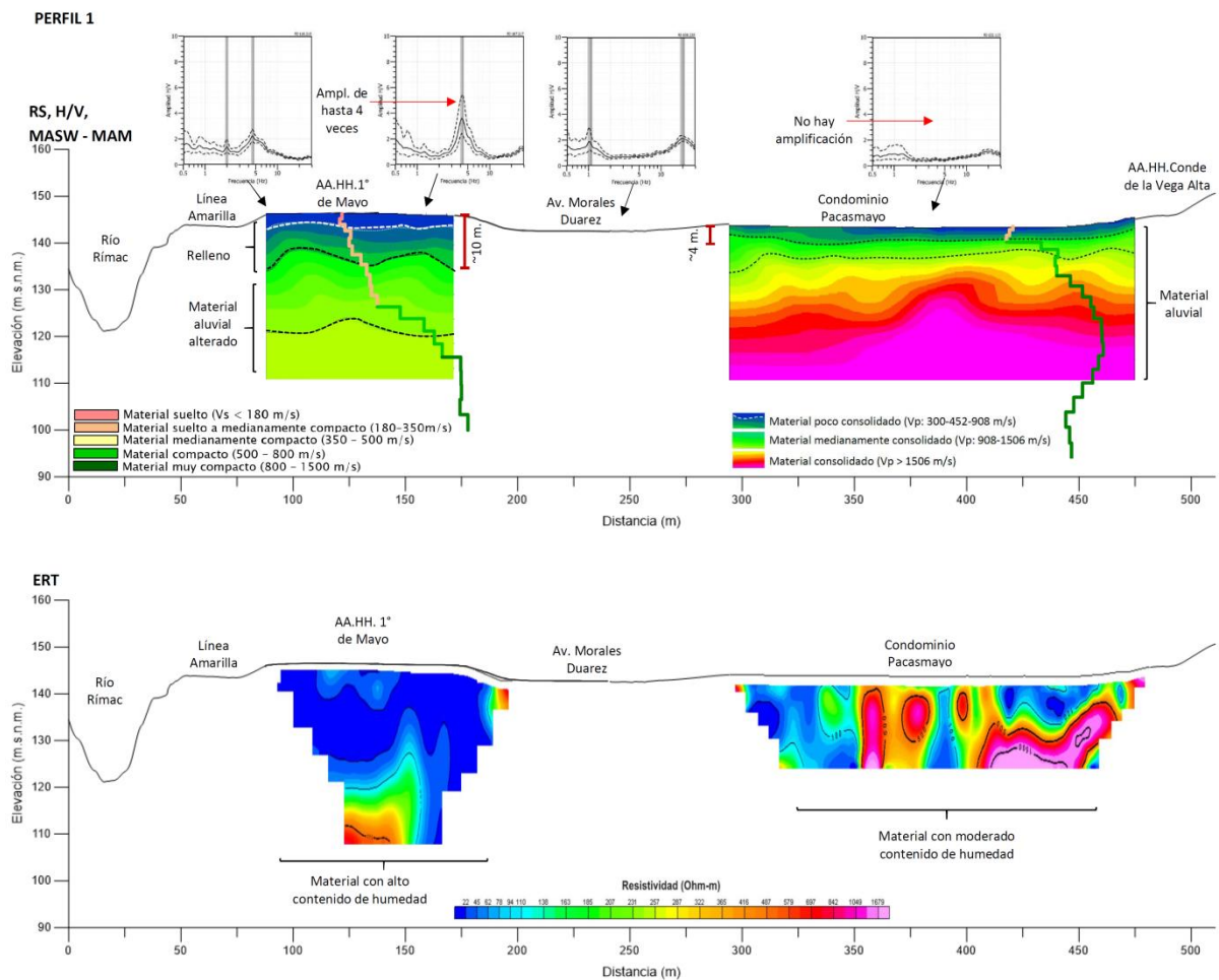
Figura 45. Vista del Perfil-01 y correlación de los resultados obtenidos con los métodos de H/V, ERT, RS y MASW-MAM para el extremo Este de la MIRR
