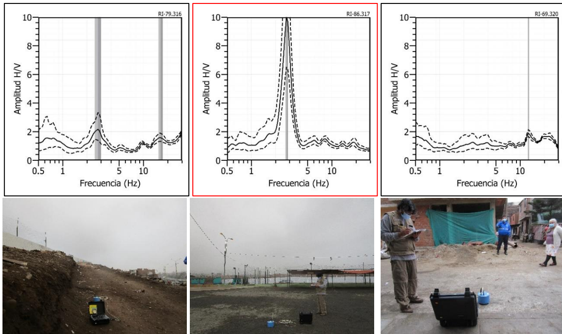
Figura 23. a) Razones espectrales obtenidas para puntos RI-79, RI-86 y RI-69, ubicados de norte a sur en el sector del Complejo Deportivo Villa María (ex botadero "El Montón").
