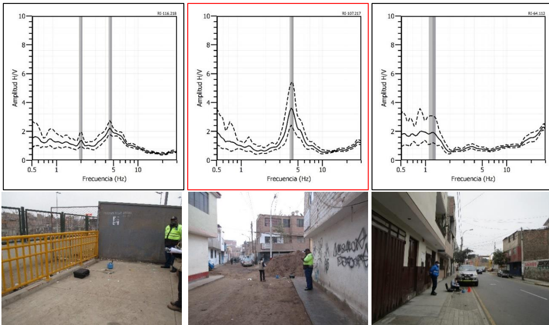
Figura 23. c) Razones espectrales obtenidas para puntos RI-116, RI-107 y RI-64, ubicados de norte a sur en el AA.HH. 1° de Mayo.
