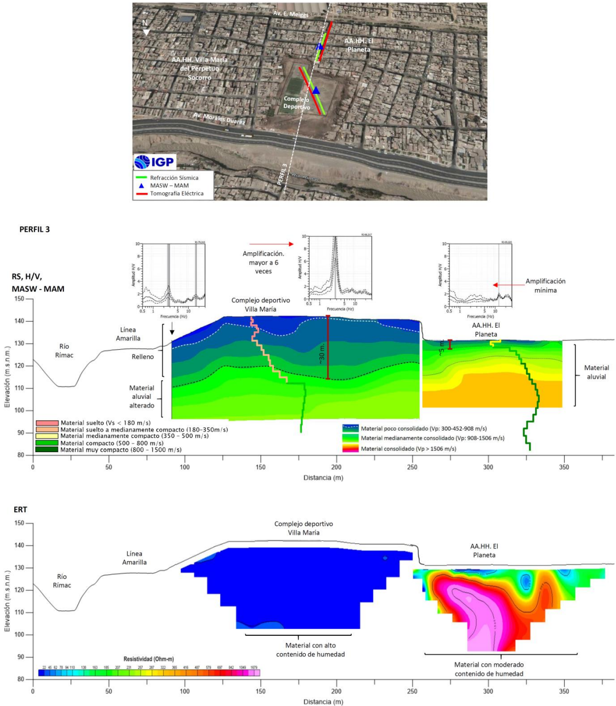
Figura 47. Vista del Perfil-03 y la correlación de los resultados obtenidos con los métodos de H/V, ERT, RS y MASW-MAM para el Sector Central de la MIRR del distrito de Lima Cercado.
