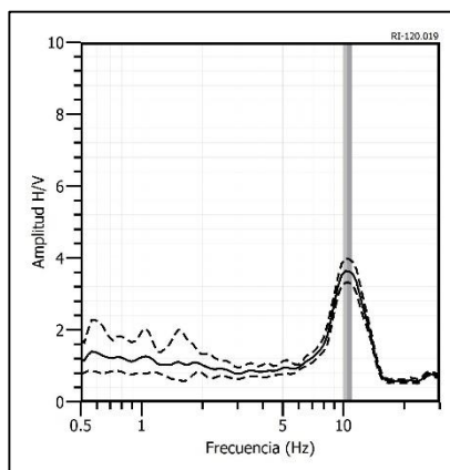
Figura 21b. Ejemplos de razones espectrales (H/V) para los puntos RI-30, RI-107 y RI-120, ubicados en el AA.HH. 1° de Mayo y en Conde de la Vega Alta. Las líneas continuas representan la razón espectral y las discontinuas su desviación estándar. Las barras grises, definen la frecuencia predominante.
