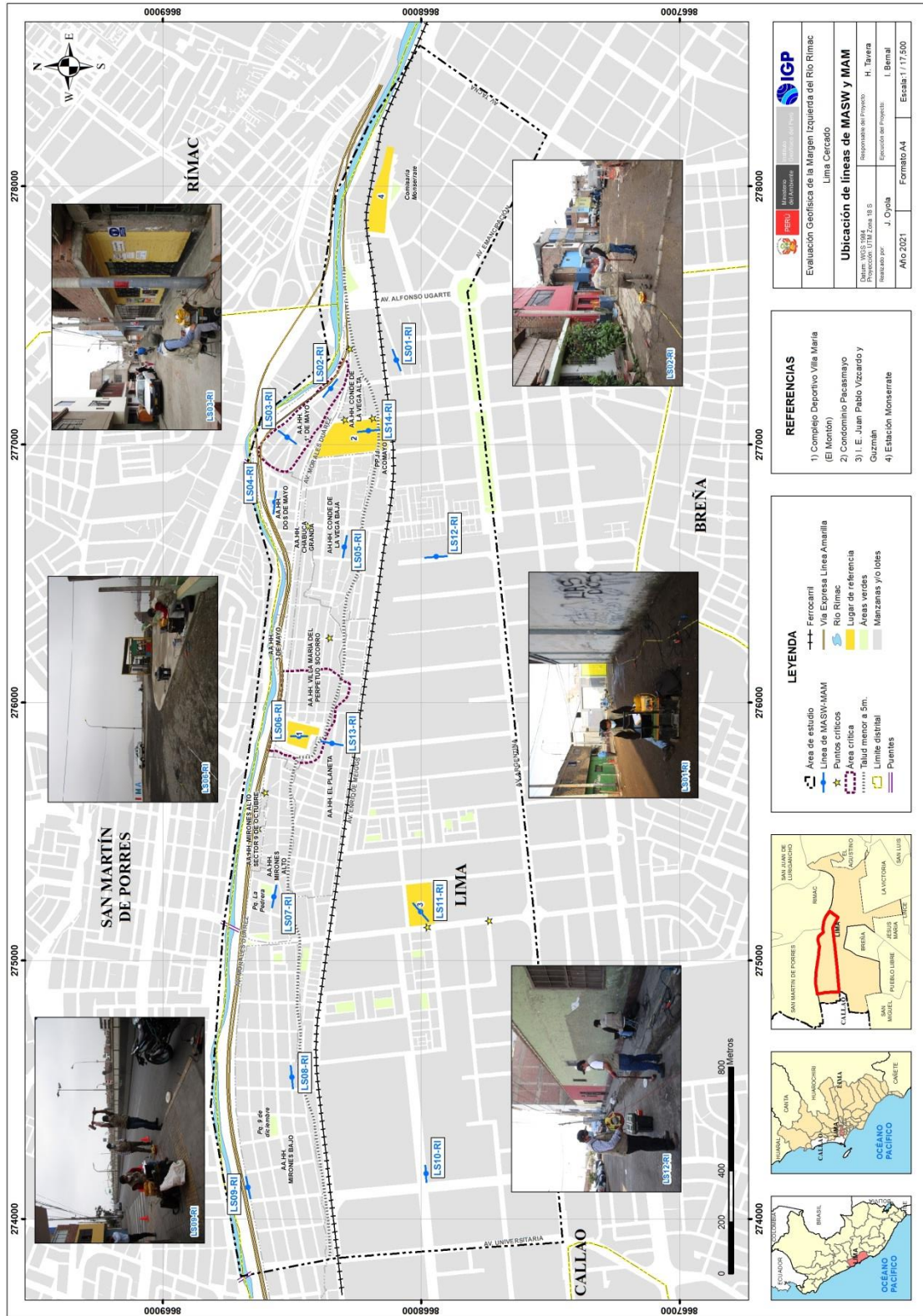
Figura 32. Distribución espacial de las líneas MASW y MAM, codificadas como LS01-RI, ..., LS14-RI.
