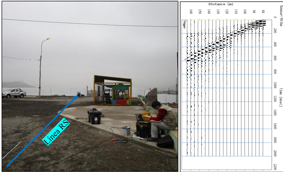
Figura 27. Disposición del equipo de adquisición de datos con la técnica de refracción sísmica (RS03-RI, Complejo deportivo Villa María) y registro sísmico obtenido.
