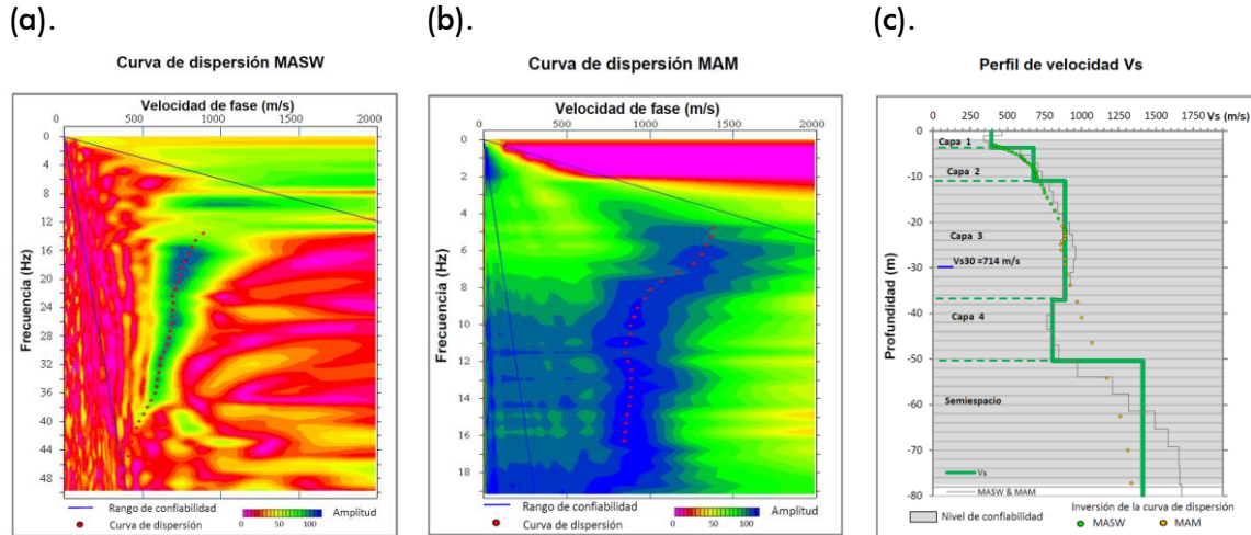
Figura 34. Curvas de dispersión obtenidos a partir de las técnicas MASW (a) y MAM (b) y perfil de velocidad obtenido a partir de la combinación de ambos ensayos (c).
