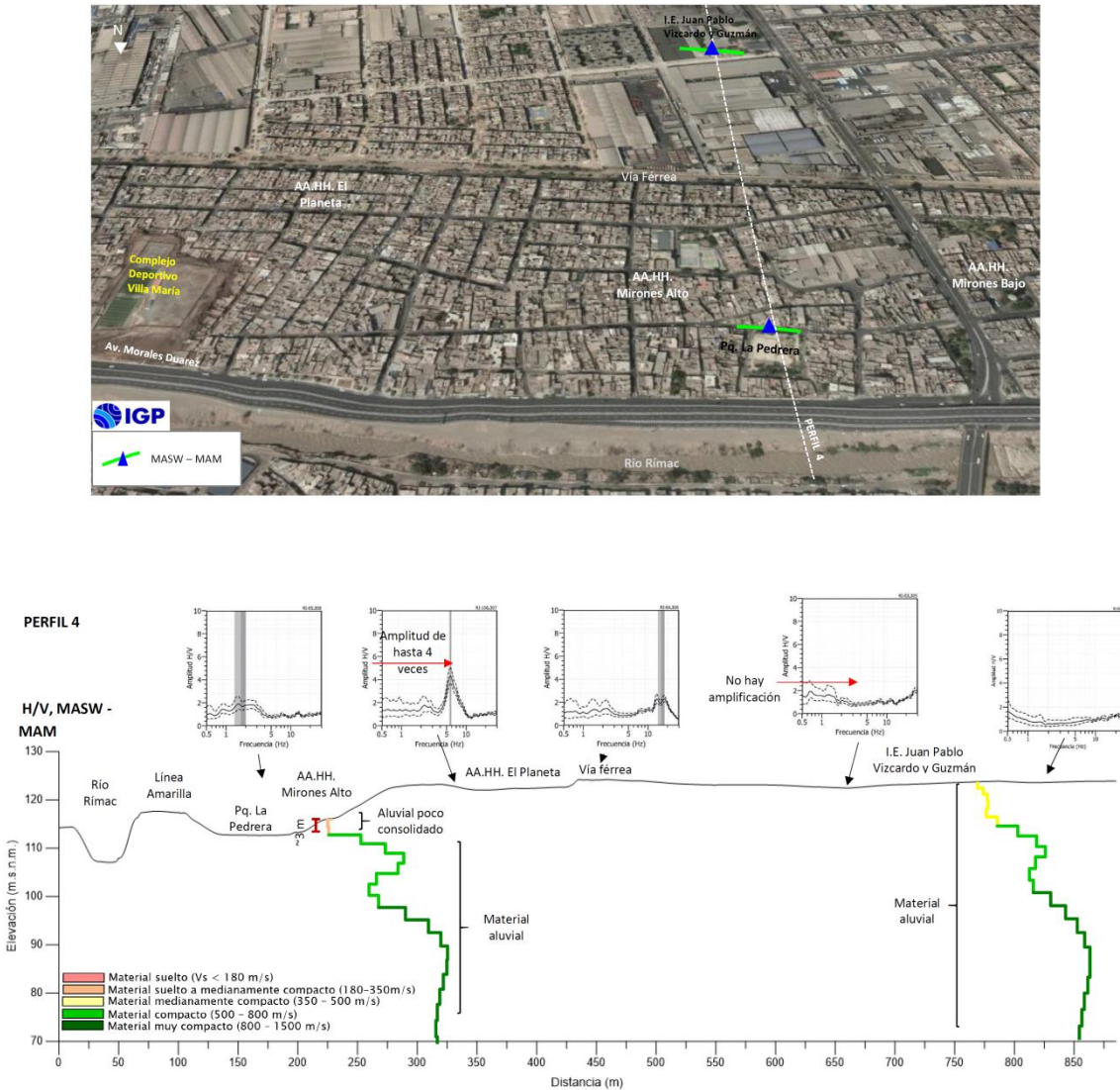
Figura 48. Vista del Perfil-04 y correlación de los resultados obtenidos con los métodos de H/V y MASW-MAM para el extremo Oeste de la MIRR.
