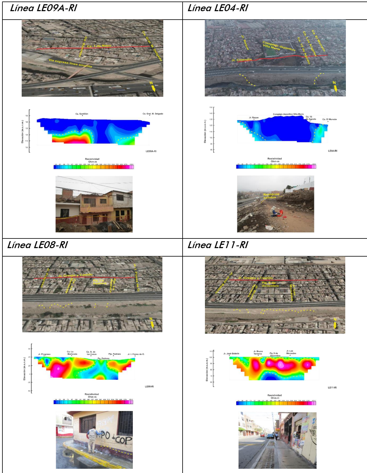
Figura 39. Ubicación y orientación de las líneas de tomografía eléctrica, realizadas en el extremo NE (LE09A-RI), Central (LE04-RI) y NO (LE08-RI, LE11-RI) de la MIRR. Las interlíneas delimitan las zonas con mayor contenido de humedad en cada sección y su proyección.
