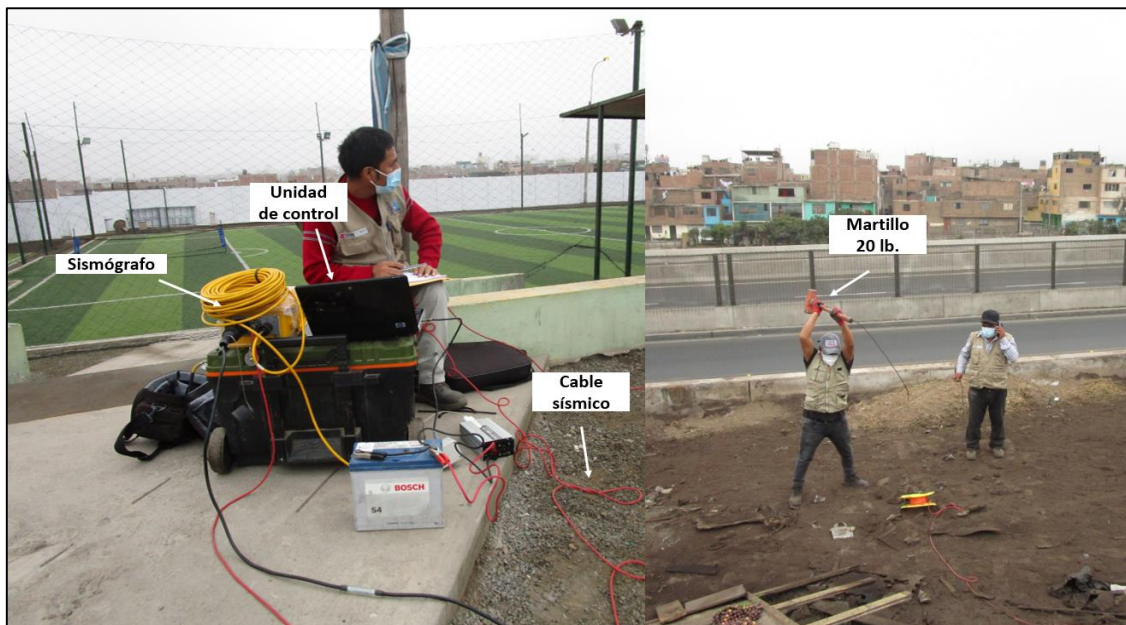
Figura 25. Equipos utilizados en la adquisición de datos RS.
