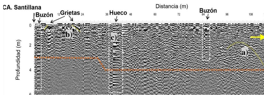
Figura 43. Radargrama, con los diferentes tipos de reflectores asociados a anomalías de tipo hiperbólico (a), lineal (b) y puntuales (c).
