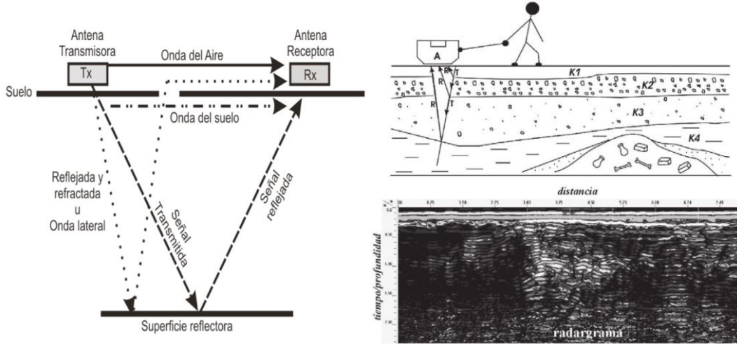
Figura 40. Esquema de la base del método de georadar y de un radargrama (Villela, 2013)
