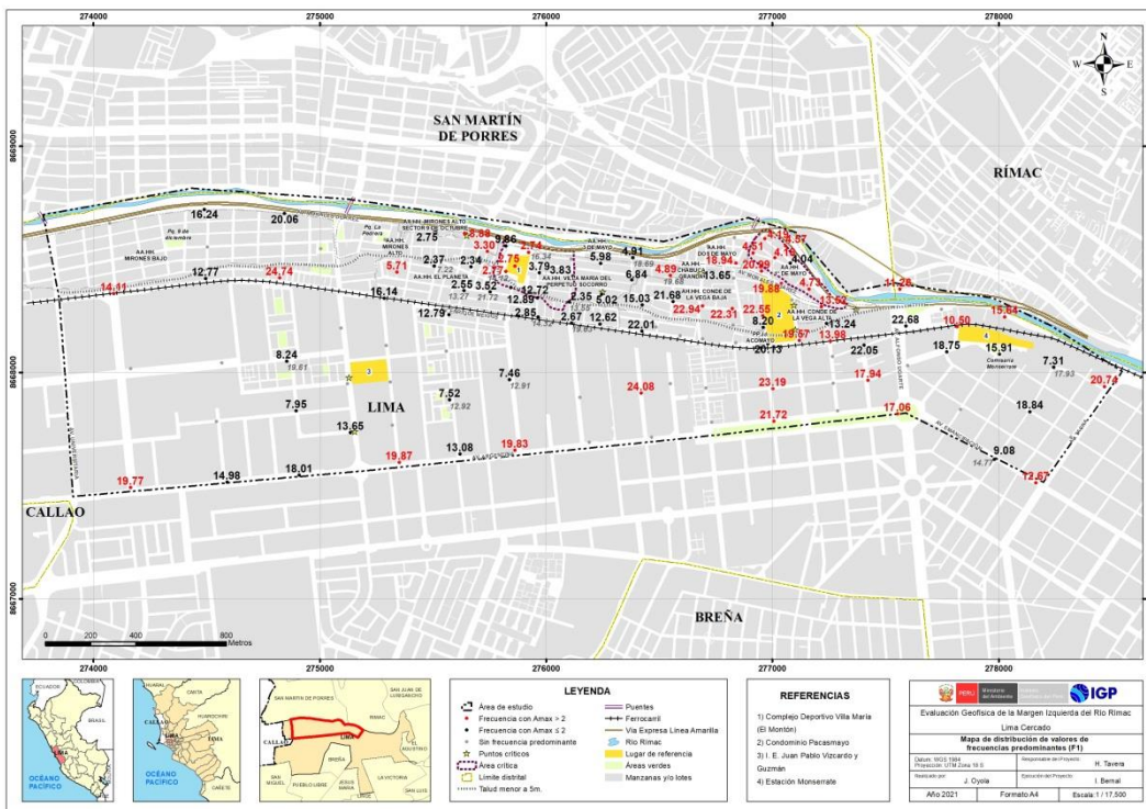
Figura 22. Distribución espacial de las frecuencias F_0 ( F < 2.0 Hz) y F_1 ( F \geq 2.0 Hz). Los valores en rojo, corresponden a puntos con amplificaciones mayores a 2 veces.
