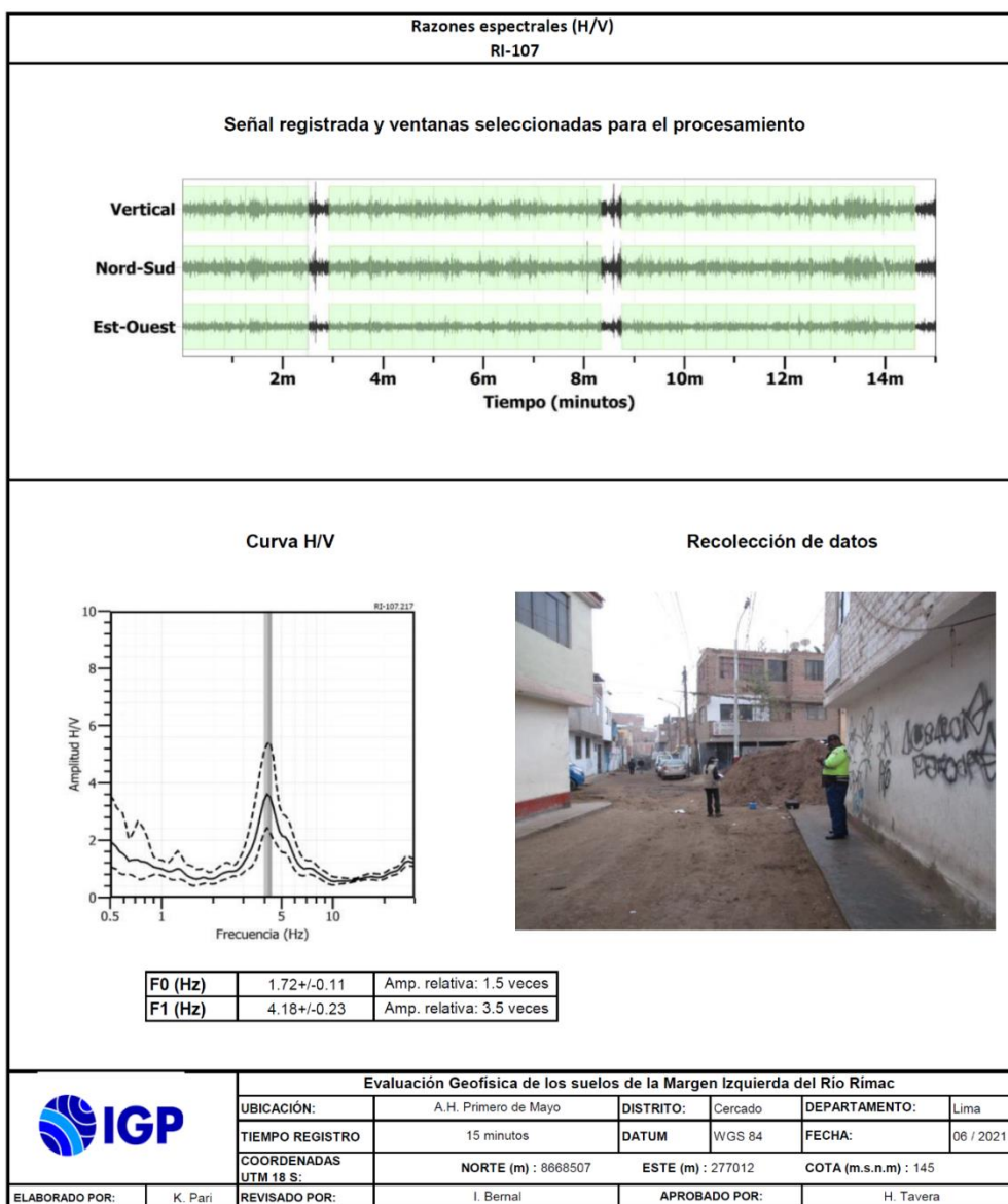
Figura 20. Resultados obtenidos con el método de razones espectrales (H/V) para el punto RI-107. Arriba, la señal registrada y abajo la curva promedio de las razones espectrales (H/V) en línea gruesa y su desviación estándar en líneas discontinuas. Las barras grises, definen la frecuencia predominante.
