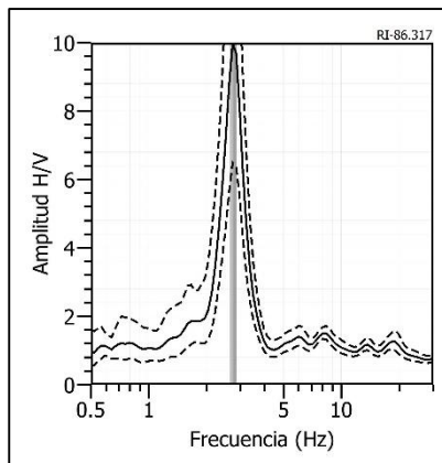
Figura 21a. Ejemplos de razones espectrales (H/V) para los puntos RI-74 (I.E. Juan Pablo Vizcardo – Guzmán) y RI-79 y RI-86 (Complejo Ddeportivo Villa María - ex botadero “El Montón”). Las líneas continuas representan la razón espectral y las discontinuas su desviación estándar. Las barras grises, definen la frecuencia predominante.
