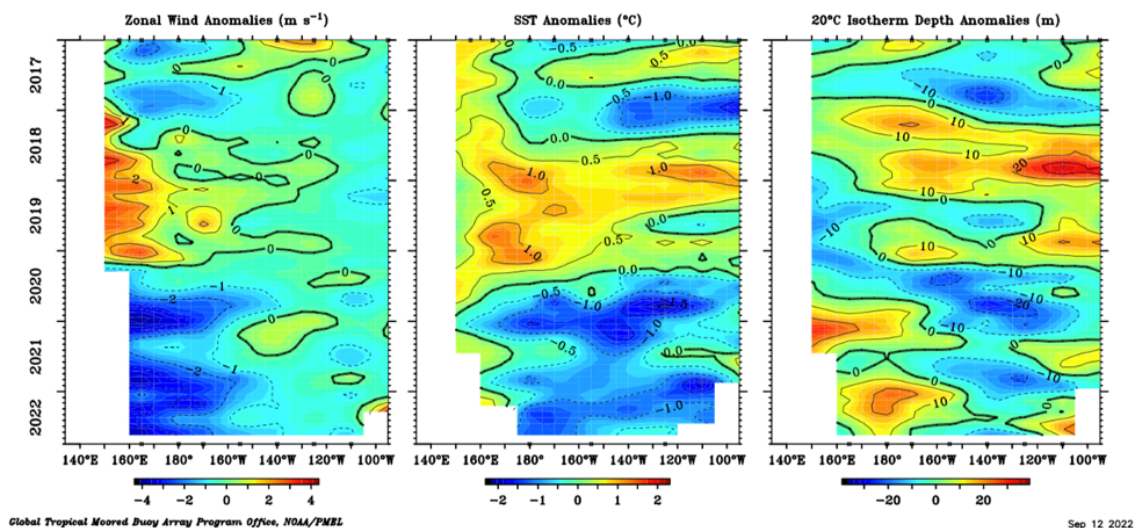
Figura 2. Promedio mensual de la anomalía del viento zonal (a), de la profundidad de la isoterma de 20 ^{\circ}C (b) y de la temperatura superficial del mar (c) a lo largo de la franja ecuatorial del Pacífico (2°S-2°N). Esta imagen se elaboró de otras que se obtienen del proyecto TAO: www.pmel.noaa.gov/tao .
