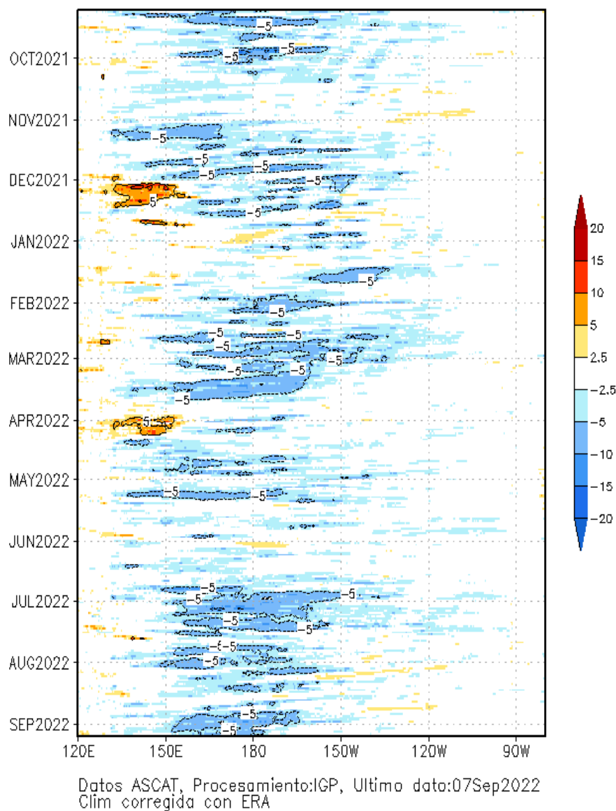
Figura 3. Diagrama longitud-tiempo de las anomalías del esfuerzo de viento zonal ecuatorial que se obtiene de los datos del producto ASCAT hasta el 07 de setiembre de 2022. Elaborado por el IGP.
