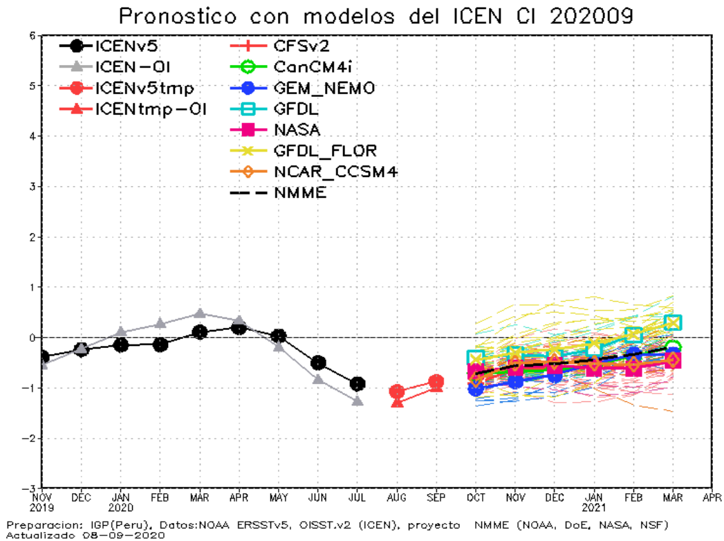
Figura 13. Índice Costero El Niño (ICEN negro con círculos llenos, fuente ERSSTv5; ICEN gris con triángulos, fuente OISSTv2) y sus valores temporales (ICENV5tmp, rojo con círculo lleno, ICENTmp-OI, rojo con triángulos llenos). Además, pronósticos numéricos del ICEN (media móvil de 3 meses de las anomalías pronosticadas de TSM en Niño 1+2) por diferentes modelos climáticos. Los pronósticos de los modelos CFSv2, CanCM4i, GEM_NEMO, GFDL, NASA, GFDL_FLOR y NCAR_CCSM4 tienen como condición inicial el mes de setiembre de 2020. (Fuente: IGP, NOAA, proyecto NMME).
