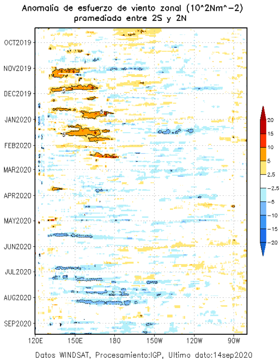
Figura 3. Diagrama longitud-tiempo de las anomalías del esfuerzo de viento zonal ecuatorial basado en datos del producto WINDSAT hasta el 14 de setiembre 2020. Elaboración: IGP.
