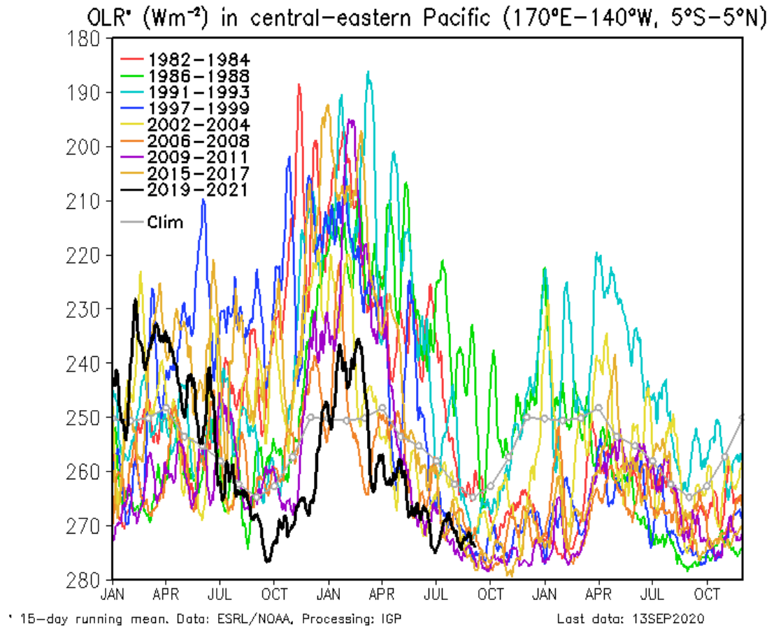
Figura 7. Actividad convectiva en el Pacífico Central Oriental ( 170^{\circ}\text{E}-140^{\circ}\text{W} y 5^{\circ}\text{S}-5^{\circ}\text{N} ) en base a la información de OLR (Outgoing Longwave Radiation). Elaboración IGP
