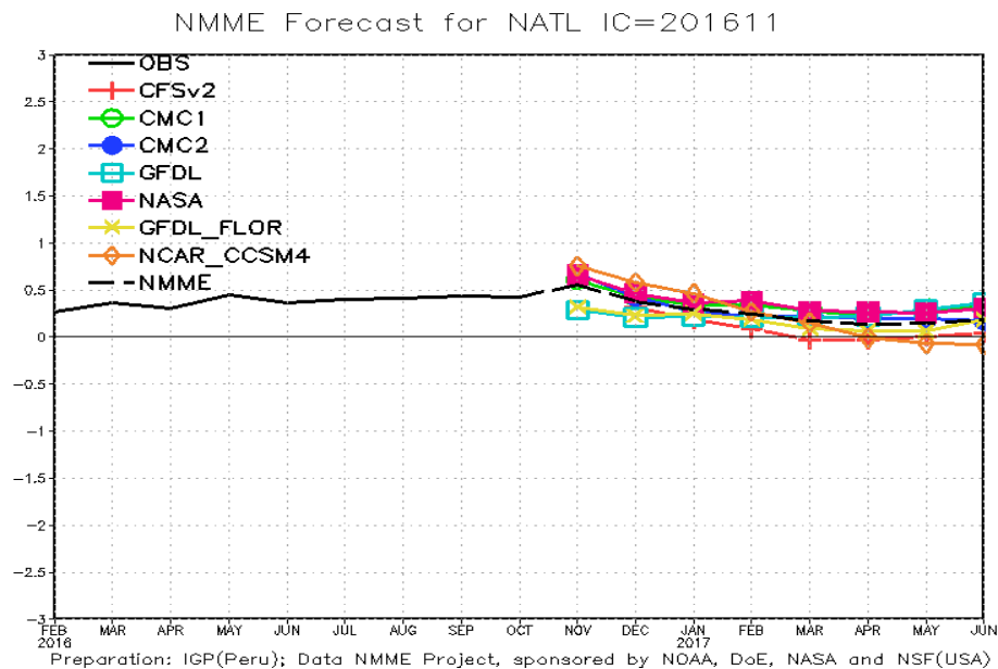
Fig. 9: Pronóstico de las anomalías de temperatura superficial del mar (TSM) para la región del Atlántico tropical Norte (NATL: 5°N-20°N, 30°W-60°W), a partir de condiciones de fines de octubre 2016. Fuente: Instituto Geofísico del Perú (IGP).
