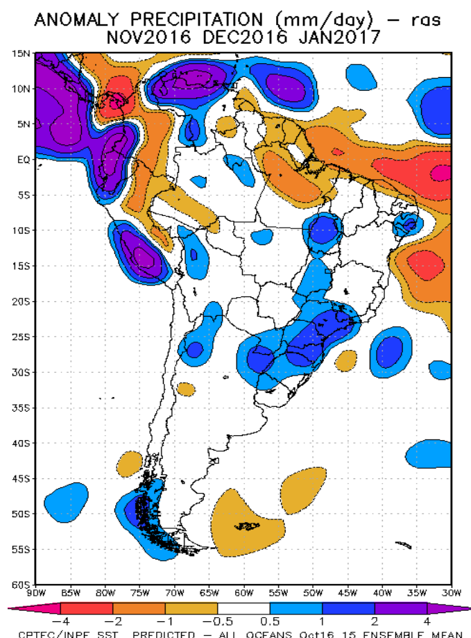
Fig. 10: Pronóstico de las anomalías de la precipitación (mm/día) método ras para el trimestre NDE del 2016-2017 en América del Sur, con datos observados del mes de octubre. Fuente: CPTEC/INPE.
