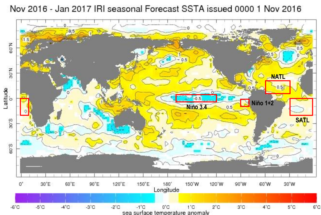
Fig. 7: Pronóstico de las anomalías de temperatura superficial del mar (°C) a nivel global, para el trimestre noviembre-enero (NDE) 2016. Rectángulos rojos indican regiones de análisis. Fuente: International Research Institute for Climate and Society (IRI).
