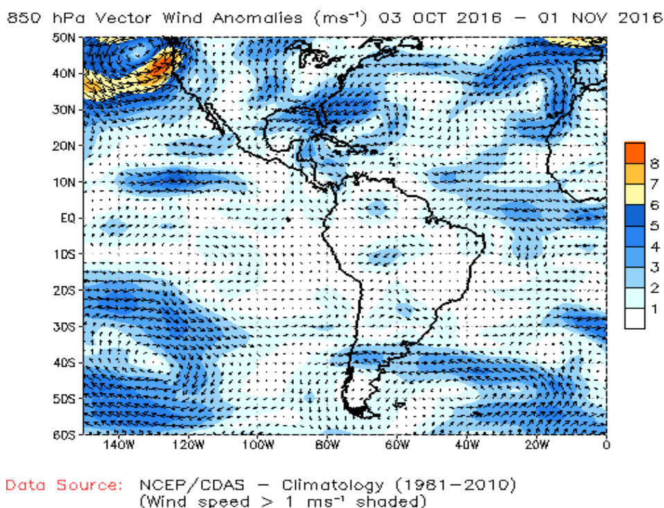
Fig. 2: Anomalia de vientos en niveles bajos (850 hPa) de la atmósfera, (del 03 de octubre al 01 de noviembre de 2016). Las anomalías fueron calculadas utilizando el periodo base los promedios entre 1981 y 2010. Fuente: NOAA/NCEP.
