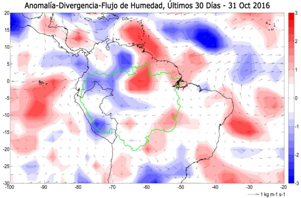
Fig. 3: Anomalías de flujo de humedad integrado en los niveles de 1000 hPa a 300 hPa de la atmósfera y su divergencia. El periodo corresponde de 01 al 30 de setiembre 2016. Las anomalías son calculadas utilizando el periodo base de 1970 a 2015. Se muestra límites de la cuenca Amazónica en línea verde.
