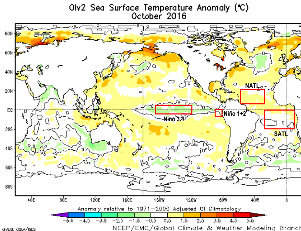
Fig. 1: Anomalías de temperatura superficial del mar (TSM) en °C del mes de octubre de 2016. Las anomalías son calculadas utilizando la climatología del periodo base 1971-2000. Fuente NOAA/NCEP.
