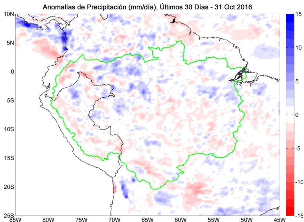
Fig. 4: Anomalías de precipitación estimadas por el TRMM-RT en mm/día hasta 31 de octubre de 2016. Las anomalías fueron calculadas con respecto al periodo base promedio 2000-2015. Se muestra límites de la cuenca Amazónica en línea verde. Las anomalías de precipitación del TRMM-RT actualizadas a tiempo real puede verse en: http://www.igp.gob.pe/eventos-extremos-amazonia-peruana/
