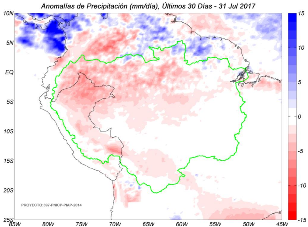
Fig. 4: Anomalías de precipitación estimadas por el TRMM-RT en mm/día hasta 31 de julio de 2017. Las anomalías fueron calculadas con respecto al periodo base promedio 2000-2016. Se muestra los límites de la cuenca Amazónica en líneas de color verde. Las anomalías de precipitación del TRMM-RT actualizadas a tiempo real puede verse en: http://intranet.igp.gob.pe/eventos-extremos-amazonia-peruana/ .
