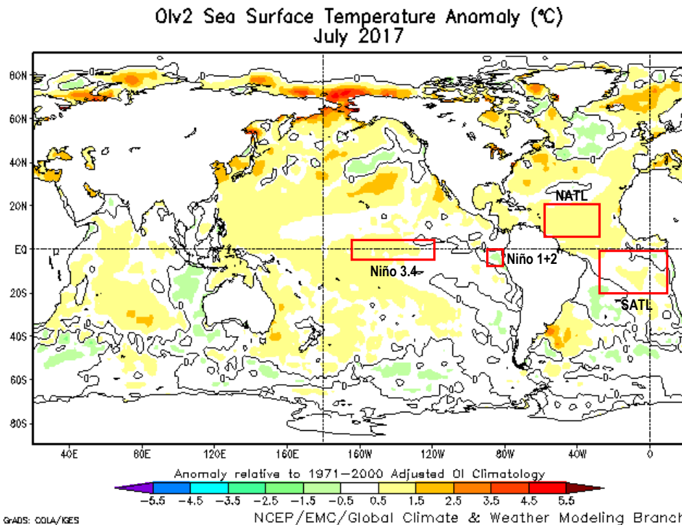
Fig. 1: Anomalías de temperatura superficial del mar (TSM) en °C del mes de julio de 2017. Las anomalías son calculadas utilizando la climatología del periodo base 1971-2000. Fuente NOAA/NCEP.
