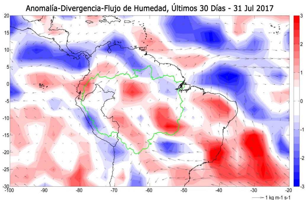
Fig. 3: Anomalías de flujo de humedad integrado en los niveles de 1000 hPa a 300 hPa de la atmósfera y su divergencia. El periodo corresponde de 01 al 31 de julio 2017. Las anomalías son calculadas utilizando el periodo base de 1970 a 2016. Los límites de la cuenca Amazónica se muestran en línea verde.
