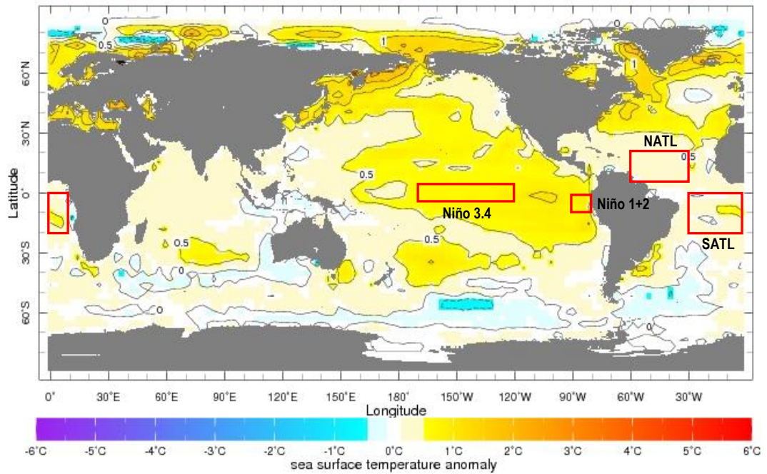
Fig. 7: Pronóstico de las anomalías de TSM (°C) a nivel global, para el trimestre julio-setiembre (ASO) 2017. Rectángulos rojos indican regiones de análisis. Fuente: International Research Institute for Climate and Society (IRI) .
