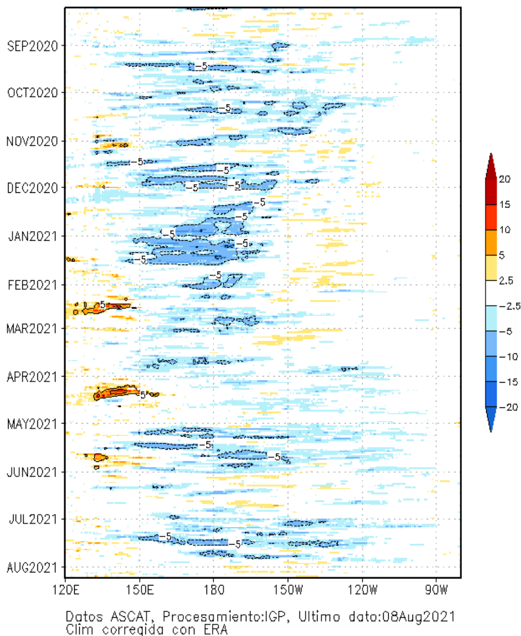
Figura 3. Diagrama longitud-tiempo de las anomalías del esfuerzo de viento zonal ecuatorial que se obtiene de los datos del producto ASCAT hasta el 08 de agosto de 2021. Elaborado por el IGP.
