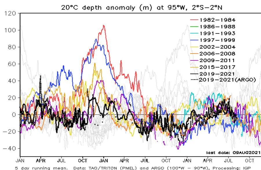
Figura 6. Anomalía de la profundidad de la isoterma de 20 °C (m) en 95°W y promediada entre 2°S y 2°N, con datos de ARGO (línea negra cortada) y TAO (línea negra continua). Elaborado por el IGP.
