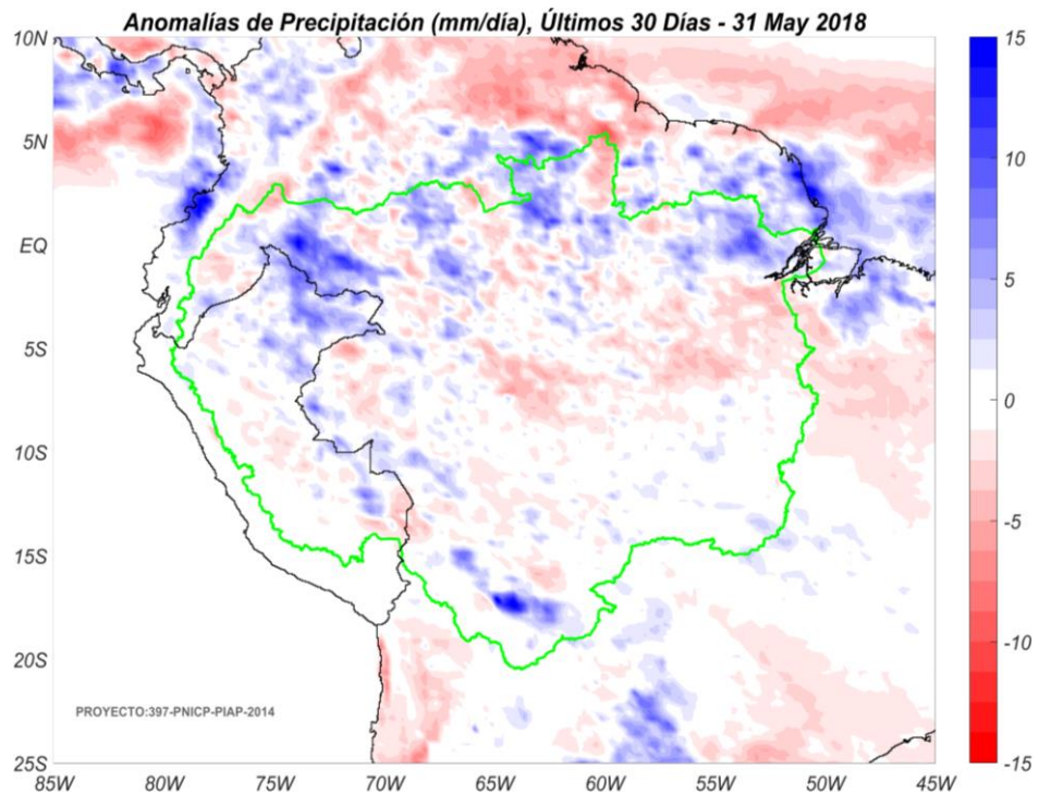
Fig. 4: Anomalías de precipitación estimadas por el TRMM-RT en mm/día hasta 31 de mayo de 2018. Las anomalías fueron calculadas con respecto al periodo base promedio 2000-2017. Se muestra los límites de la cuenca Amazónica en líneas de color verde. Las anomalías de precipitación del TRMM-RT actualizadas a tiempo real puede verse en: http://intranet.igp.gob.pe/eventos-extremos-amazonia-peruana/ .
