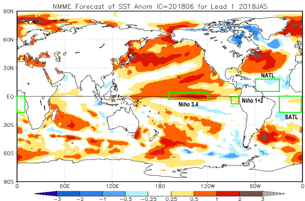
Fig. 7: Pronóstico de las anomalías de TSM (°C) a nivel global, para el trimestre julio-setiembre 2018 (JAS). Rectángulos verdes indican regiones de análisis. Fuente: National Multi-Model Ensemble (NMME) .
