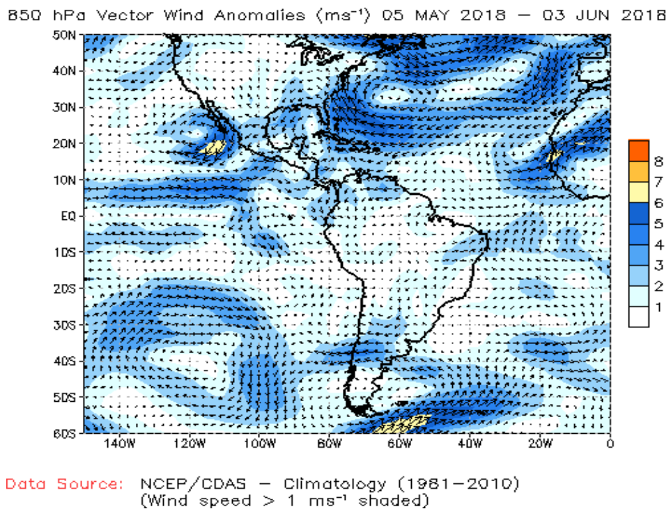
Fig. 2: Vectores de Anomalías de viento en niveles bajos (850 hPa) de la atmósfera, (del 05 mayo al 03 de junio de 2018). Las anomalías fueron calculadas utilizando el periodo base los promedios entre 1981 y 2010. Fuente: NOAA/NCEP.
