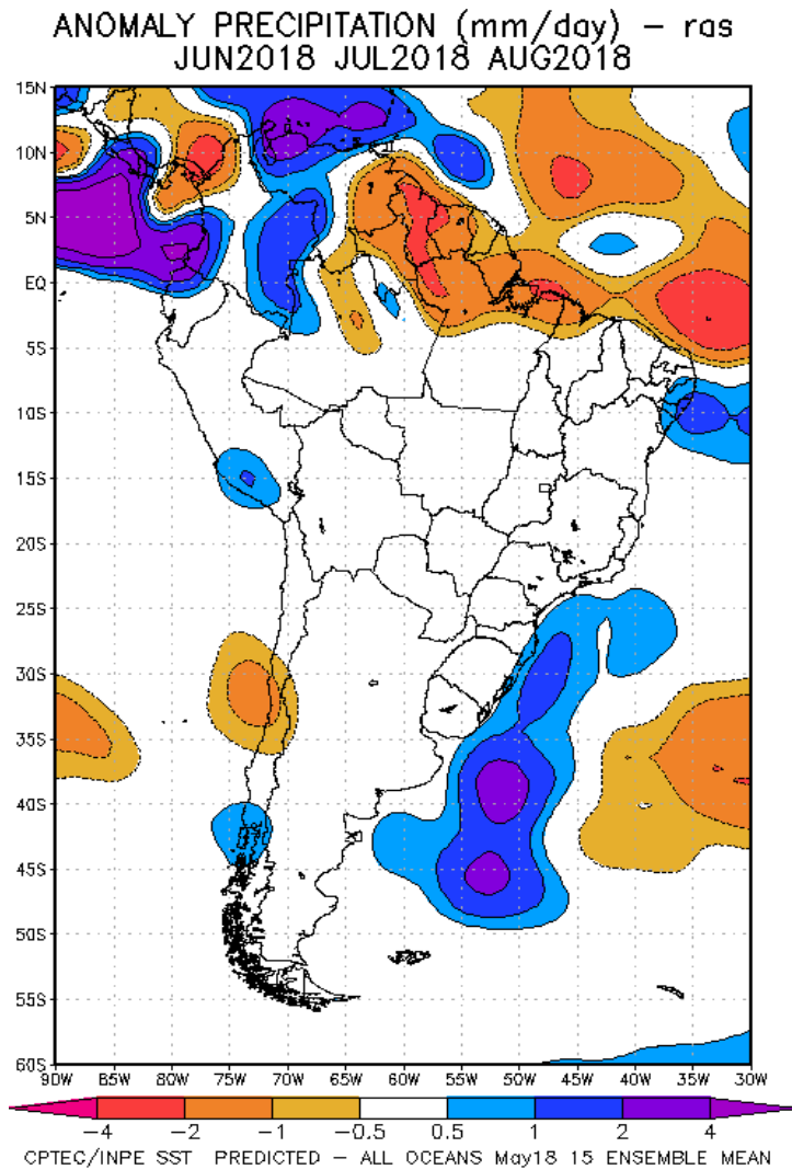
Fig. 10: Pronóstico de las anomalías de la precipitación (mm/día) método ras para el trimestre JJA del 2018 en América del Sur, con datos observados del mes de mayo de 2018. Fuente: CPTEC/INPE.
