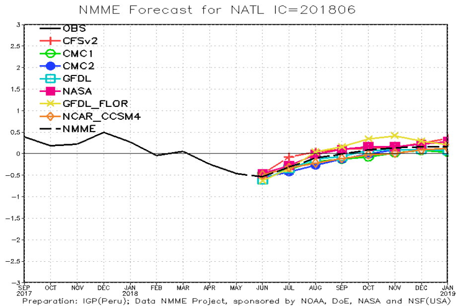
Fig. 9: Pronóstico de las anomalías de temperatura superficial del mar (TSM) para la región del Atlántico tropical Norte (NATL: 5°N-20°N, 30°W-60°W), a partir de condiciones de fines de mayo 2018. Fuente: Instituto Geofísico del Perú (IGP) .
