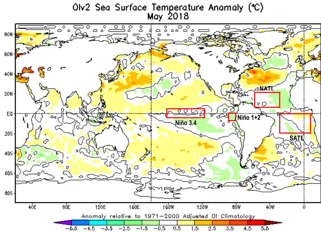
Fig. 1: Anomalías de temperatura superficial del mar (TSM) en °C del mes de mayo de 2018. Las anomalías son calculadas utilizando la climatología del periodo base 1971-2000. Fuente CPTEC/INPE/BRASIL.
