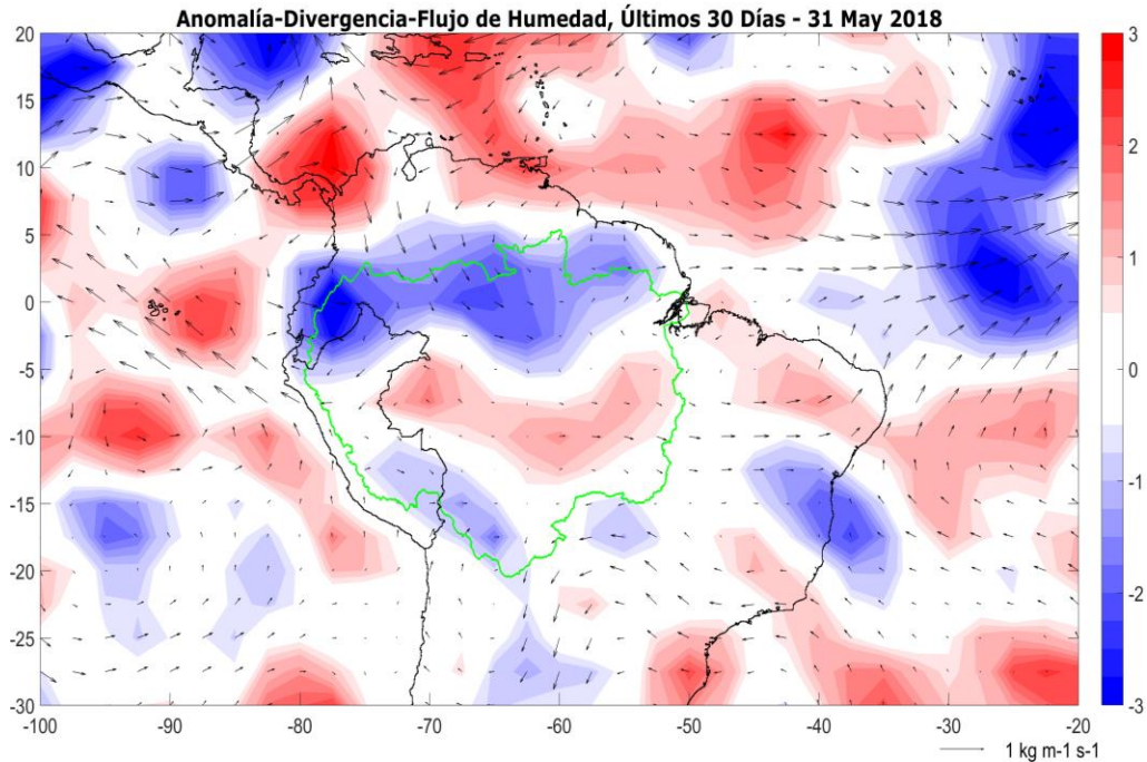
Fig. 3: Anomalías de flujo de humedad integrado en los niveles de 1000 hPa a 300 hPa de la atmósfera (vectores) y su divergencia (colores). El periodo corresponde del 01 hasta el 31 de mayo 2018. Las anomalías son calculadas utilizando el periodo base de 1970 a 2017. Los límites de la cuenca Amazónica se muestran en línea verde.
