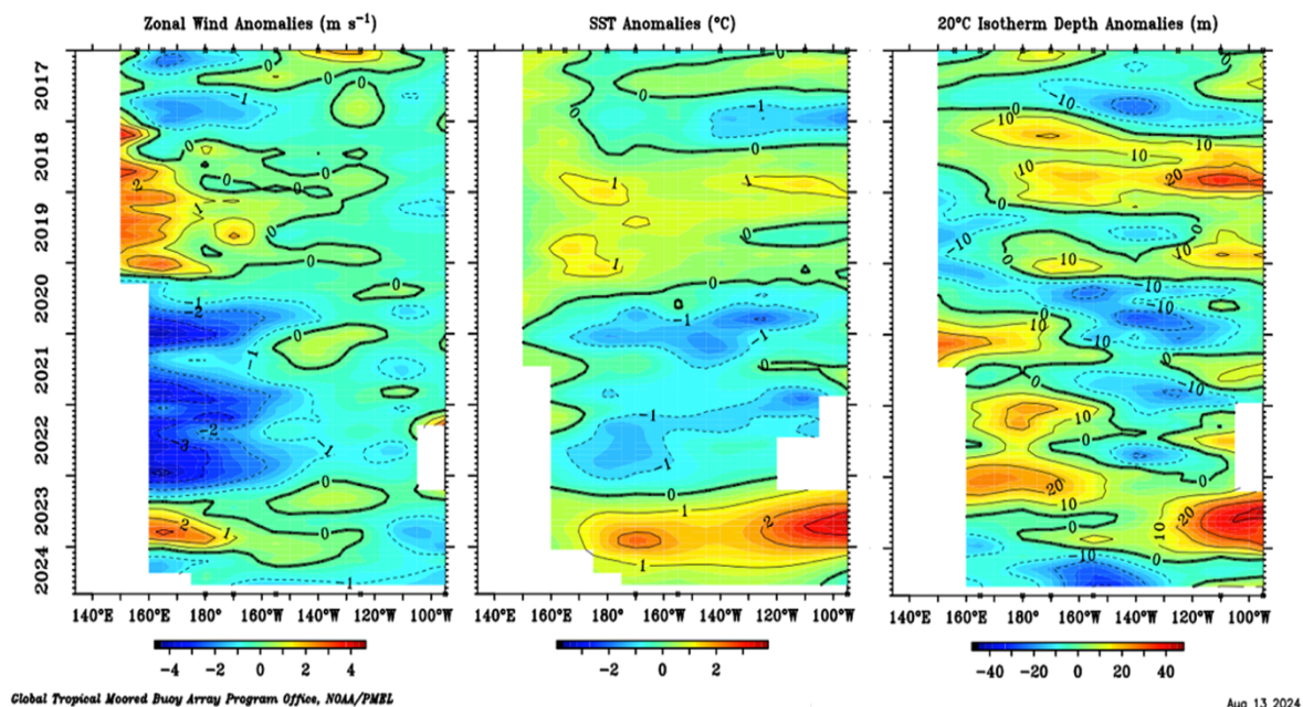
Figura 2. Promedio mensual a lo largo de la franja ecuatorial del Pacífico (2°S-2°N) de las anomalías del viento zonal (panel izquierdo), de la temperatura superficial del mar (panel central) y de la profundidad de la isoterma de 20 °C (panel derecho). Esta imagen se elaboró de otras que se obtienen del proyecto TAO: www.pmel.noaa.gov/
