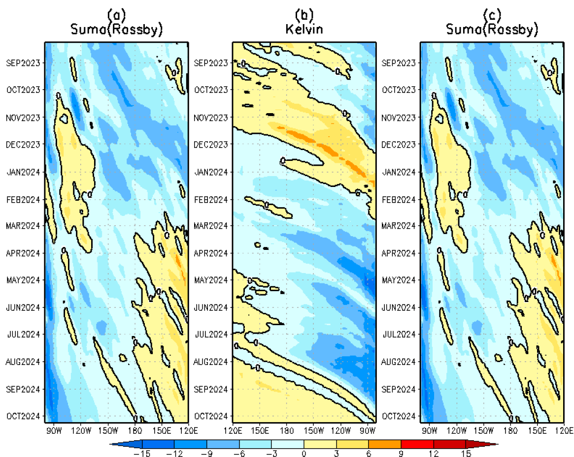
Figura 12. Igual que la Figura 45 pero el modelo tiene una termoclina variable. Fuente: IGP.
