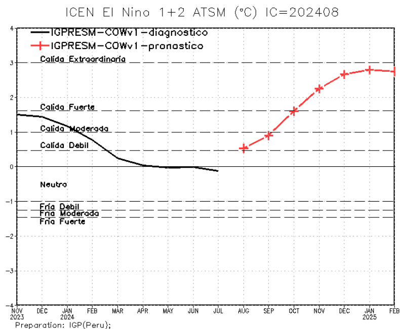
Figura 17. Pronóstico del ICEN de agosto de 2024 a febrero de 2025, generado por el Modelo Regional Earth SystemModel CROCO-OASIS-WRF v.1' (IGP RESM-COW v.1) con condiciones iniciales de agosto.
