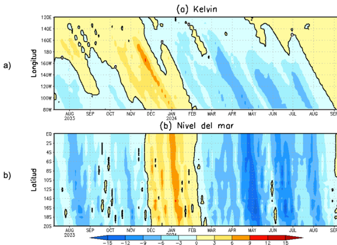
Figura 13. Simulación numérica de la anomalía del nivel del mar (cm) a lo largo de la franja ecuatorial del océano Pacífico (panel superior) y a lo largo de la costa peruana (panel inferior). Esta simulación se realizó con el modelo oceánico lineal (LOM) forzado con esfuerzo de viento del reanalysis de NCEP. La línea verde entrecortada indica el inicio de la simulación del pronóstico con esfuerzo de viento igual a cero. Elaborado por el IGP.
