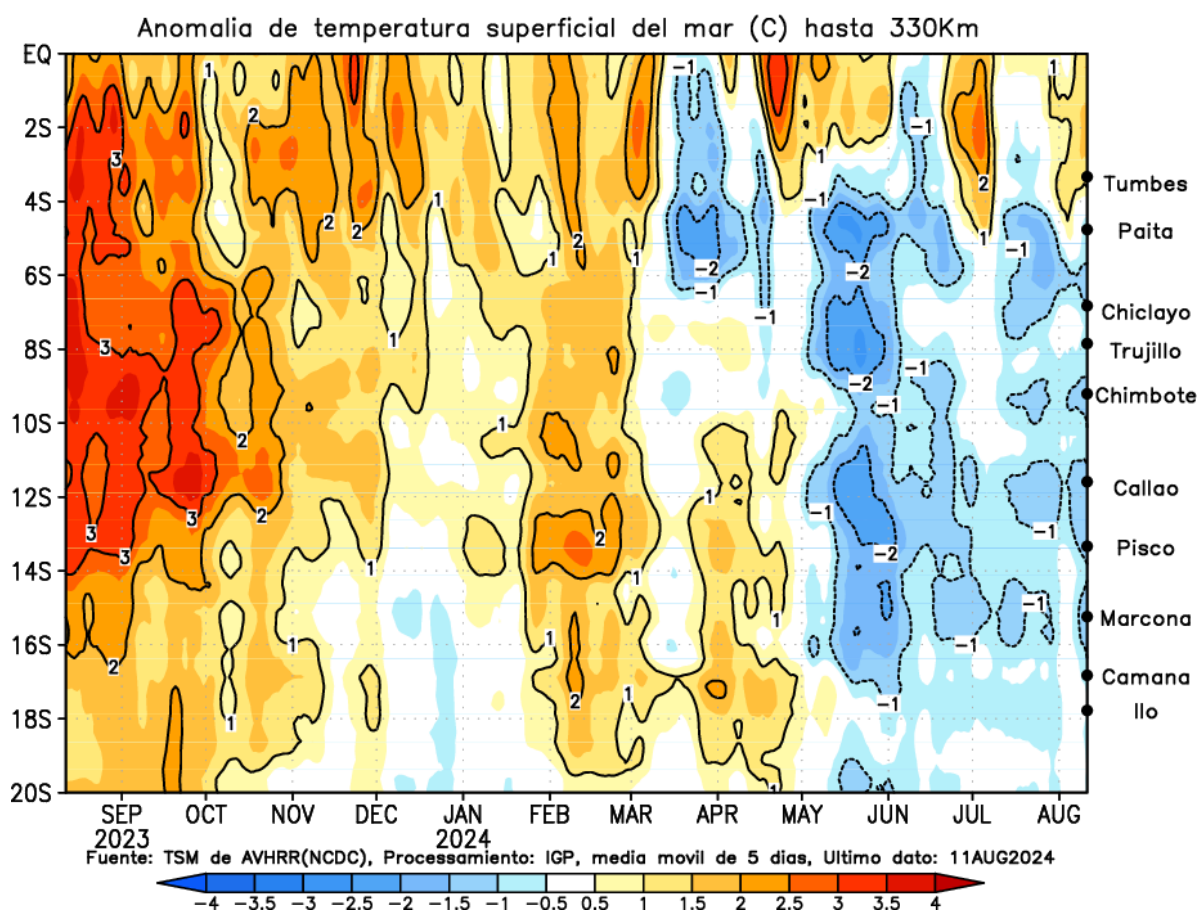
Figura 9. Anomalia de la TSM dentro de los 300 km de la costa peruana. Elaborado por el IGP.
