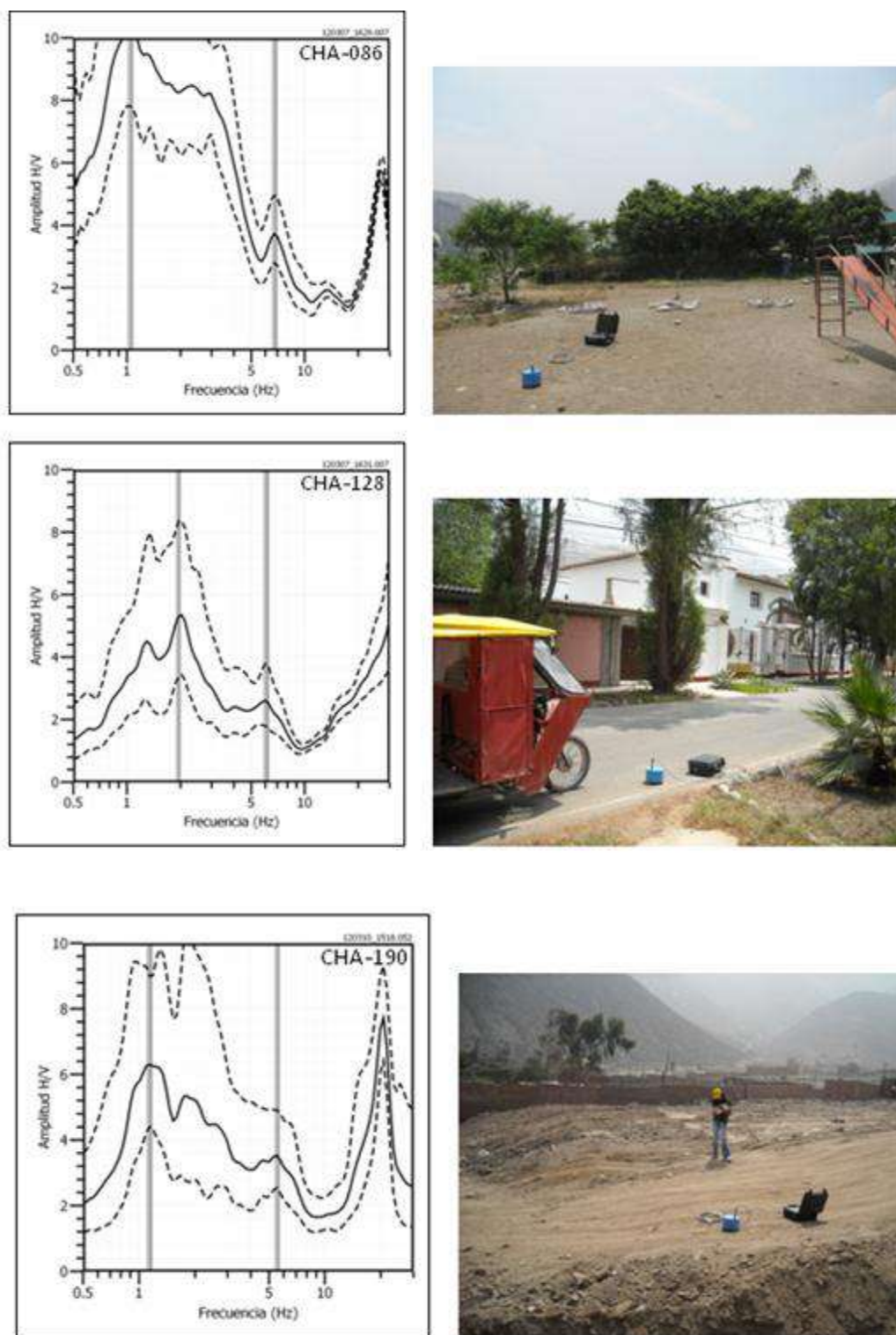
Figura 40: //Continuación... Ejemplos de razones espectrales obtenidas para los puntos CHA-086, CHA-128 y CHA-190 ubicados sobre el Área A2 (Figura 39).
