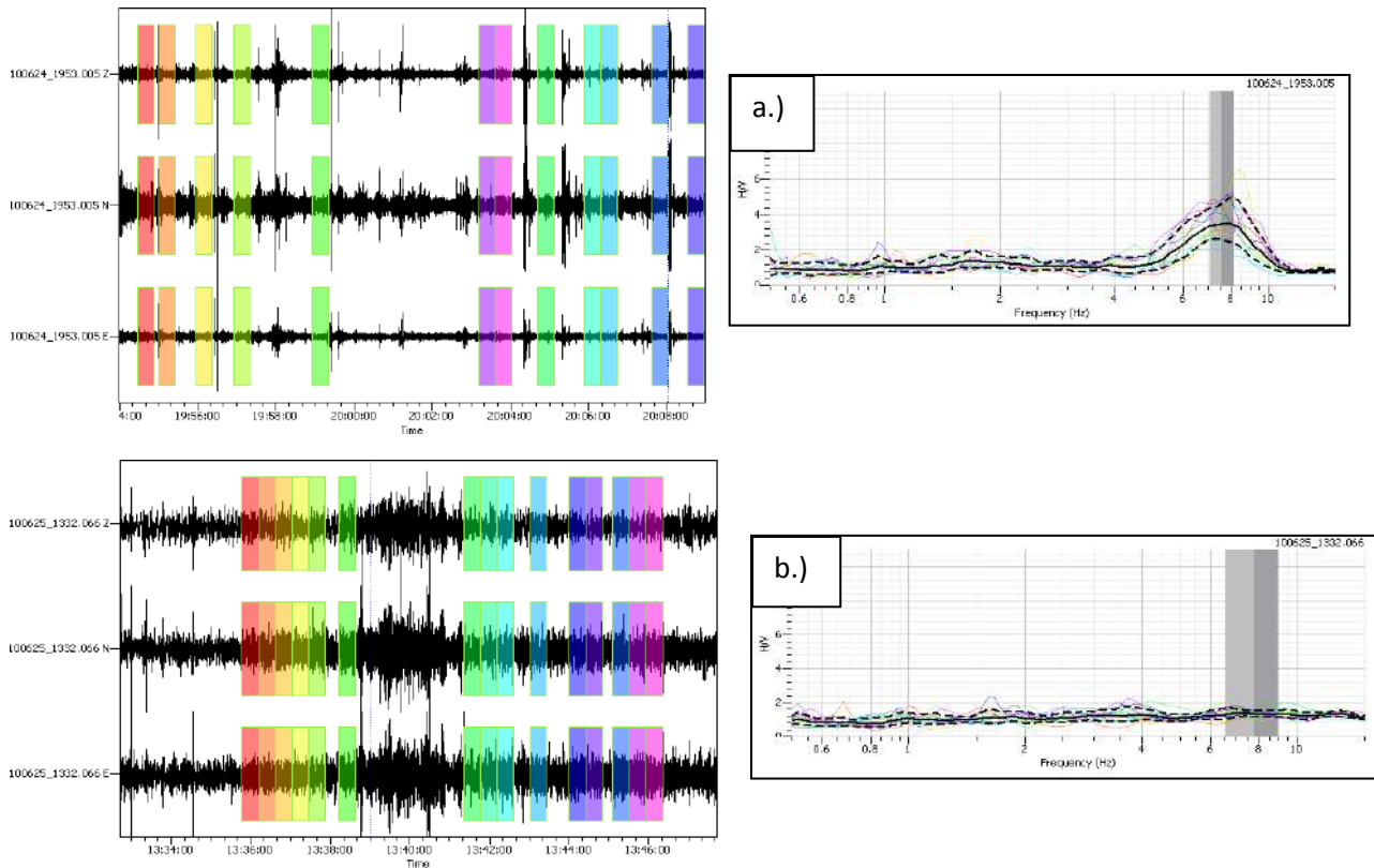
Figura 6: Ejemplo de selección de ventanas de registro de vibración ambiental (rectángulos de colores) en sus tres componentes y con sus respectivos gráficos de razones espectrales H/V. a.) Registros y razones H/V donde se identifican frecuencias predominantes, b.) Registros en los cuales no resalta ninguna frecuencia predominante. Las líneas gruesas en los gráficos H/V indican el promedio de las curvas de razones espectrales y las líneas discontinuas su desviación estándar.
