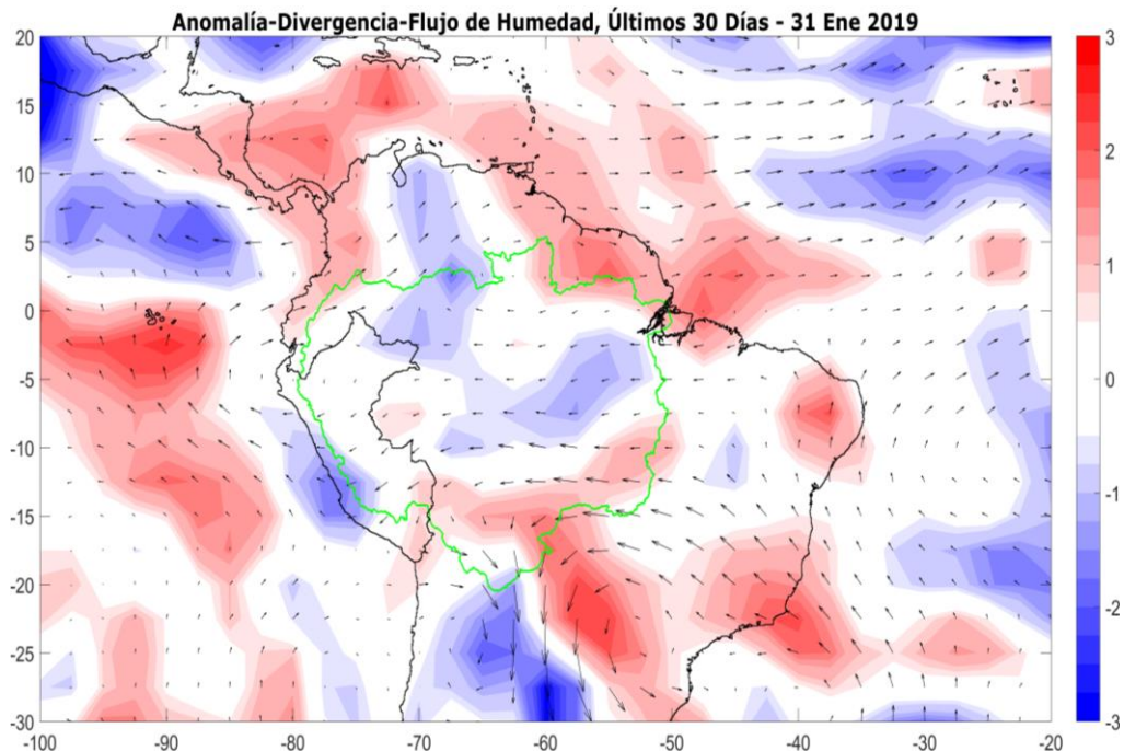
Fig. 3: Anomalías de flujo de humedad integrado en los niveles de 1000 hPa a 300 hPa de la atmósfera (vectores) y su divergencia (colores). El periodo corresponde del 01 hasta el 31 de enero 2019. Las anomalías son calculadas utilizando el periodo base de 1979 a 1995. Los límites de la cuenca Amazónica se muestran en línea verde.
