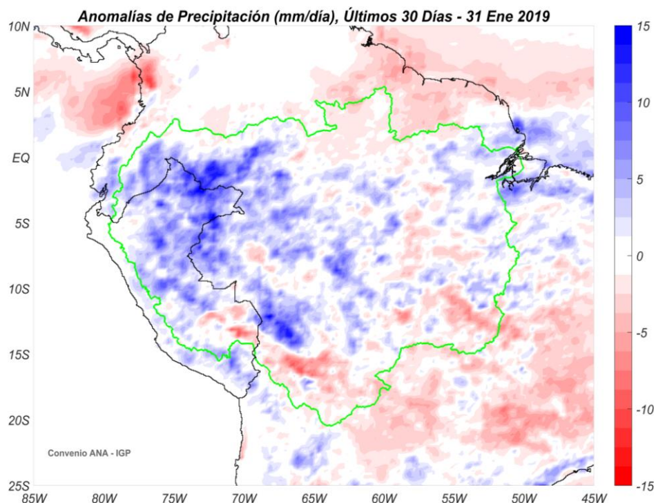
Fig. 4: Anomalías de precipitación estimadas por el TRMM-RT en mm/día hasta 31 de enero de 2019. Las anomalías fueron calculadas con respecto al periodo base promedio 2000-2017. Se muestra los límites de la cuenca Amazónica en líneas de color verde. Las anomalías de precipitación del TRMM-RT actualizadas a tiempo real puede verse en: http://intranet.igp.gob.pe/eventos-extremos-amazonia-peruana/ .
