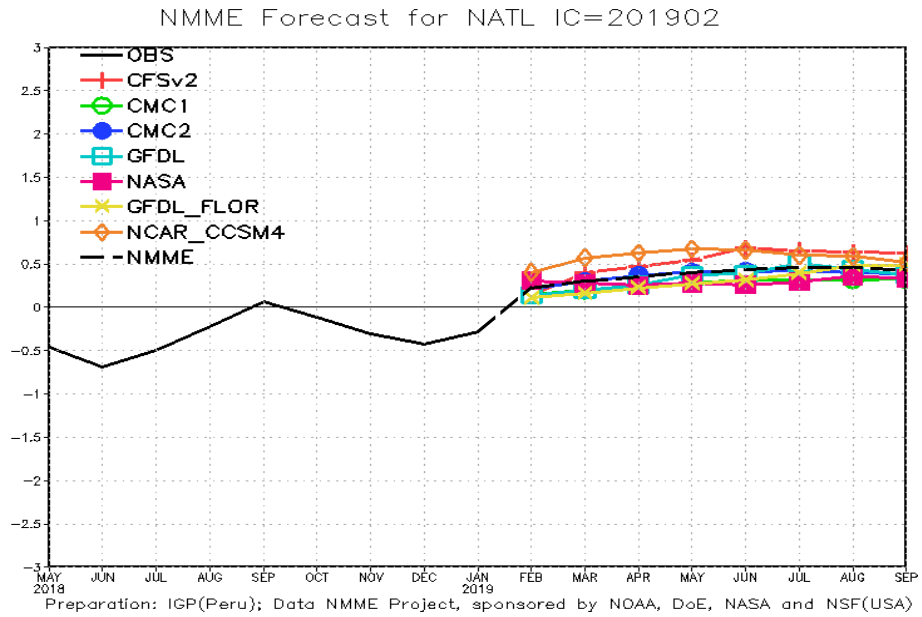
Fig. 9: Pronóstico de las anomalías de temperatura superficial del mar (TSM) para la región del Atlántico tropical Norte (NATL: 5°N-20°N, 30°W-60°W), a partir de condiciones de fines de enero 2019. Fuente: Instituto Geofísico del Perú (IGP) .
