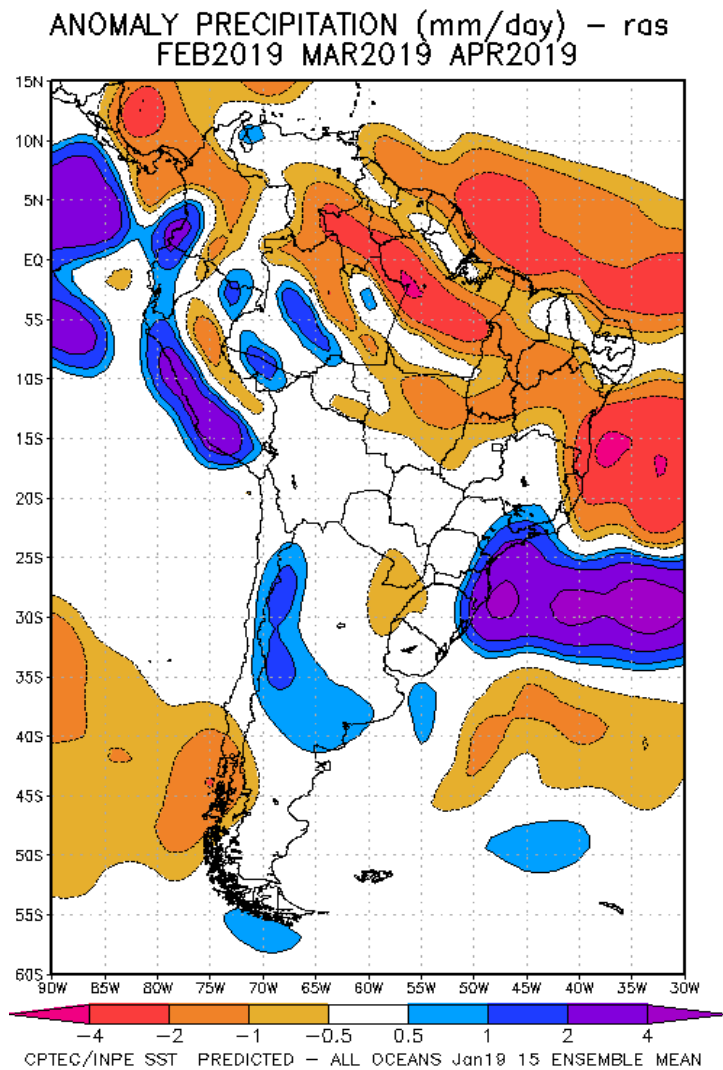
Fig. 10: Pronóstico de las anomalías de la precipitación (mm/día) método ras para el trimestre FMA del 2019 en América del Sur, con datos observados de fines del mes de enero de 2019. Fuente: CPTEC/INPE.
