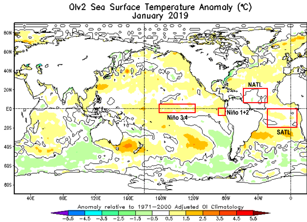
Fig. 1: Anomalías de temperatura superficial del mar (TSM) en °C del mes de enero de 2019. Las anomalías son calculadas utilizando la climatología del periodo base 1971-2000. Fuente CPTEC/INPE/BRASIL.
