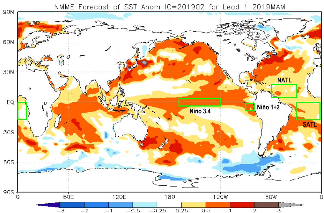
Fig. 7: Pronóstico de las anomalías de TSM (°C) a nivel global, para el trimestre marzo-abril-mayo 2019 (MAM). Rectángulos verdes indican regiones de análisis. Fuente: National Multi-Model Ensemble (NMME) .
