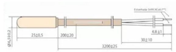
Figura 2. Sensor de temperatura SB70.
