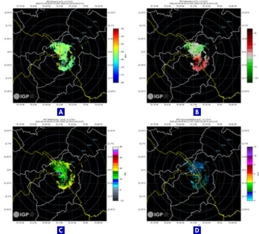
Figura 7. Gráfico meteorológico generado por el método Spectra: (a) potencia, (b) velocidad Dopper, (c) reflectividad, (d) ancho espectral.
