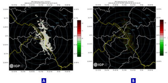
Figura 5. (a) Gráfico meteorológico de velocidad Doopler generado por el método Pulse Pair. (b) Gráfico meteorológico de velocidad Doopler generado por el método Spectra.
