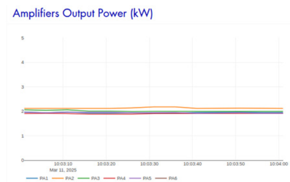
Figura 2. Gráfica de la potencia incidente de un módulo. Cada línea corresponde a un amplificador.
