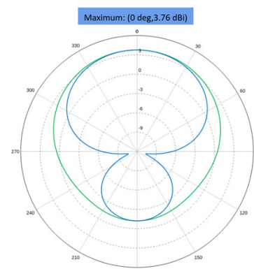
Figura 1. Patrón de radiación de antena QHA de 400 MHz con las dimensiones iniciales.
