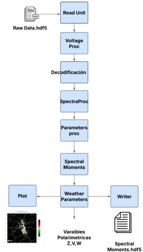
Figura 2. Diagrama de bloques de Signal Chain utilizando el método Spectra.
