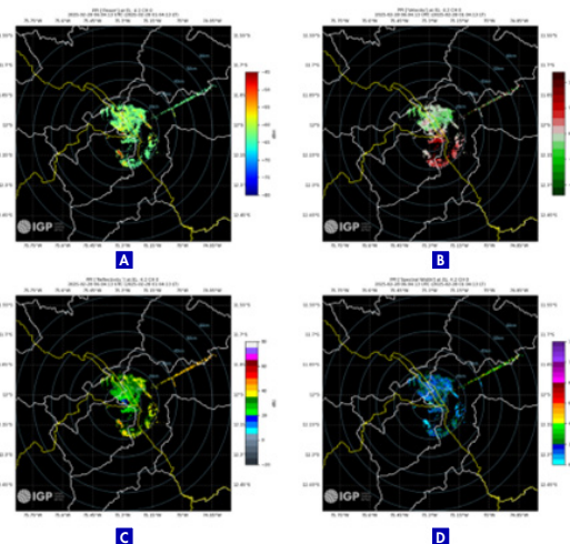
Figura 6. Gráfico meteorológico generado por el método Pulse Pair: (a) potencia, (b) velocidad Doopler, (c) reflectividad, (d) ancho espectral.
