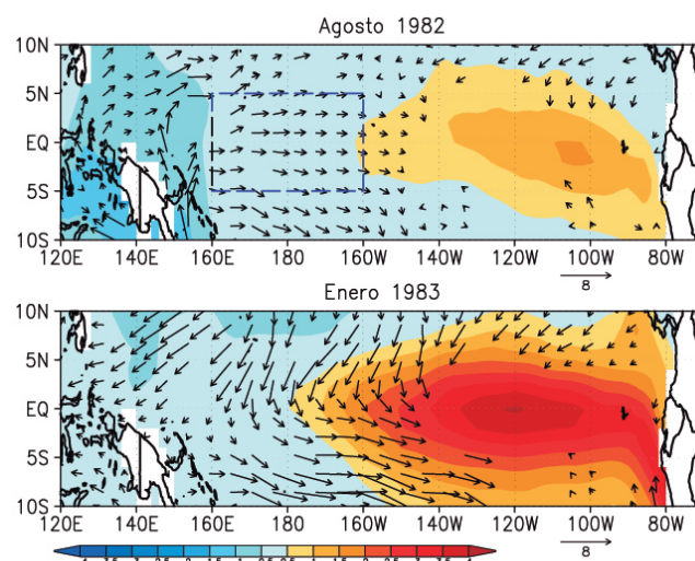
Figura 2. Anomalías de la temperatura superficial del mar (colores; °C; datos: ERSST) y esfuerzo de viento (10-2 Nm-2; datos: NCEP/NCAR Reanalysis) en agosto 1982 (arriba) y enero 1983 (abajo). El recuadro indica la región para el índice en las Figuras 3 y 4.
