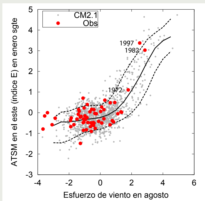
Figura 3. Anomalías observadas (rojo) del esfuerzo de viento del oeste en 160^{\circ}\text{E} - 160^{\circ}\text{W} , 5^{\circ}\text{S} - 5^{\circ}\text{N} en agosto (datos: WASWind) vs el índice E de anomalía de temperatura superficial del mar en el Pacífico ecuatorial oriental en el enero siguiente (datos: HadISST). En gris se muestran 1200 años de datos sintéticos de simulaciones con el modelo GFDL CM2.1 (los percentiles de 10, 50 y 90 % se indican en negro), los cuales le dan más credibilidad al análisis observacional basado en una pequeña muestra. Adaptado de Takahashi y Dewitte, 2014.
