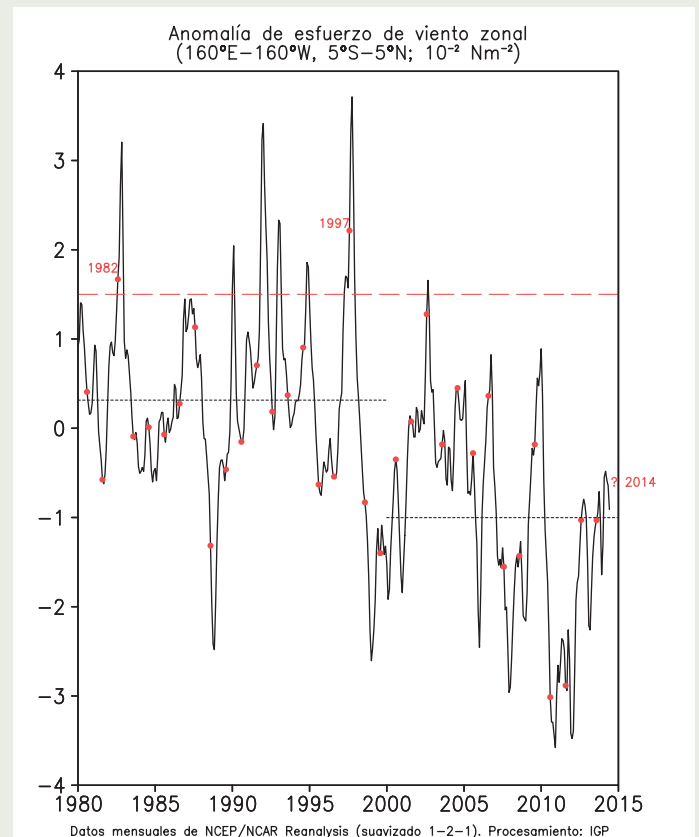
Figura 4. Anomalías mensuales del esfuerzo de viento del oeste en 160^{\circ}\text{E} - 160^{\circ}\text{W} , 5^{\circ}\text{S} - 5^{\circ}\text{N} (datos: NCEP/NCAR Reanalysis, con suavizado 1-2-1). Los valores de agosto se indican en rojo. Los promedios de 1980-1999 y 2000-2013 se muestran punteados. El valor umbral, ajustado para esta fuente de datos, se indica con la línea discontinua.
