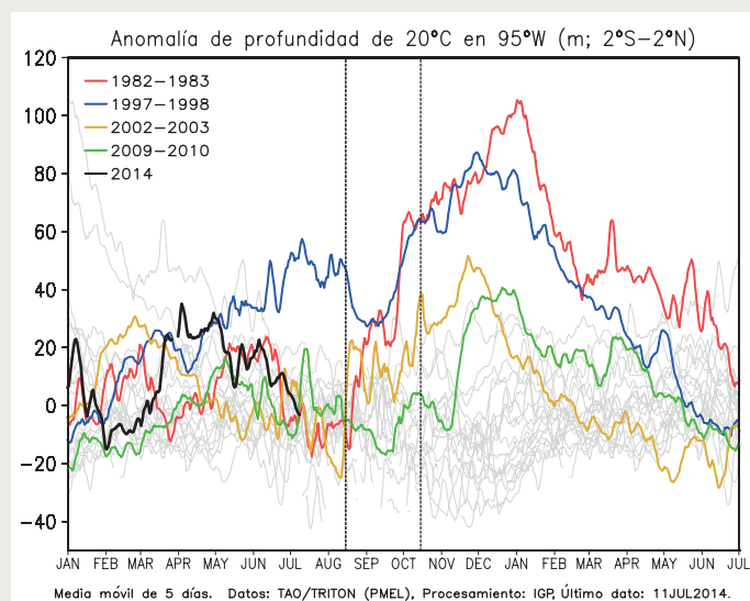
Figura 1. Anomalía de la profundidad (metros) de la isoterma de 20 °C (proxy de la termoclina) calculada de boyas oceanográficas en 95°W (promedio entre 2°S y 2°N, con media móvil de 5 días). Algunos eventos El Niño selectos se indican con colores y los datos del 2014 están en negro. Datos: TAO/TRITON (PMEL).
