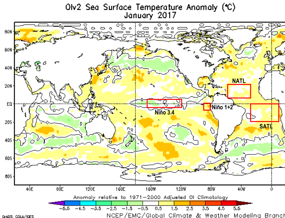
Fig. 1: Anomalías de temperatura superficial del mar (TSM) en °C del mes de enero de 2017. Las anomalías son calculadas utilizando la climatología del periodo base 1971-2000. Fuente NOAA/NCEP.
