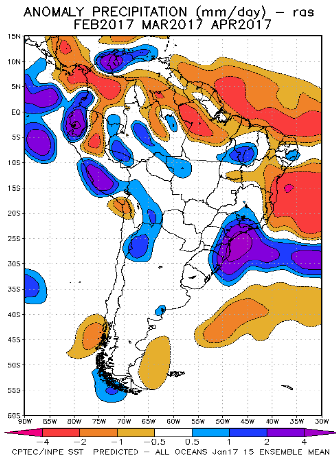
Fig. 10: Pronóstico de las anomalías de la precipitación (mm/día) método ras para el trimestre FMA del 2017 en América del Sur, con datos observados del mes de enero. Fuente: CPTEC/INPE.
