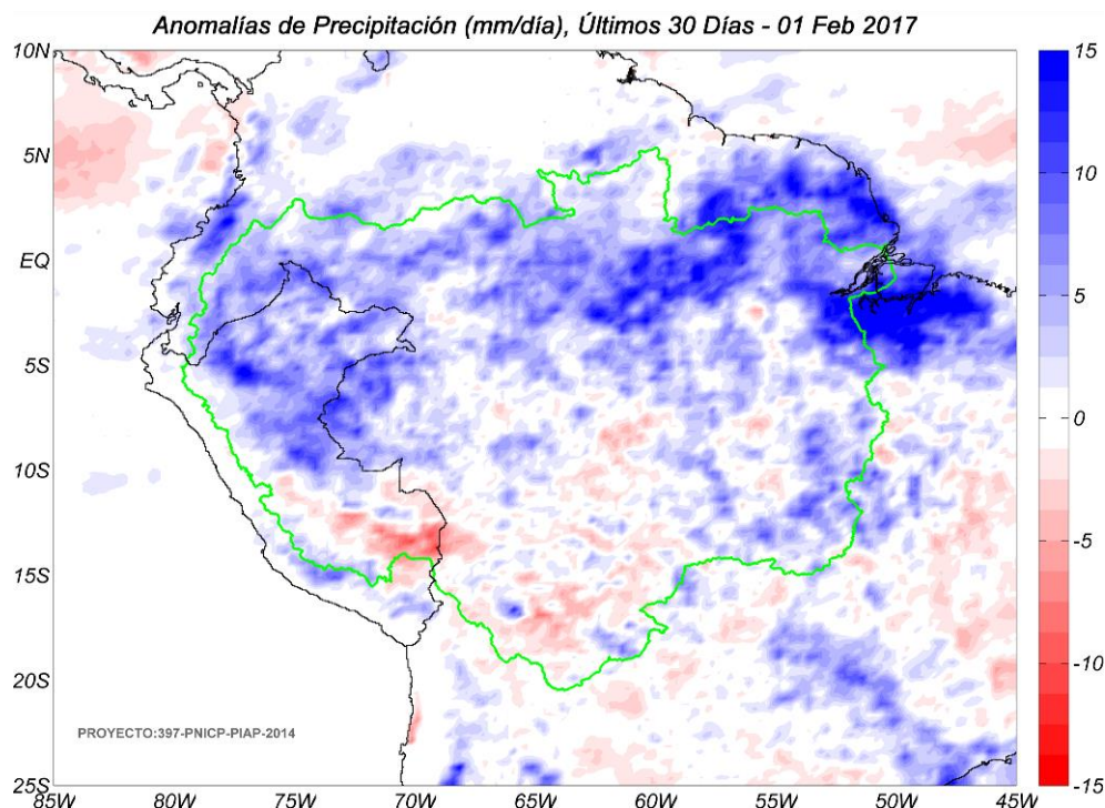
Fig. 4: Anomalías de precipitación estimadas por el TRMM-RT en mm/día hasta 01 de febrero de 2017. Las anomalías fueron calculadas con respecto al periodo base promedio 2000-2015. Se muestra límites de la cuenca Amazónica en línea verde. Las anomalías de precipitación del TRMM-RT actualizadas a tiempo real puede verse en: http://www.igp.gob.pe/eventos-extremos-amazonia-peruana/
