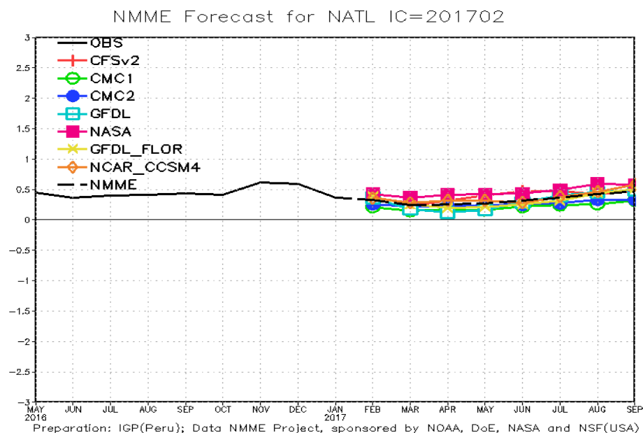
Fig. 9: Pronóstico de las anomalías de temperatura superficial del mar (TSM) para la región del Atlántico tropical Norte (NATL: 5°N-20°N, 30°W-60°W), a partir de condiciones de fines de enero 2017. Fuente: Instituto Geofísico del Perú (IGP).
