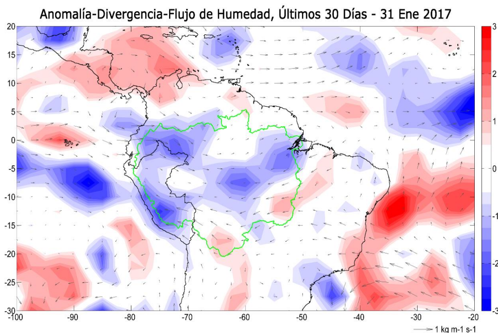
Fig. 3: Anomalías de flujo de humedad integrado en los niveles de 1000 hPa a 300 hPa de la atmósfera y su divergencia. El periodo corresponde de 01 al 31 de enero 2017. Las anomalías son calculadas utilizando el periodo base de 1970 a 2015. Se muestra límites de la cuenca Amazónica en línea verde.
