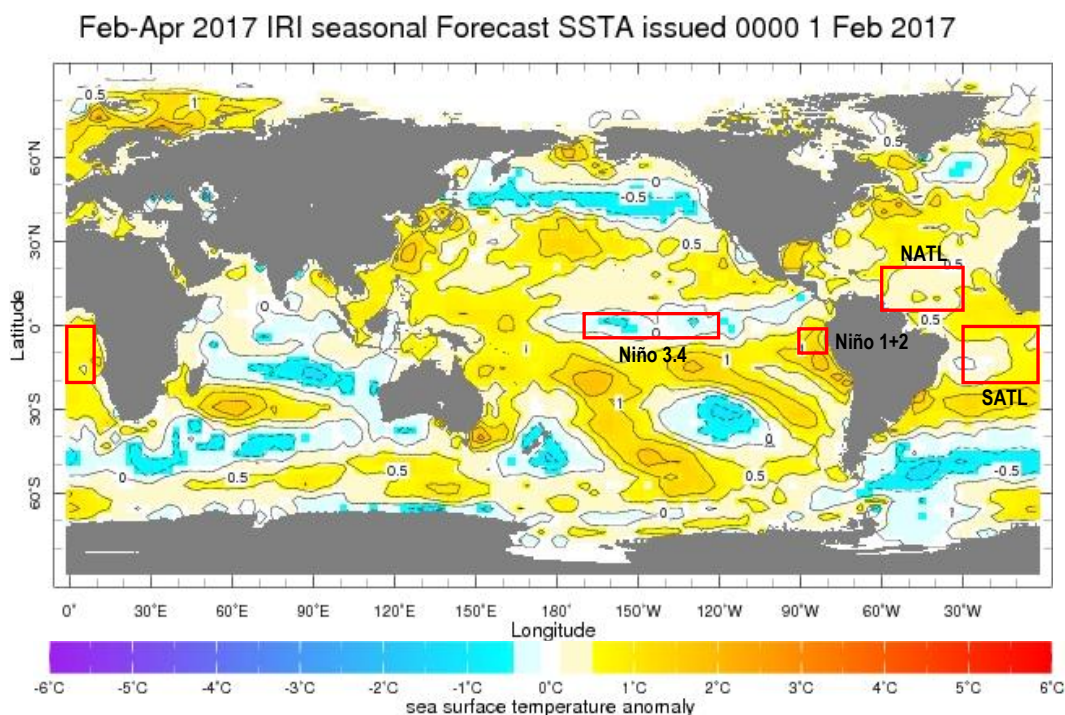
Fig. 7: Pronóstico de las anomalías de temperatura superficial del mar (°C) a nivel global, para el trimestre febrero-abril (FMA) 2017. Rectángulos rojos indican regiones de análisis. Fuente: International Research Institute for Climate and Society (IRI).
