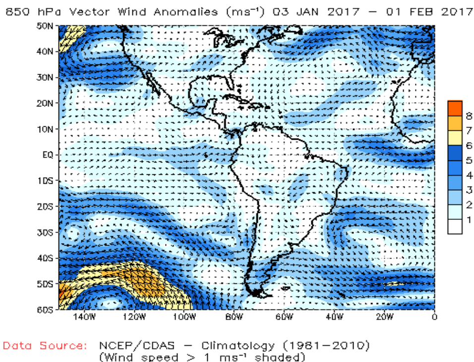
Fig. 2: Anomalía de vientos en niveles bajos (850 hPa) de la atmósfera, (del 03 de enero al 01 de febrero de 2017). Las anomalías fueron calculadas utilizando el periodo base los promedios entre 1981 y 2010. Fuente: NOAA/NCEP.
