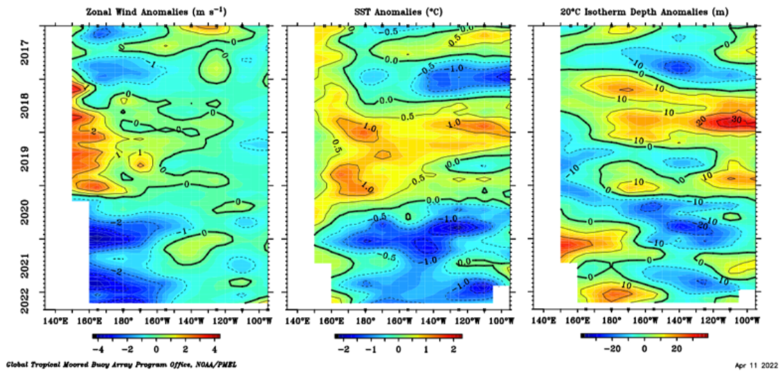
Figura 2. Promedio mensual de la anomalía del viento zonal (a), de la profundidad de la isoterma de 20 ^{\circ}\text{C} (b) y de la temperatura superficial del mar (c) a lo largo de la franja ecuatorial del Pacífico (2°S-2°N). Esta imagen se elaboró de otras que se obtienen del proyecto TAO: www.pmel.noaa.gov/tao .
