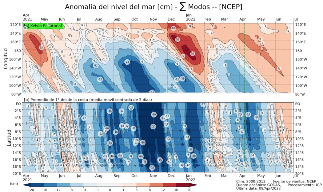
Figura 13. Simulación numérica de la anomalía del nivel del mar (cm) a lo largo de la franja ecuatorial del océano Pacífico (panel superior) y a lo largo de la costa peruana (panel inferior). Esta simulación se realizó con el modelo oceánico multimodal forzado con los vientos del reanalysis de NCEP. La línea verde entrecortada indica el inicio de la simulación del pronóstico. Elaborado por el IGP.
