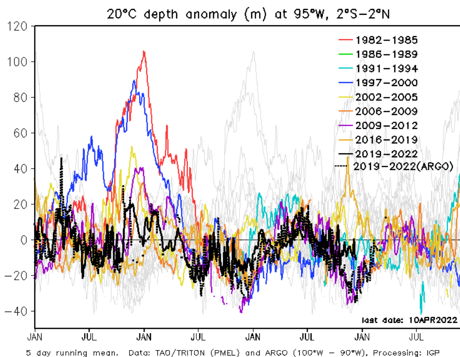
Figura 6. Anomalía de la profundidad de la isoterma de 20 °C (m) en 95°W y promediada entre 2°S y 2°N, con datos de ARGO (línea negra cortada) y TAO (línea negra continua). Elaborado por el IGP.
