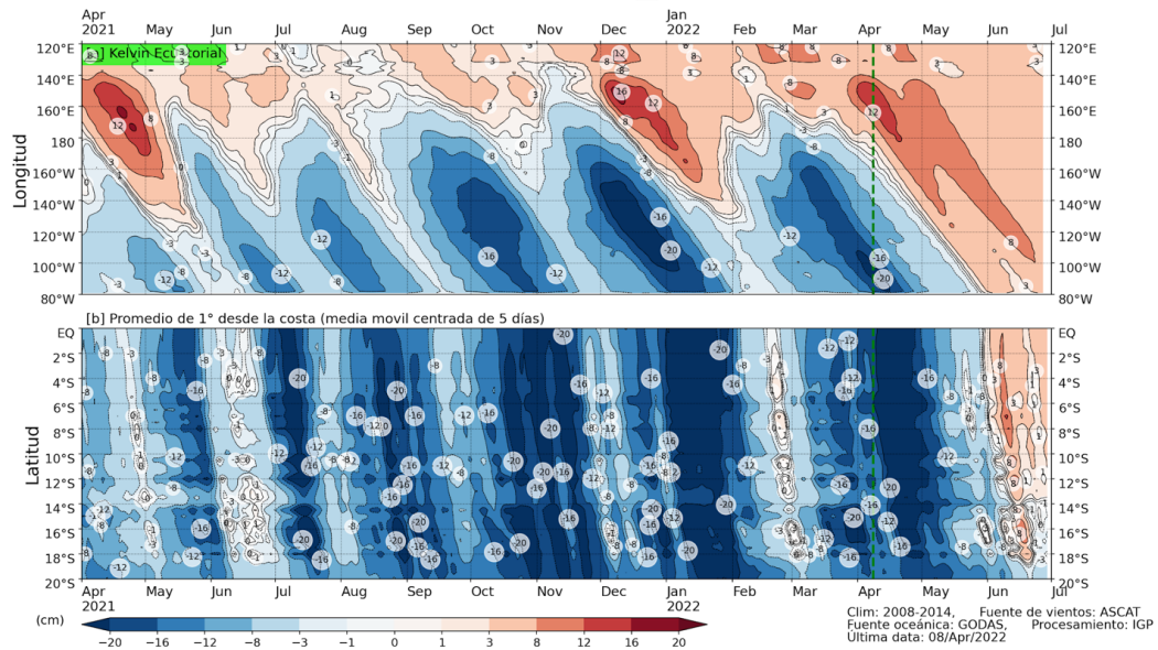
Figura 12 Simulación numérica de la anomalía del nivel del mar (cm) a lo largo de la franja ecuatorial del océano Pacífico (panel superior) y a lo largo de la costa peruana (panel inferior). Esta simulación se realizó con el modelo oceánico multimodal forzado con el producto de vientos denominado ASCAT . La línea verde entrecortada indica el inicio de la simulación del pronóstico. Elaborado por el IGP.
