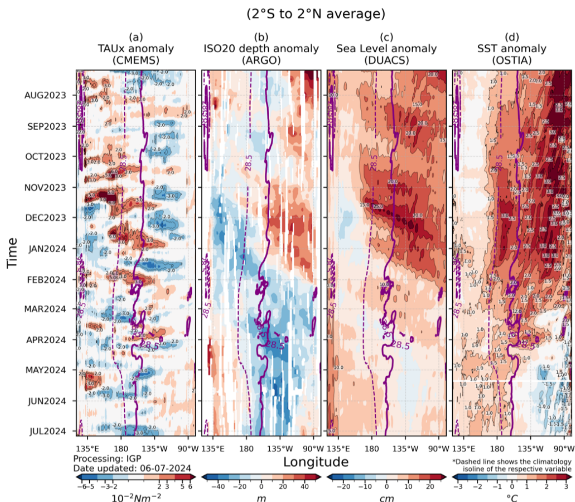
Figura 4. Diagrama longitud-tiempo en la franja ecuatorial de las anomalías, de izquierda a derecha, a) del esfuerzo de viento zonal (ASCAT), b) de la profundidad de la termoclina (ARGO), c) del nivel del mar (DUACS) y d) de la temperatura del mar (OSTIA). La línea morada continua (entrecortada) indica laposición observada (climatológica) de la isoterma de 28.5 ° C. Elaborado por el IGP.
