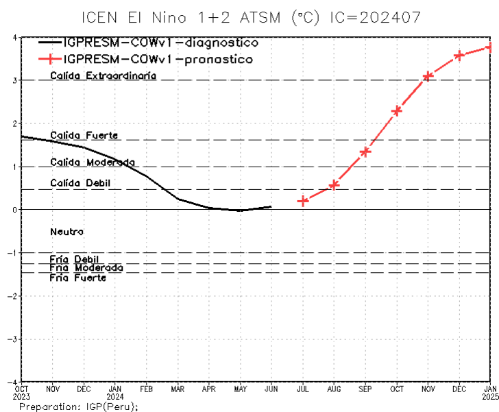
Figura 17. Pronóstico del ICEN de julio de 2024 a enero de 2025, generado por el Modelo Regional Earth SystemModel CROCO-OASIS-WRF v.1' (IGP RESM-COW v.1) con condiciones iniciales de julio.
