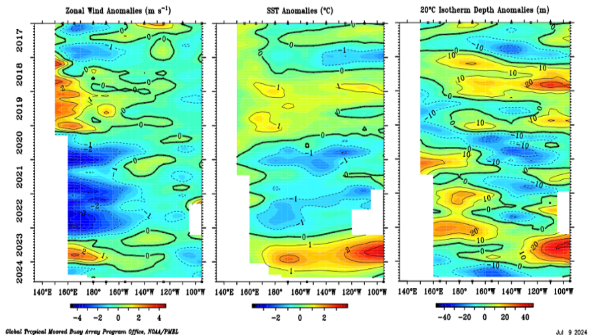
Figura 2. Promedio mensual a lo largo de la franja ecuatorial del Pacífico (2°S-2°N) de las anomalías del viento zonal (panel izquierdo), de la temperatura superficial del mar (panel central) y de la profundidad de la isoterma de 20 °C (panel derecho). Esta imagen se elaboró de otras que se obtienen del proyecto TAO: www.pmel.noaa.gov/
