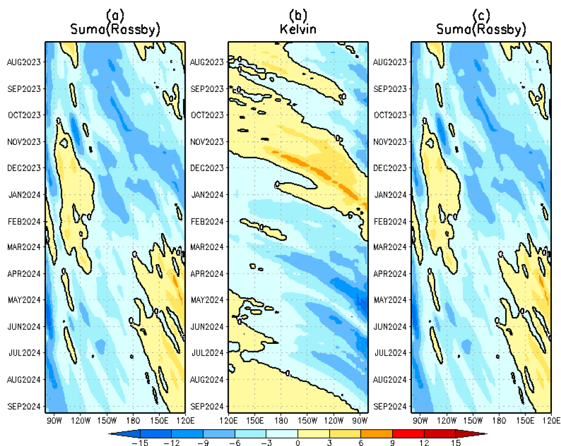
Figura 12. Igual que la Figura 45 pero el modelo es forzado con termoclina variable. Fuente: IGP.
