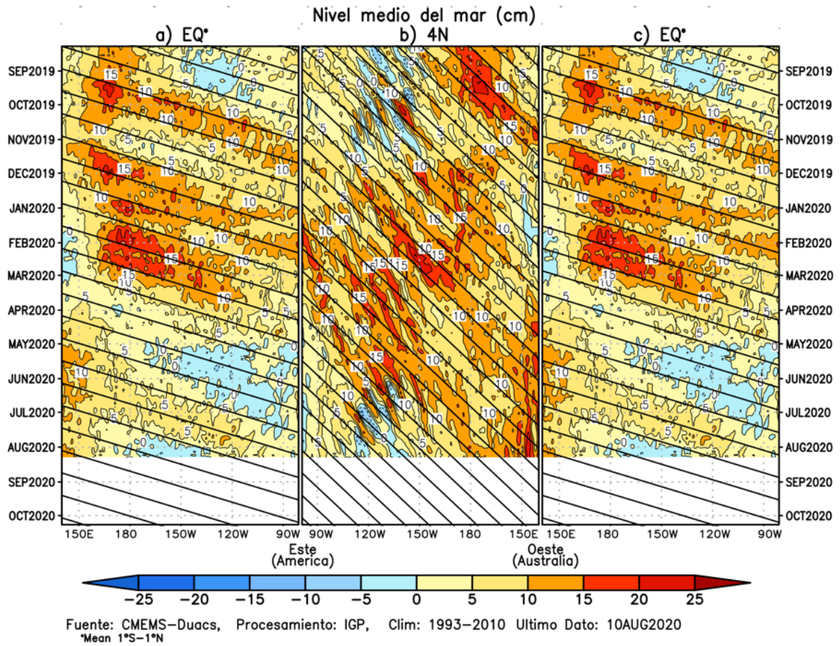
Figura 4. Diagramas longitudin- tiempo de la anomalía del nivel medio del mar en el Pacifico usando el producto DUACS. Las figuras (a) y (c) son las mismas y representan la información a lo largo de la línea ecuatorial, mientras que (b) a lo largo de 4°N pero con el eje zonal de Este a Oeste. Las líneas diagonales indican la trayectoria teórica de la onda de Kelvin (a y c) y Rossby (b) si tuvieran una velocidad aproximada de 2.6 m/s y 0.87 m/s, respectivamente. Elaborado por el IGP.
