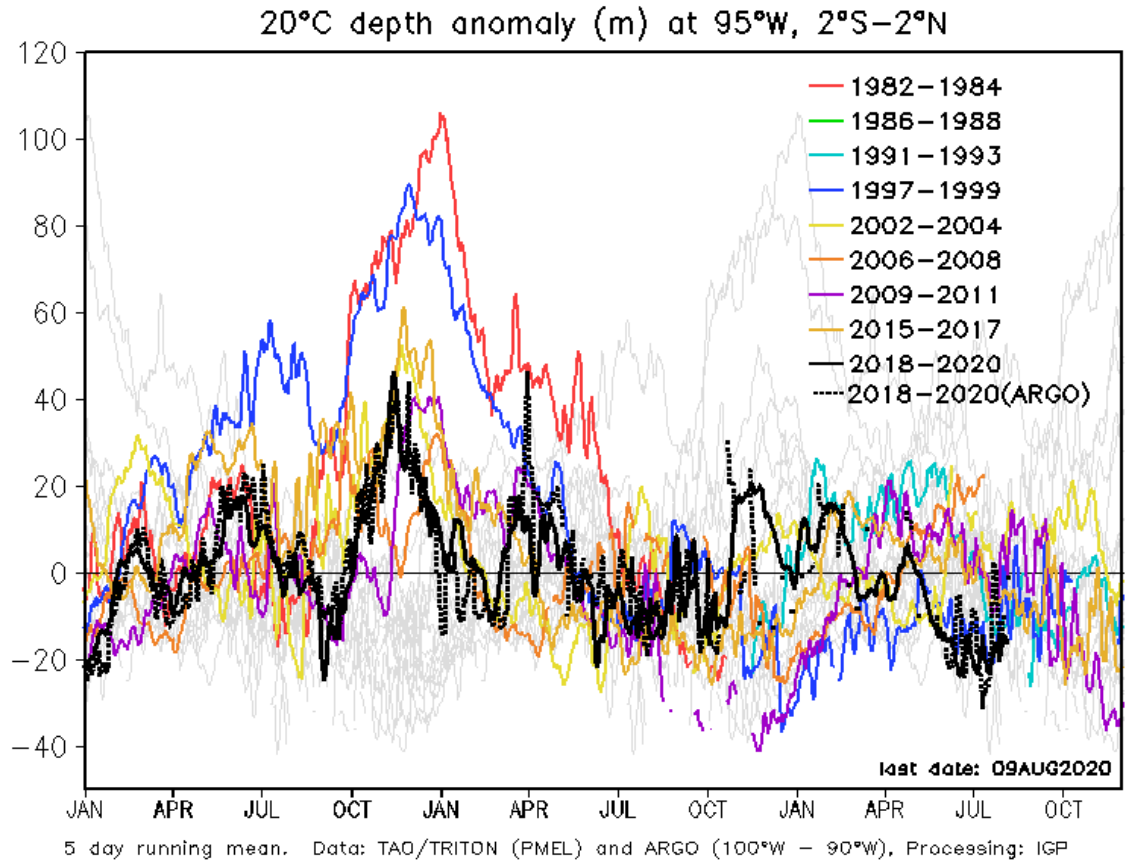
Figura 6. Anomalía de la profundidad de la isoterma de 20 °C (m) en 95° W ,2°S-2°N, con datos de ARGO y TAO. Elaboración: IGP.
