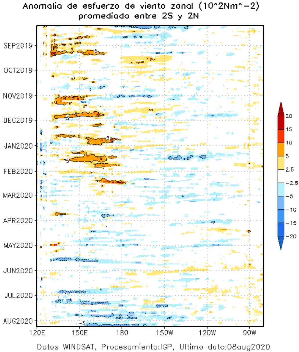
Figura 3. Diagrama longitud-tiempo de las anomalías del esfuerzo de viento zonal ecuatorial basado en datos del producto WINDSAT hasta el 08 de agosto 2020. Elaboración: IGP.
