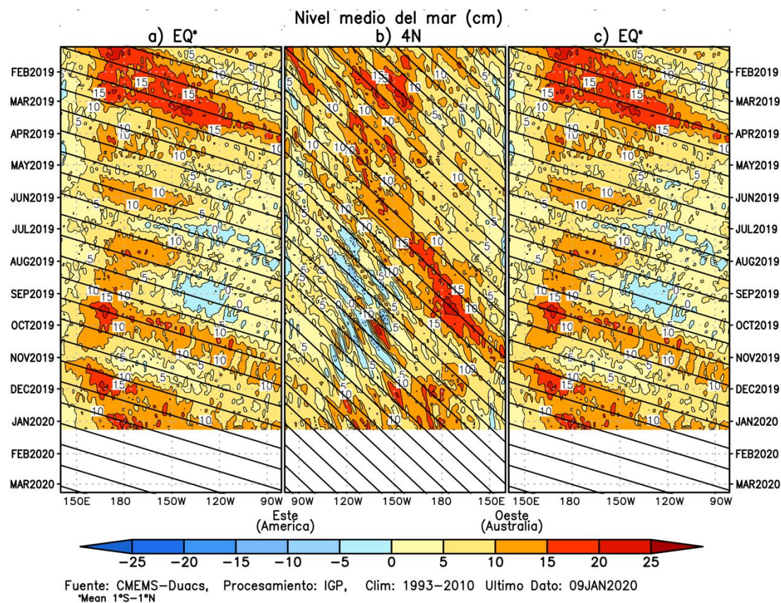
Figura 4. Diagramas longitud- tiempo de la anomalía del nivel medio del mar en el Pacifico usando el producto DUACS. Las figuras (a) y (c) son las mismas y representan la información a lo largo de la línea ecuatorial, mientras que (b) a lo largo de 4°N pero con el eje zonal de Este a Oeste. Las líneas diagonales indican la trayectoria teórica de la onda Kelvin (a y c) y Rossby (b) si tuvieran una velocidad aproximada de 2.6 m/s y 0.87 m/s, respectivamente . Elaborado por el IGP.
