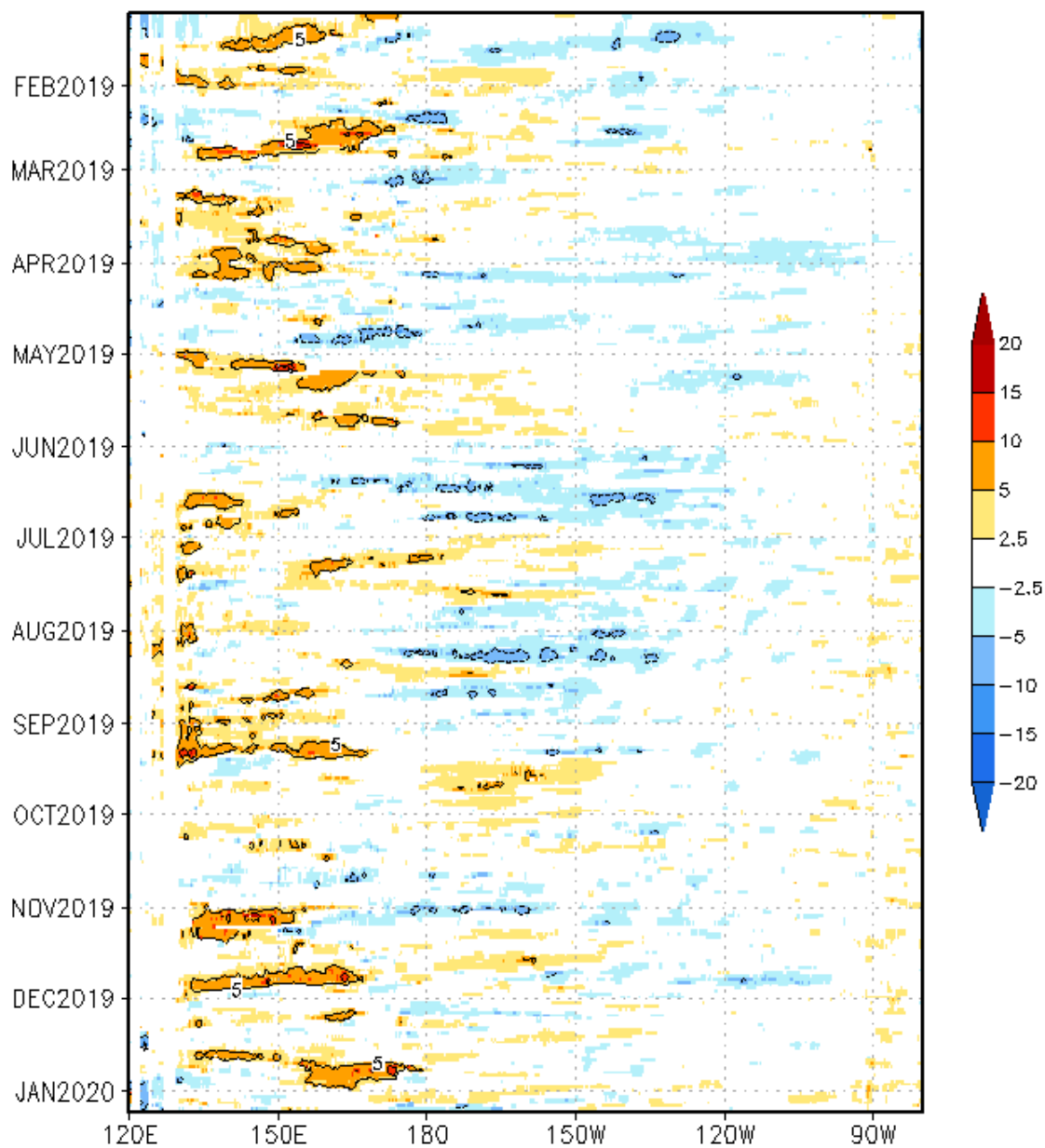
Figura 3. Diagrama longitudin-tempo de las anomalías del esfuerzo de viento zonal ecuatorial basado en datos del producto WINDSAT hasta el 08 de enero 2020. Elaboración: IGP.
