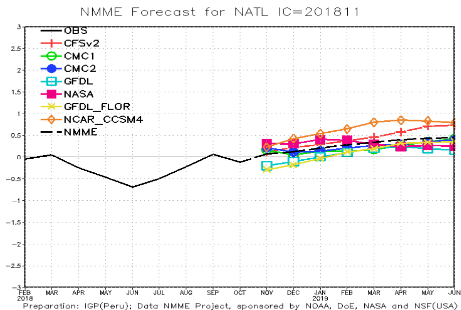
Fig. 9: Pronóstico de las anomalías de temperatura superficial del mar (TSM) para la región del Atlántico tropical Norte (NATL: 5°N-20°N, 30°W-60°W), a partir de condiciones de fines de octubre 2018. Fuente: Instituto Geofísico del Perú (IGP) .
