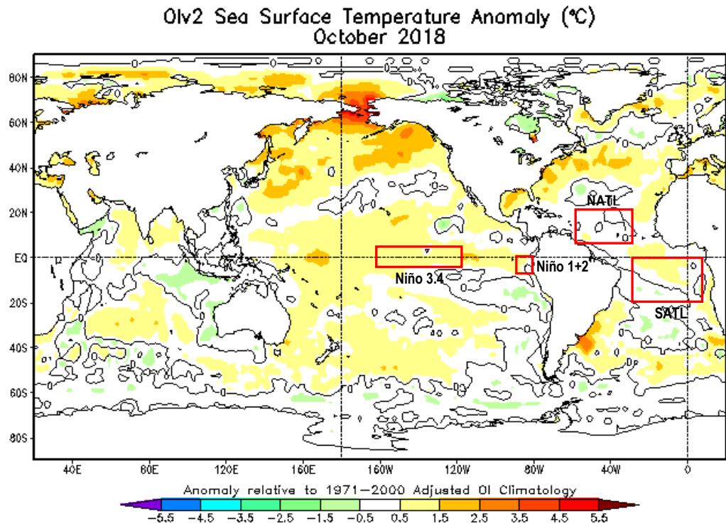
Fig. 1: Anomalías de temperatura superficial del mar (TSM) en °C del mes de octubre de 2018. Las anomalías son calculadas utilizando la climatología del periodo base 1971-2000. Fuente CPTEC/INPE/BRASIL.
