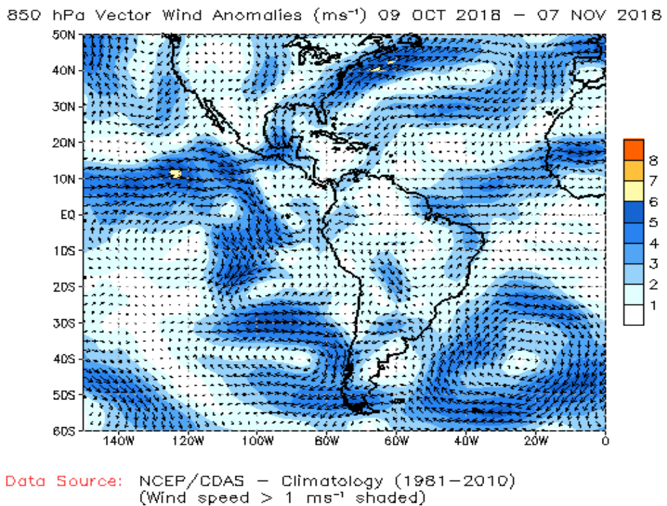
Fig. 2: Vectores de Anomalías de viento en niveles bajos (850 hPa) de la atmósfera, (del 09 de octubre al 07 de noviembre de 2018). Las anomalías fueron calculadas utilizando el periodo base los promedios entre 1981 y 2010. Fuente: NOAA/NCEP.
