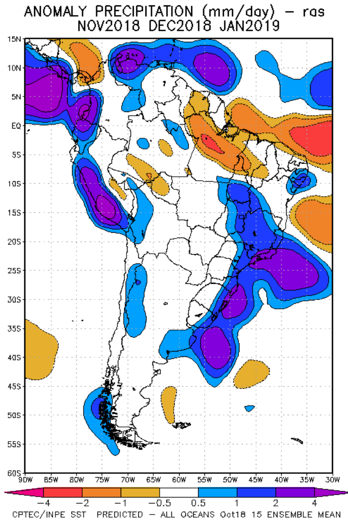
Fig. 10: Pronóstico de las anomalías de la precipitación (mm/día) método ras para el trimestre NDE del 2018 en América del Sur, con datos observados de fines del mes de octubre de 2018. Fuente: CPTEC/INPE.
