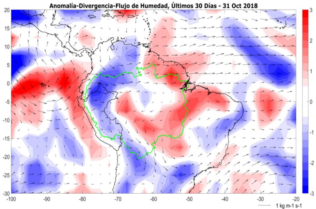
Fig. 3: Anomalías de flujo de humedad integrado en los niveles de 1000 hPa a 300 hPa de la atmósfera (vectores) y su divergencia (colores). El periodo corresponde del 01 hasta el 31 de octubre 2018. Las anomalías son calculadas utilizando el periodo base de 1970 a 2017. Los límites de la cuenca Amazónica se muestran en línea verde.
