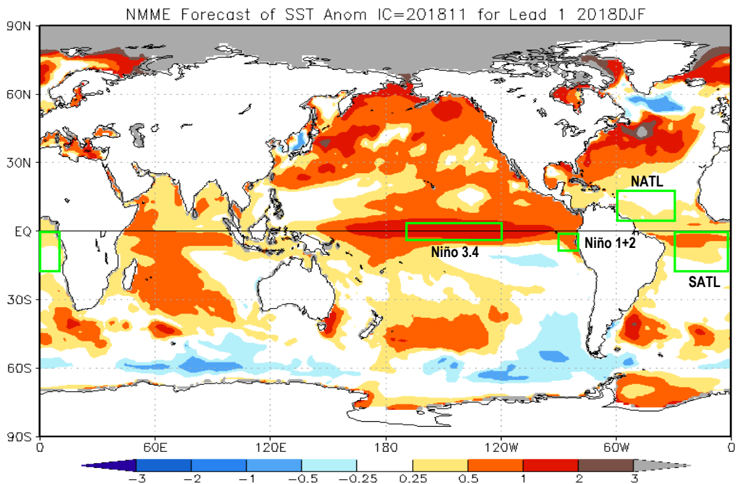
Fig. 7: Pronóstico de las anomalías de TSM (°C) a nivel global, para el trimestre diciembre 2018 - febrero 2019 (DEF). Rectángulos verdes indican regiones de análisis. Fuente: National Multi-Model Ensemble (NMME).
