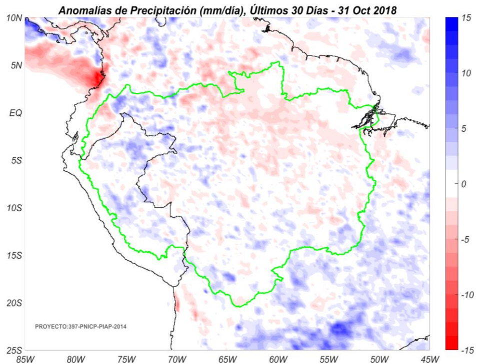
Fig. 4: Anomalías de precipitación estimadas por el TRMM-RT en mm/día hasta 31 de octubre de 2018. Las anomalías fueron calculadas con respecto al periodo base promedio 2000-2017. Se muestra los límites de la cuenca Amazónica en líneas de color verde. Las anomalías de precipitación del TRMM-RT actualizadas a tiempo real puede verse en: http://intranet.igp.gob.pe/eventos-extremos-amazonia-peruana/ .
