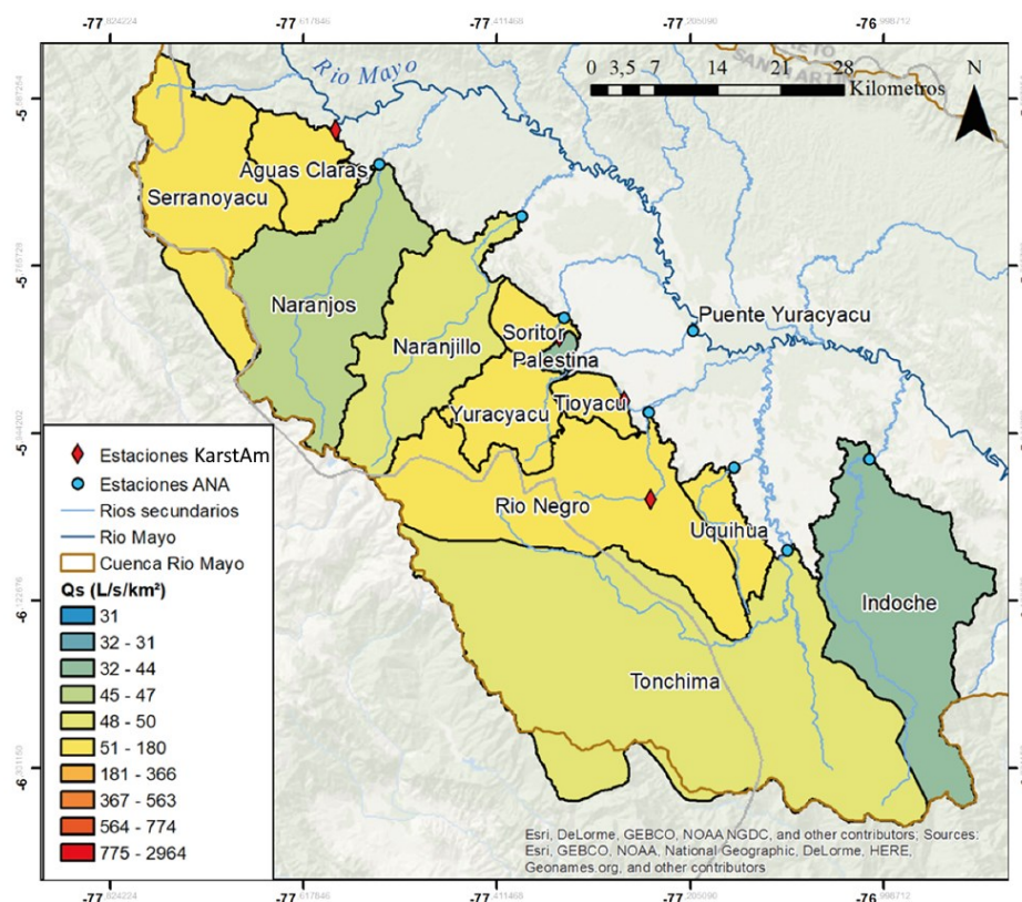
Figura 14 - Mapa de las cuencas hidrogeológicas estimadas y sus caudales específicos, según las cuencas topográficas, la geología y la estructura
