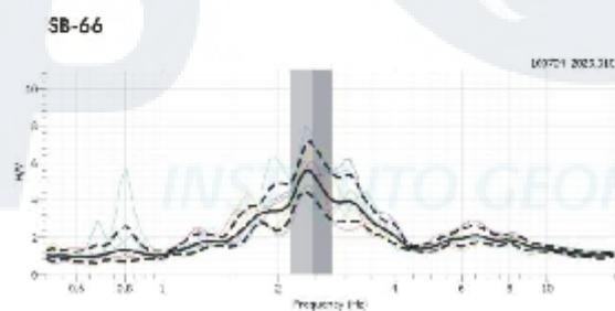
Figura 13c.- Ejemplo de gráficas de razones espectrales obtenidas en la zona céntrica del Distrito de San Bartolo. Los puntos SB-20, SB-51, SB-66 presentan frecuencias predominantes de 2 a 3Hz Otros, ver Figura 13a.
