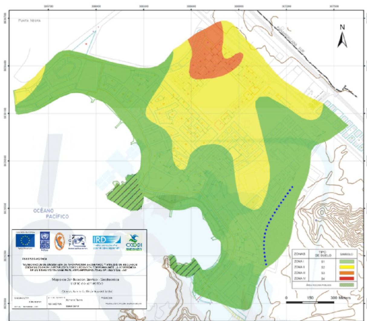
Figura 16.- Mapa de Zonificación Sísmica-Geotécnica (comportamiento Dinámico del Suelo) para el Distrito de San Bartolo
