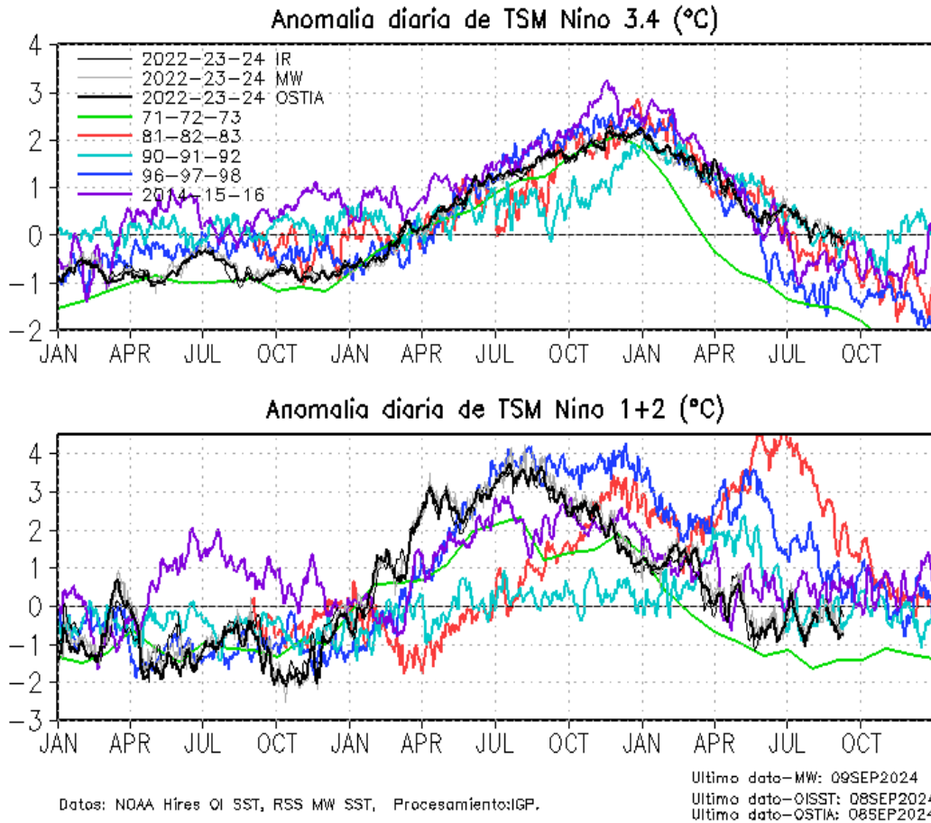
Figura 1. Series de tiempo de la anomalía diaria de la TSM en la región Niño 3.4 (arriba) y en la región Niño 1+2 (abajo). Las líneas en color negro (gruesa), gris y negro (fina) indican la evolución de la anomalía de la TSM usando información infrarroja (IR), microondas (MW) y del producto OSTIA, respectivamente. Las líneas de color verde, rojo, celeste, azul y magenta indican la evolución de la anomalía de la TSM para los periodos 1971-1973, 1981-1983, 1990-1992, 1996-1998 y 2014-2016. Elaborado por el IGP.
