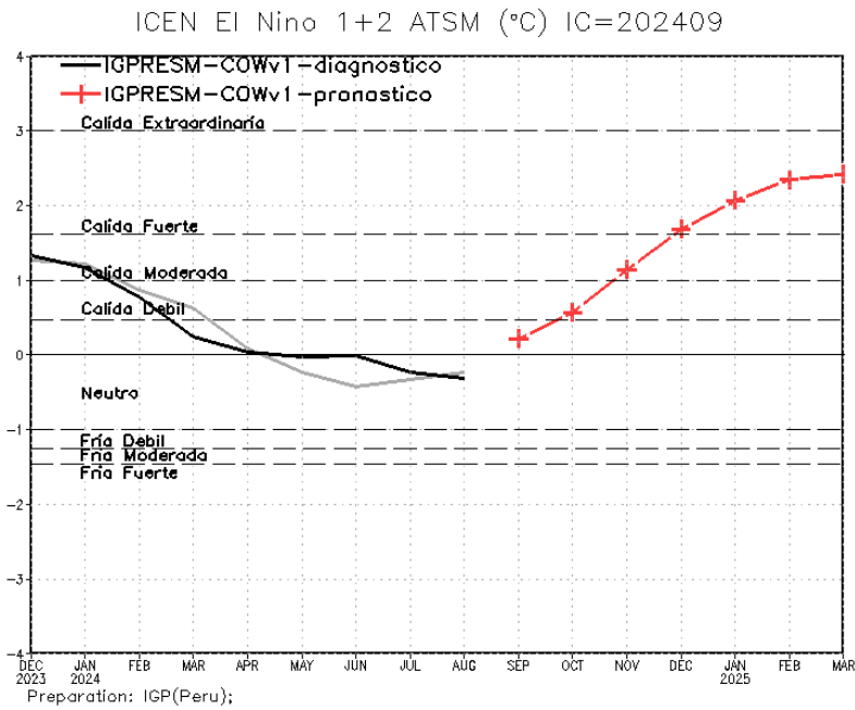
Figura 17. Pronóstico del ICEN de setiembre de 2024 a marzo de 2025 (línea roja con cruz), generado por el Modelo Regional Earth SystemModel CROCO-OASIS-WRF v.1’ (IGP RESM-COW v.1) con condiciones iniciales de setiembre.
