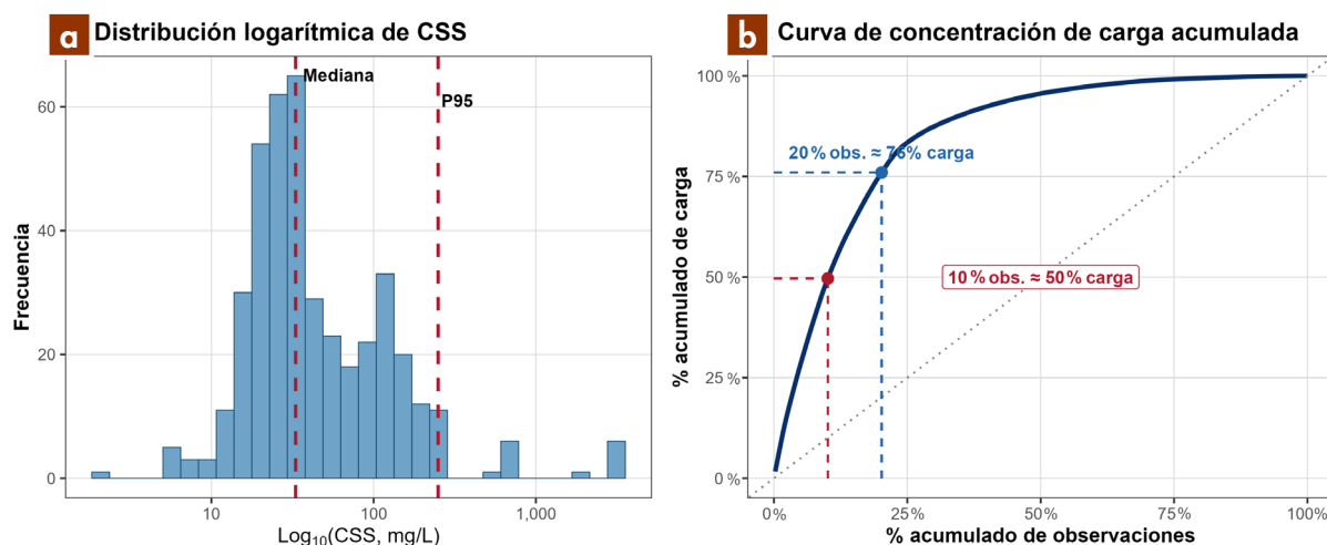
Figura 5.1.1. Monitoreo de la concentración de sedimentos en suspensión en la estación Allato, río Lircay: a) distribución logarítmica de la CSS y b) curva de concentración de carga acumulada.
