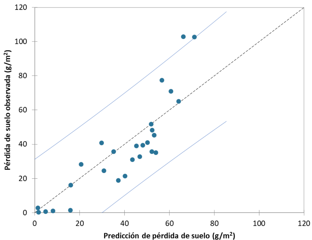
Figura 4.2.9. Validación del modelo: correlación entre la pérdida de suelo observada y predicha (g/m²).
