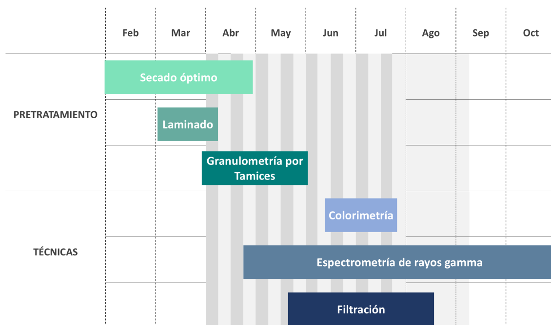
Figura 2.2.5. Balance de tiempos de respuesta y rendimiento analítico ejecutado para el distrito de Lircay en 2023.
