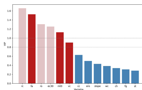
Figura 4.2.8. Importancia de la Variable (VIP): Jerarquía de factores influyentes en la producción de sedimentos.
