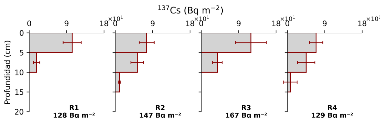
Figura 4.1.1. Distribución de Cs-137 en el perfil del suelo de sitios de referencia.
