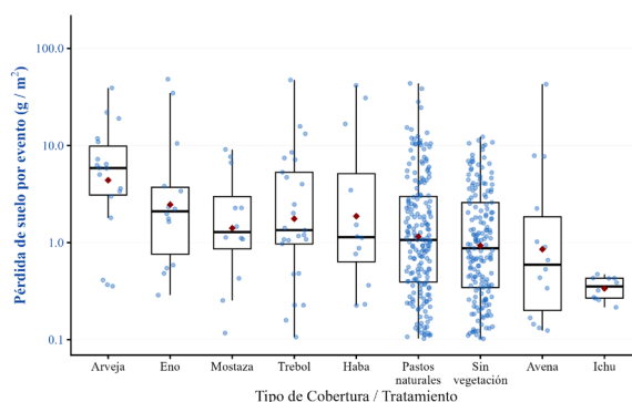
Figura 4.2.5. Variabilidad de la pérdida de suelo por evento (g/m 2 ) según el tipo de cobertura y tratamiento en el distrito de Lircay.
