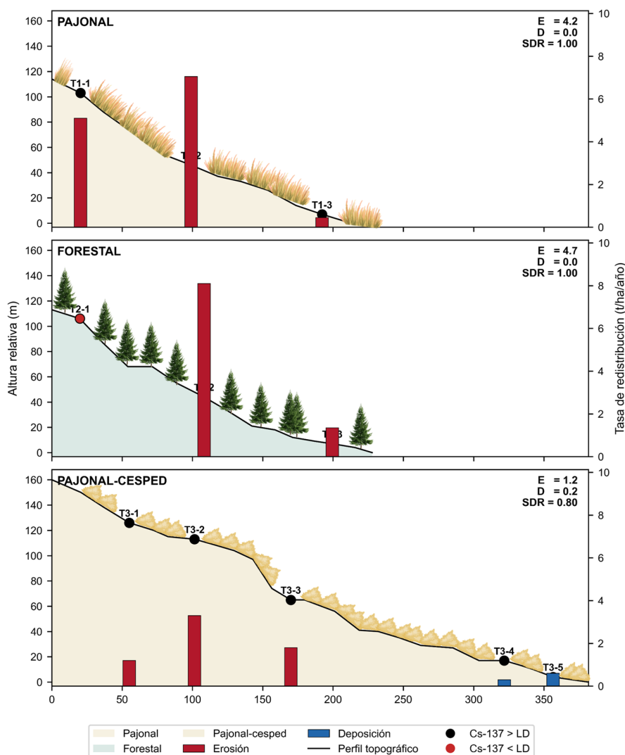
Figura 4.1.7. Tasas de redistribución de suelo e inventarios de Cs-137 en las laderas T1 (pajonal), T2 (forestal) y T3 (pajonal-césped). Los puntos de muestreo se codifican como T[tránsito]-[posición], donde el número tras el guion indica la posición en la ladera de arriba hacia abajo (p. ej., T1-1 corresponde al punto más alto del tránsito 1).
