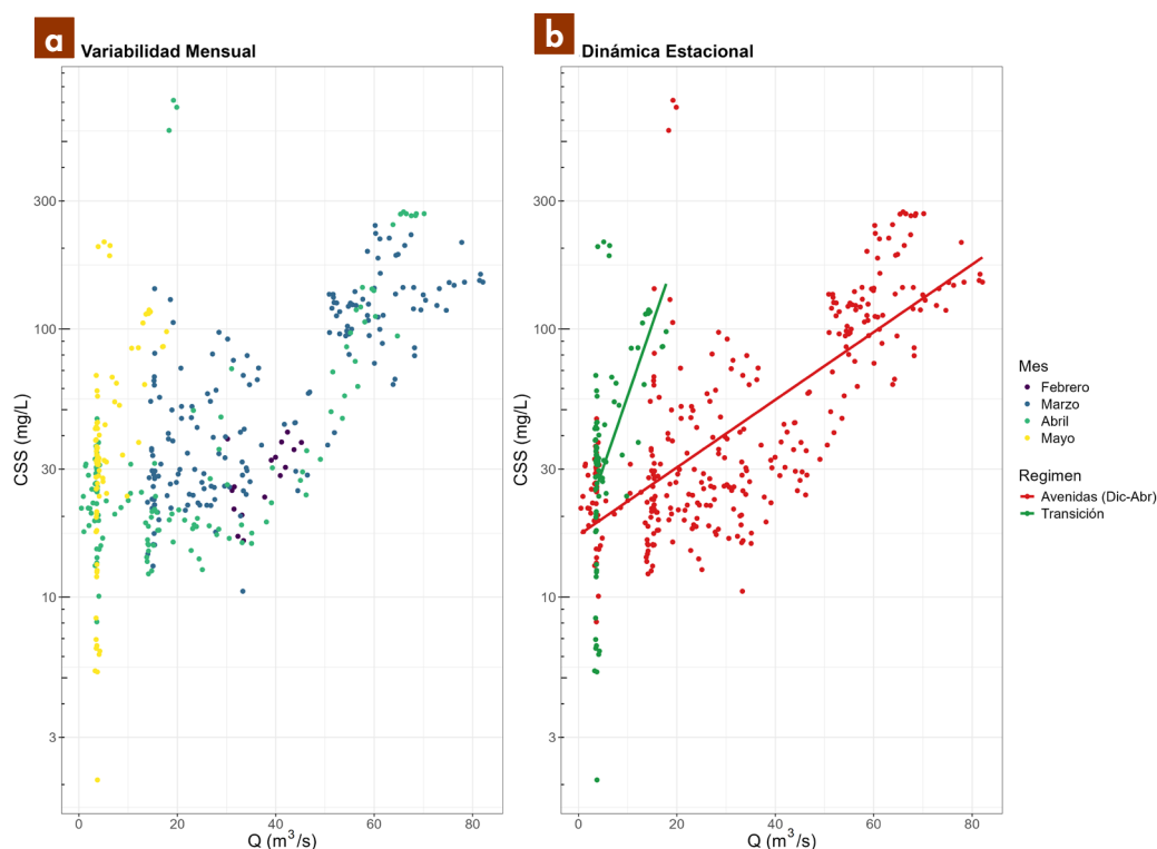
Figura 5.1.2. Relación caudal–CSS y variabilidad temporal del transporte en suspensión en la estación Allato.
