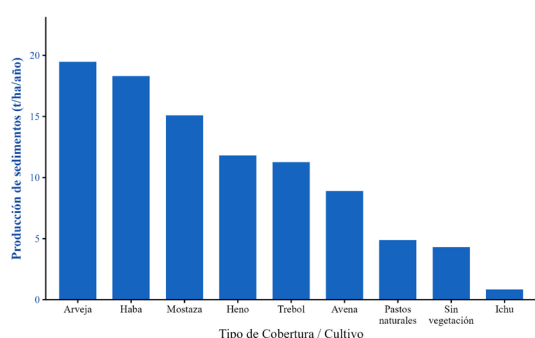
Figura 4.2.6. Producción de sedimentos anualizada (t/ha/año) estimada para los diferentes tratamientos evaluados en Lircay.
