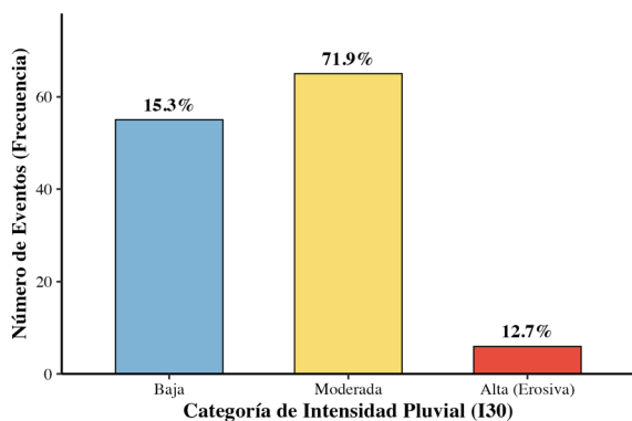
Figura 4.2.4. Clasificación de eventos según su intensidad máxima ( I_{30} ) en el distrito de Lircay. Las etiquetas superiores indican el porcentaje de aporte de cada categoría respecto a la precipitación total acumulada de enero-mayo de 2023.
