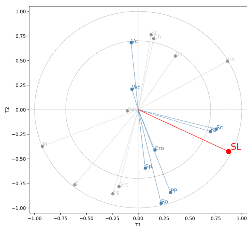
Figura 4.2.7. biplot PLS-R: Relación vectorial entre variables hidropedológicas y pérdida de suelo.
