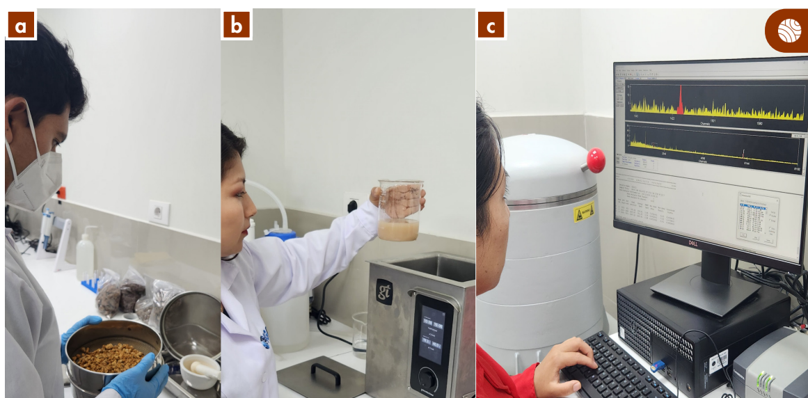
Figura 2.2.3. Procesamiento para matrices sólidas: a) Clasificación granulométrica por tamizaje; b) Acondicionamiento de muestras para difracción láser; y c) Preparación de geometría para espectrometría de rayos gamma.
