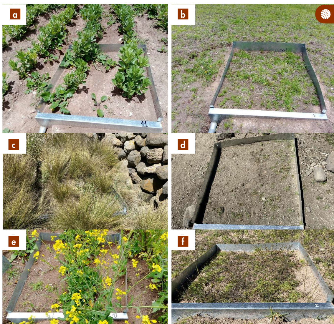
Figura 4.2.1. Red de microparcelas experimentales para el monitoreo de erosión hídrica bajo diferentes tipos de cobertura vegetal en Jatumpata y Tambranco: a) cultivos de habas en hileras, b) pastos naturales cortos, c) vegetación densa (ichu), d) suelo desnudo con presencia de clastos, e) cultivo de mostaza en floración, y f) rastrojo o cobertura degradada.
