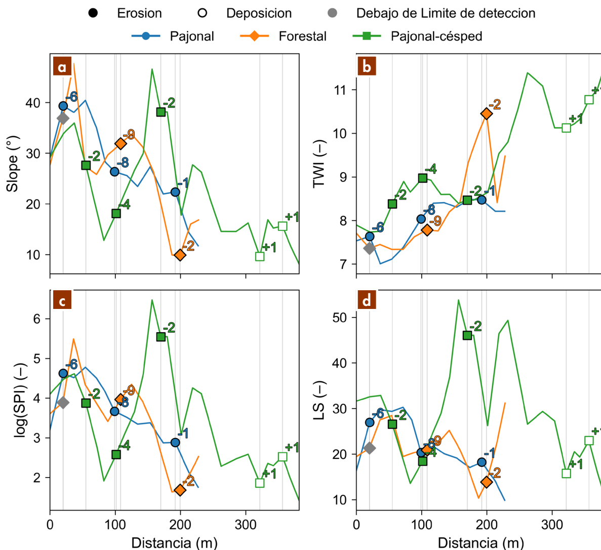
Figura 4.1.8. Influencia del factor topográfico en la redistribución del suelo en las laderas muestreadas.
