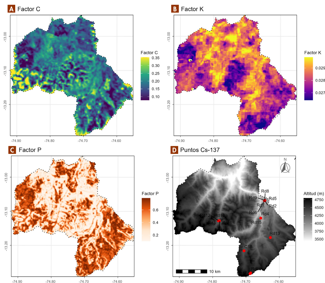
Figura 6.1.1. Variables de ingreso del modelo distribuido WaTEM/SEDEM en el distrito de Lircay. A) Cobertura vegetal del distrito de Lircay. B) Factor K, estimado a partir de datos de SoilGrids. C) Distribución espacial del factor P en el distrito. D) Tasas de erosión medidas con Cs-137, utilizadas en la etapa de calibración del modelo.
