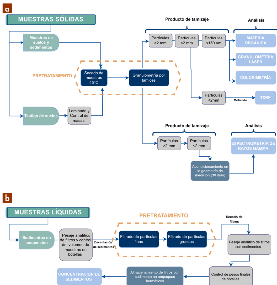
Figura 2.2.2. Flujo analítico de pretratamiento. a) Secuencia de procesamiento y obtención de derivados para matrices sólidas; b) sistema de separación de fases para la cuantificación de sedimentos en suspensión.
