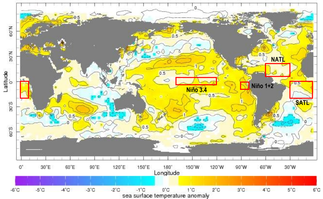
Fig. 7: Pronóstico de las anomalías de temperatura superficial del mar (°C) a nivel global, para el trimestre mayo-julio (MJJ) 2017. Rectángulos rojos indican regiones de análisis. Fuente: International Research Institute for Climate and Society (IRI) .
