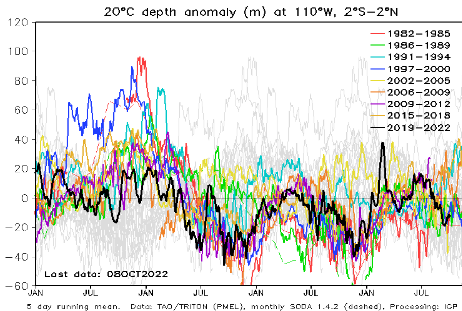
Figura 6. Anomalía de la profundidad de la isoterma de 20 °C (m) en 110°W y promediada entre 2°S y 2°N. La data usada para este calculo proviene de las boyas TAO. Elaborado por el IGP.
