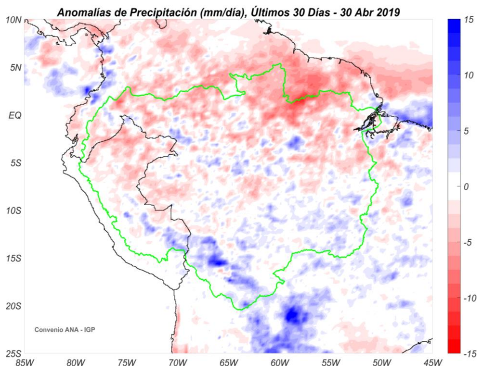
Fig. 4: Anomalías de precipitación estimadas por el TRMM-RT en mm/día hasta 30 de abril de 2019. Las anomalías fueron calculadas con respecto al periodo base promedio 2000-2018. Se muestra los límites de la cuenca Amazónica en líneas de color verde. Las anomalías de precipitación del TRMM-RT actualizadas a tiempo real puede verse en: http://intranet.igp.gob.pe/eventos-extremos-amazonia-peruana/ .
