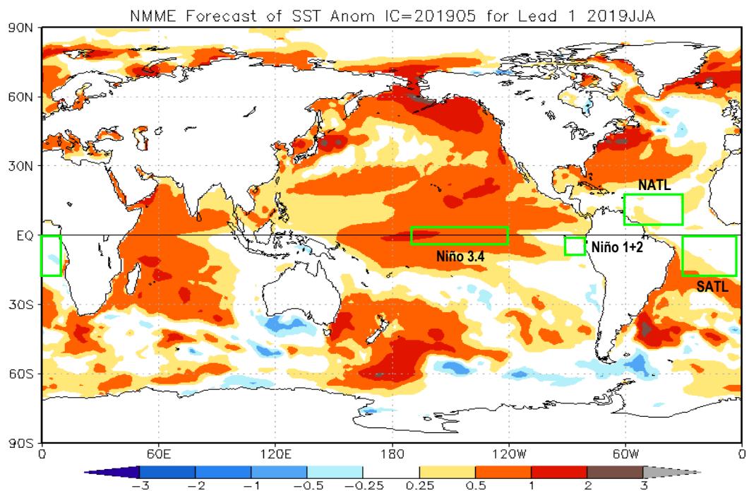
Fig. 7: Pronóstico de las anomalías de TSM (°C) a nivel global, para el trimestre junio-julio-agosto 2019 (JJA). Rectángulos verdes indican regiones de análisis. Fuente: National Multi-Model Ensemble (NMME) .
