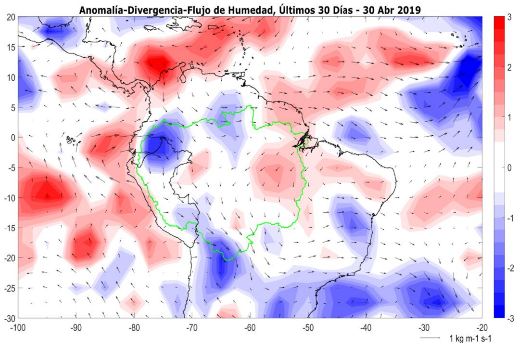
Fig. 3: Anomalías de flujo de humedad integrado en los niveles de 1000 hPa a 300 hPa de la atmósfera (vectores) y su divergencia (colores). El periodo corresponde del 01 hasta el 30 de abril 2019. Las anomalías son calculadas utilizando el periodo base de 1970 a 2018. Los límites de la cuenca Amazónica se muestran en línea verde.
