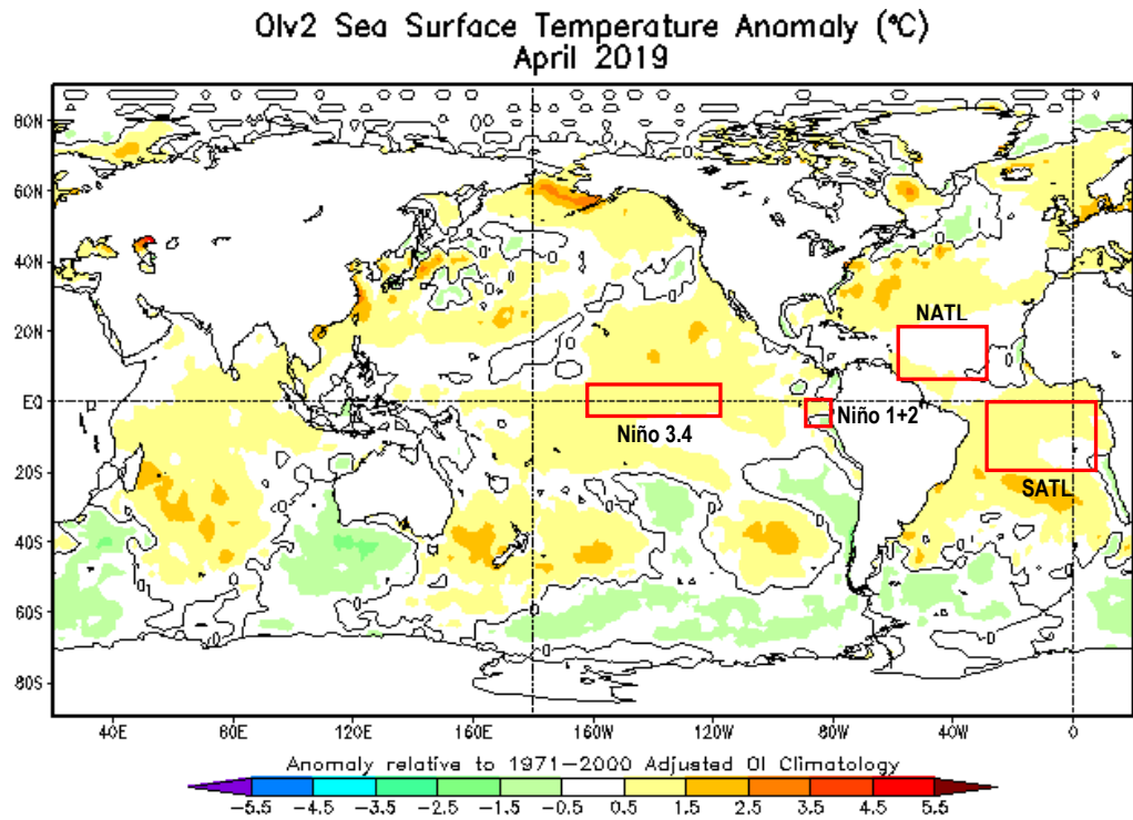
Fig. 1: Anomalías de temperatura superficial del mar (TSM) en °C del mes de abril de 2019. Las anomalías son calculadas utilizando la climatología del periodo base 1971-2000. Fuente CPTEC/INPE/BRASIL.
