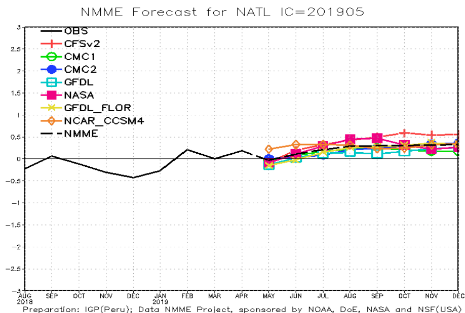
Fig. 9: Pronóstico de las anomalías de temperatura superficial del mar (TSM) para la región del Atlántico tropical Norte (NATL: 5°N-20°N, 30°W-60°W), a partir de condiciones de fines de abril 2019. Fuente: Instituto Geofísico del Perú (IGP) .
