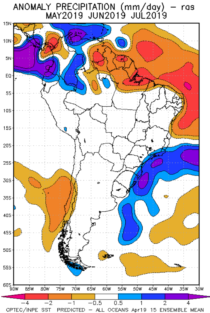
Fig. 10: Pronóstico de las anomalías de la precipitación (mm/día) método ras para el trimestre MJJ del 2019 en América del Sur, con datos observados de fines del mes de abril de 2019. Fuente: CPTEC/INPE.
