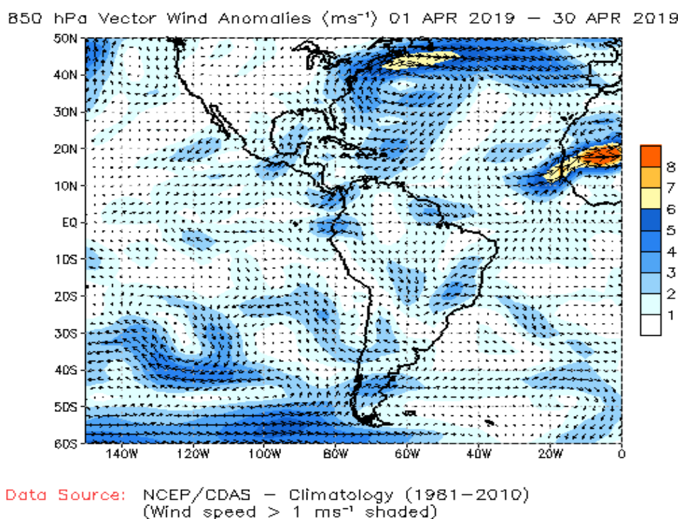
Fig. 2: Vectores de Anomalías de viento en niveles bajos (850 hPa) de la atmósfera, (del 01 al 30 de abril de 2019). Las anomalías fueron calculadas utilizando el periodo base los promedios entre 1981 y 2010. Fuente: NOAA/NCEP.
