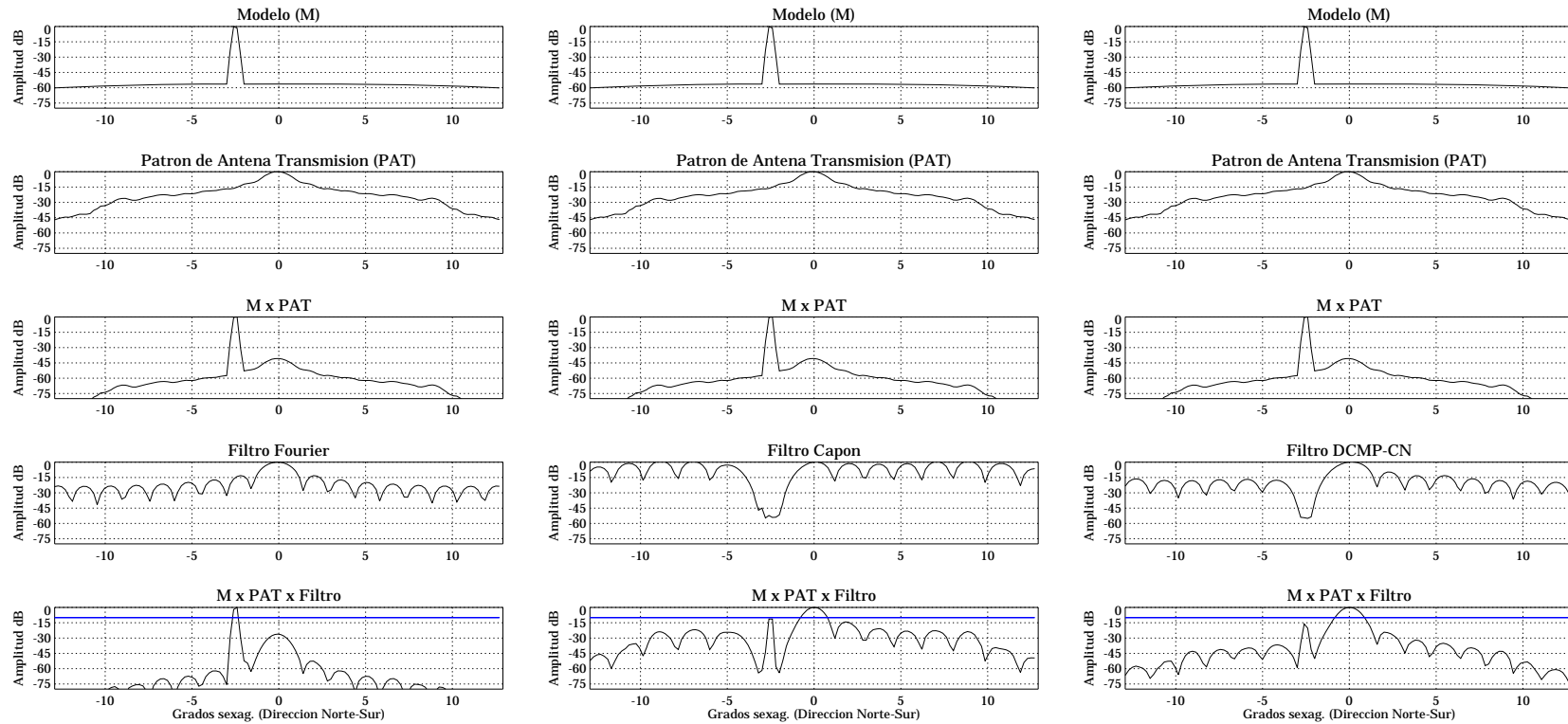
Figura 29. Resultados integrados respecto a la direcci3n 141° (Secci3n AA de la Figura 22) y normalizados en cada etapa del proceso, correspondientes a los m3todos de: (a) Fourier, (b) Capon, (c) DCMP-CN.
