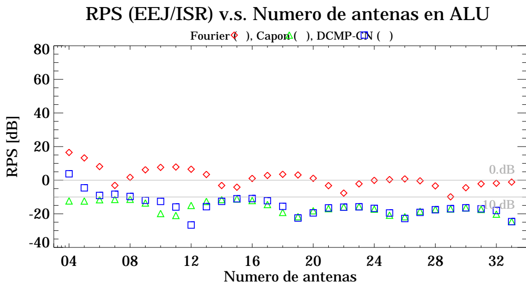
Figura 35. RPS en función del número de antenas del arreglo lineal uniforme para 40dB RPE. Arreglo: 25m de separación y dirección 141°.
