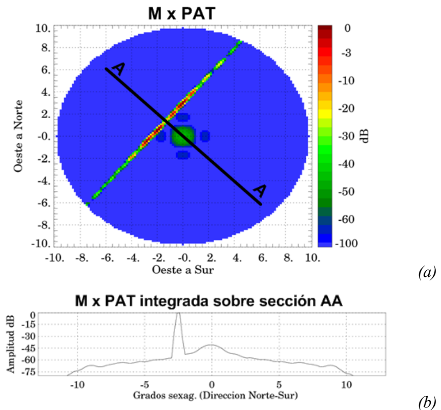
Figura 22. (a) Distribuciones de brillo después de que el modelo original (M) se afecte por el patrón de antena de transmisión (PAT), notar orientación de Sección AA transversal a la dirección del EEJ, (b) Señales integradas sobre Sección AA.
