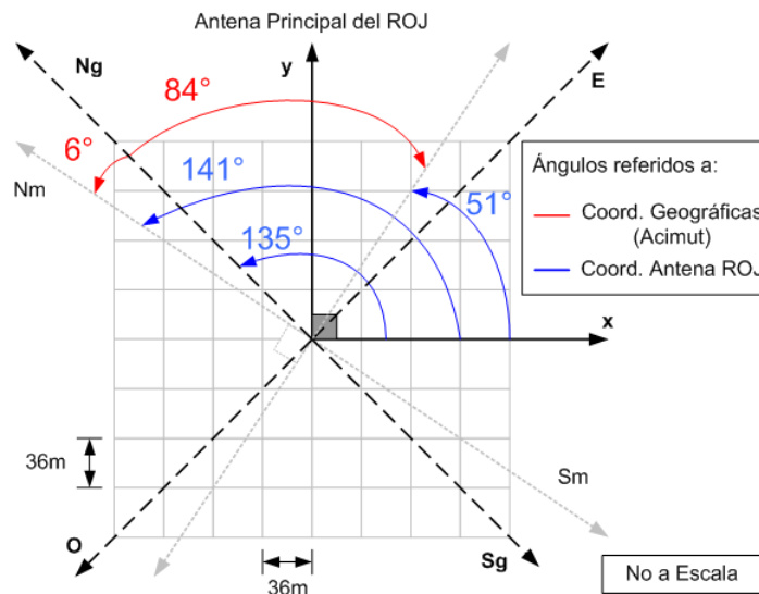
Figura 16. Sistema de Coordenadas establecido, Geográfico (ángulos en Rojo), y de acuerdo con los ejes de la antena principal del ROJ (ángulos en Azul). Notar que la dirección del Norte magnético (Nm) está desplazada 6^\circ aproximadamente del Norte geográfico (Ng) según modelo IGRF (IUGG-IAGA, 2005).
