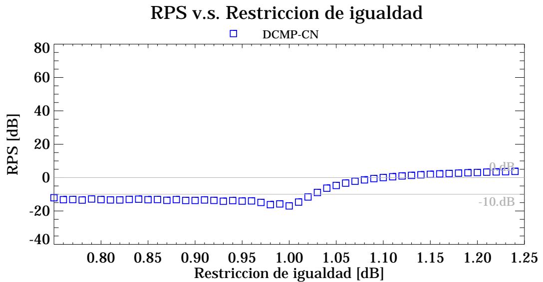
Figura 21. Relación de Potencia de Salida (RPS) respecto al valor de la restricción de igualdad. ULA 12 elementos, 25m espaciamiento, dirección 141°, RPE 60dB.
