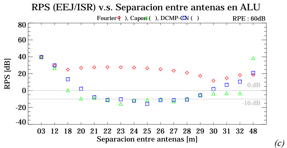
Figura 36. RPS en función de la separación entre antenas del arreglo lineal uniforme. Arreglo: 12 elementos y dirección 141°. Para valores RPE: (a) 50dB, (b) 55dB, y (c) 60dB.
