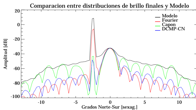
Figura 30. Resultados integrados respecto a la dirección 141° (Sección AA de la Figura 22) al final del filtrado espacial (sin auto-normalización), correspondientes a los métodos evaluados.
