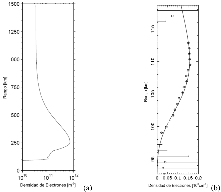
Figura 1. Perfil ionosférico de densidad de electrones correspondientes a la región ecuatorial: (a) Perfil diario de toda la Ionósfera según modelo IRI (Rodríguez, 2008), (b) Perfil diario de la región E medido con radar bistático en el ROJ, en línea continua se muestra la función de densidad de electrones de Chapman (Shume et al., 2005).
