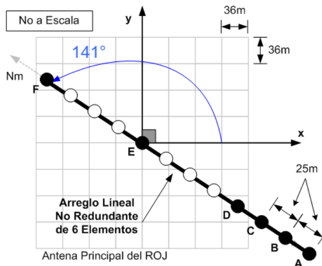
Figura 44. Arreglo Lineal No Redundante con 6 elementos, se muestran la dirección de 141° del arreglo respecto a las coordenadas de la antena principal del ROJ. El diagrama no está a escala. Los círculos sombreados corresponden a las posiciones de las antenas del arreglo, mientras que los círculos vacíos corresponden a las antenas que se dejan de utilizar.
