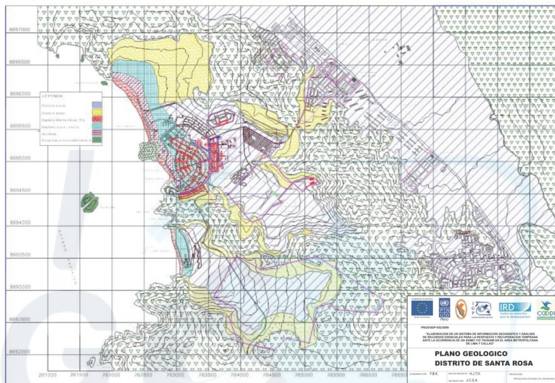
Figura 8.- Mapa geológico para el Distrito de Santa Rosa.
