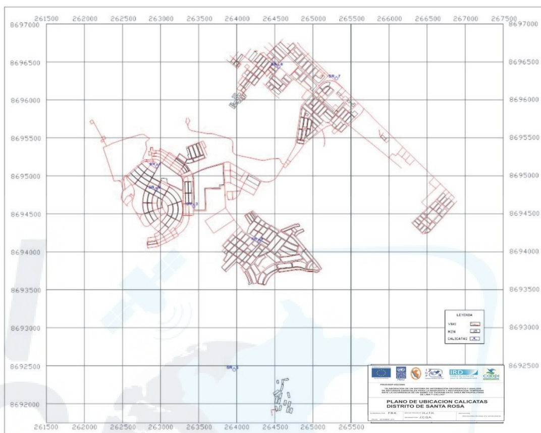
Figura 15.- Distribución espacial de las siete (7) calicatas ejecutadas en el Distrito de Santa Rosa.
