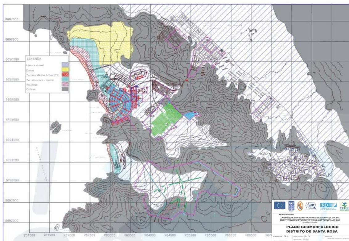
Figura 10.- Mapa geomorfológico para el Distrito de Santa Rosa.
