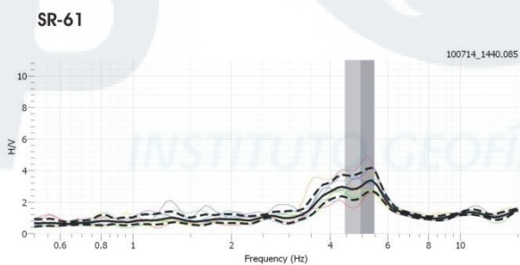
Figura 13d.- Ejemplo de gráficas de razones espectrales obtenidas en el extremo Sur del Distrito de Santa Rosa (Área-3). Los puntos SR-56, SR-60, SR-61 presentan frecuencias que fluctúan entre 5 y 6Hz. Otros, ver Figura 13a.
