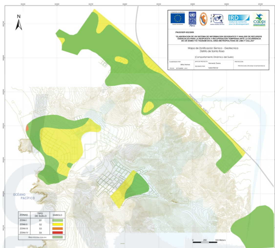
Figura 16.- Mapa de Zonificación Sísmico-Geotécnica (Comportamiento Dinámico del Suelo) para el Distrito de Santa Rosa.
