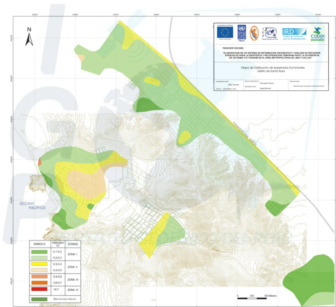
Figura 14.- Mapa de distribución de periodos dominantes para el Distrito de Santa Rosa.
