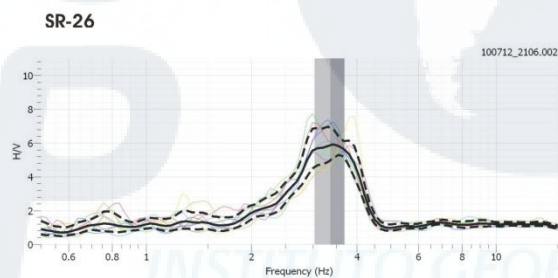
Figura 13a. Ejemplo de gráficas de razones espectrales obtenidas en el extremo NE del Distrito de Santa Rosa (Área-1). Los puntos SR-20, SR-23, SR-26 presentan frecuencias predominantes que fluctúan entre 3 a 4Hz. Las líneas delgadas continuas corresponden a las razones espectrales obtenidas para cada ventana de observación, la línea gruesa el promedio de estas curvas y las líneas discontinuas, su desviación estándar.
