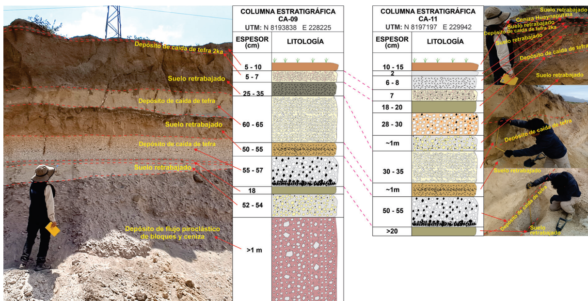
Figura 15. Columnas estratigráficas representativas (CA-09 y CA-11) de los depósitos de caída de tefra identificados en Alto Cayma, donde se reconocen niveles asociados a erupciones del volcán Misti.
