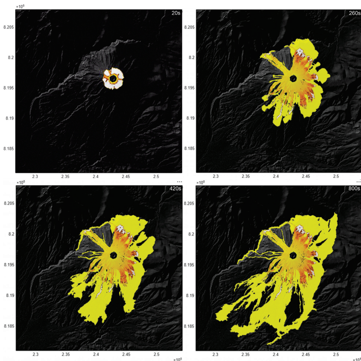
Figura 17. Proceso secuencial de simulación haciendo uso del código VolcFlow para los flujos piroclásticos del Misti.
