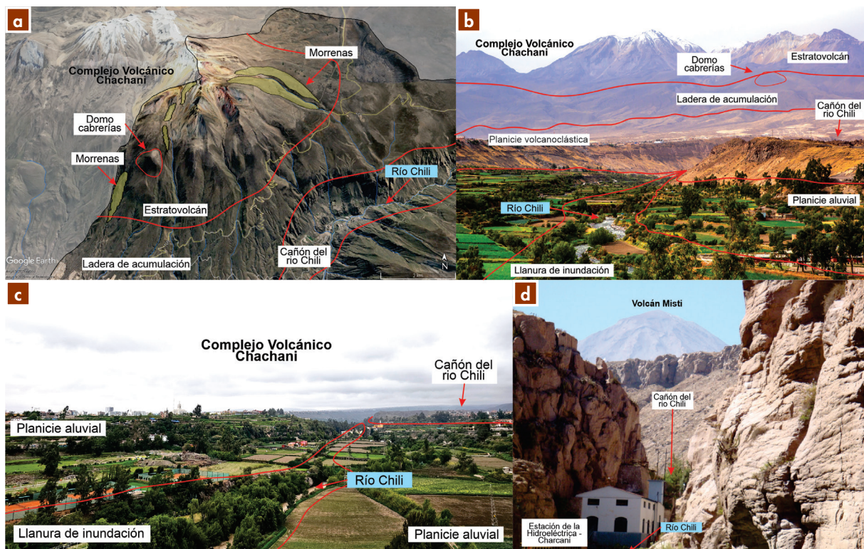
Figura 5. Unidades geomorfológicas presentes en el distrito de Cayma. a) Morrenas, domo Cabrerías, estratovolcán, laderas de acumulación y cañón del río Chili. b) Vista panorámica de las principales unidades geomorfológicas asociadas al volcán Chachani. c) Planicie aluvial y llanura de inundación desarrolladas a lo largo del río Chili. d) Cañón del río Chili y sectores del volcán Misti.
