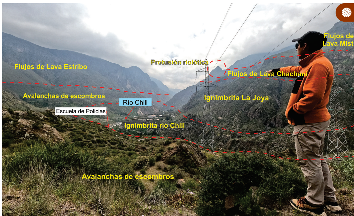
Figura 8. Vista del valle del río Chili, donde se observan la protrusión riolítica, las ignimbritas Río Chili y La Joya, avalanchas de escombros del Misti y flujos de lava.
