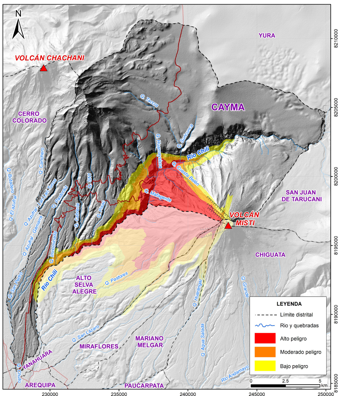
Figura 28. Mapa de peligros por avalancha de escombros en el distrito de Cayma.
