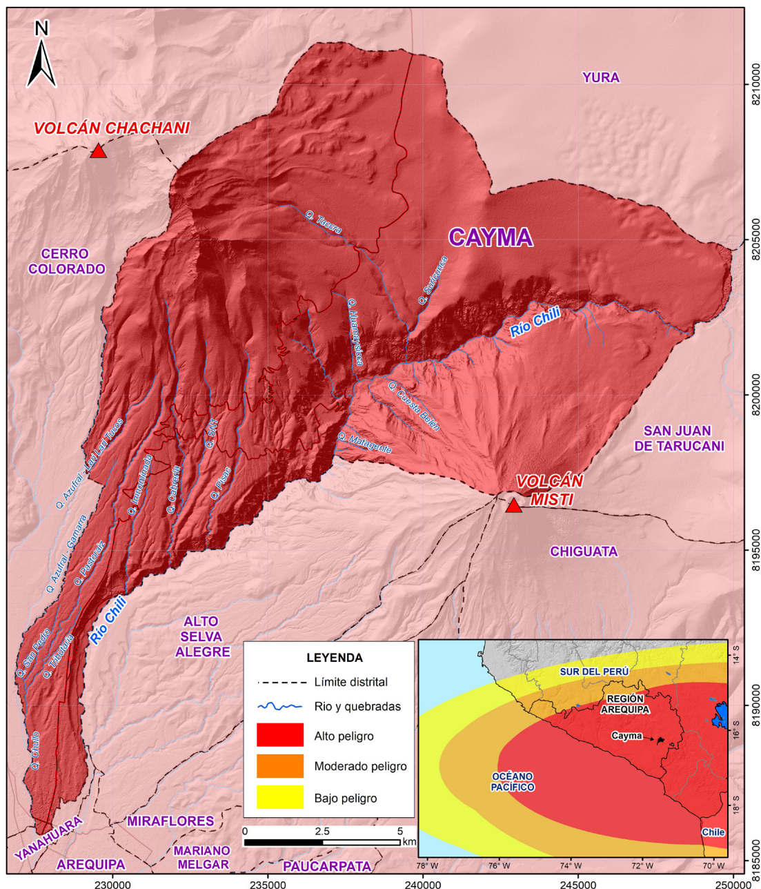
Figura 31. Mapa de peligro por caída de tefra para un escenario de erupción pliniana (IEV 5), modificado de Rivera et al. (2024).
