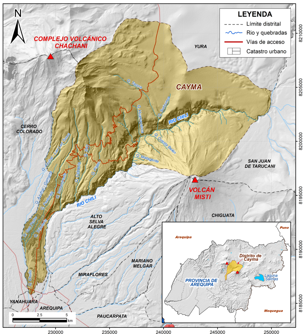
Figura 1. Ubicación geográfica y límites del distrito de Cayma.
