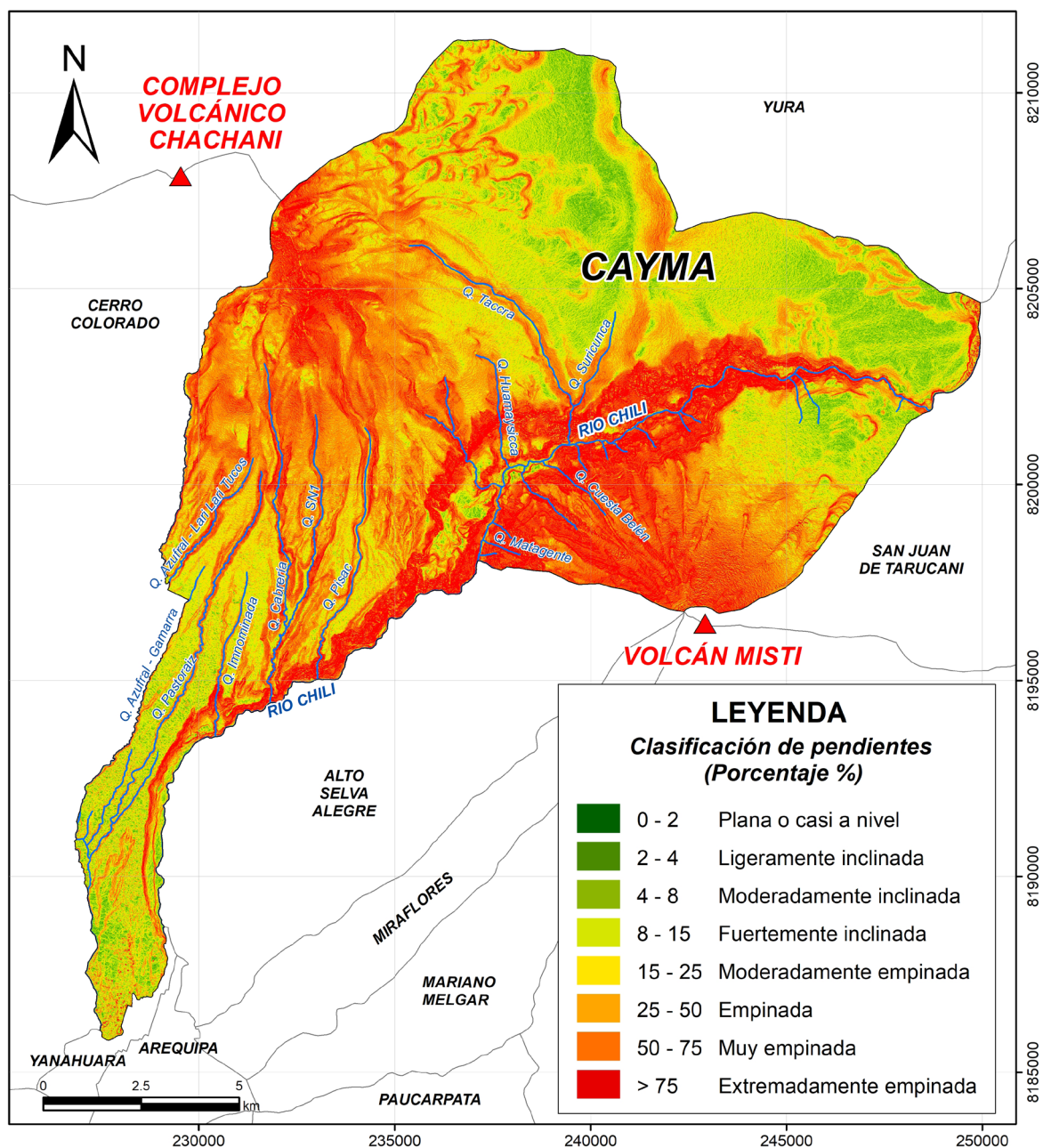
Figura 3. Mapa de pendientes del distrito de Cayma.
