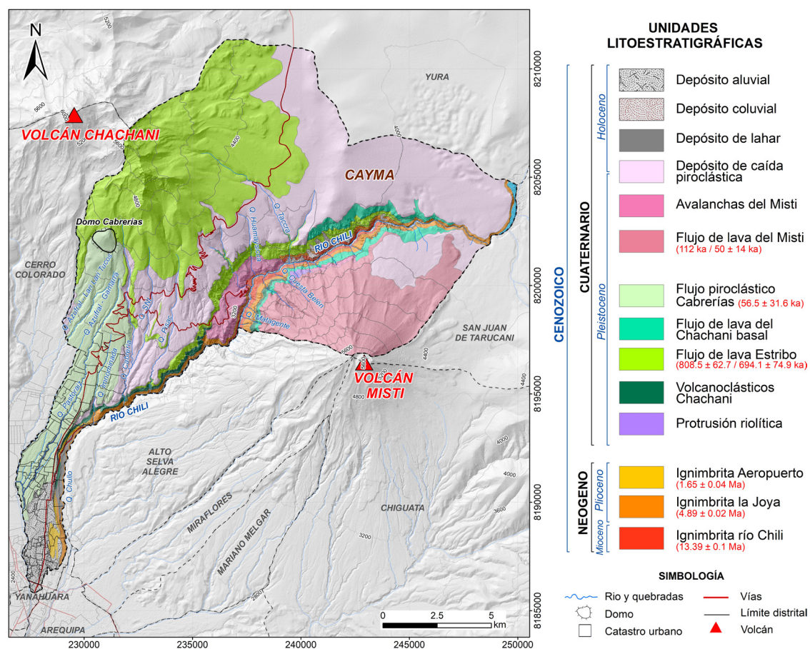
Figura 6. Mapa geológico del distrito de Cayma.
