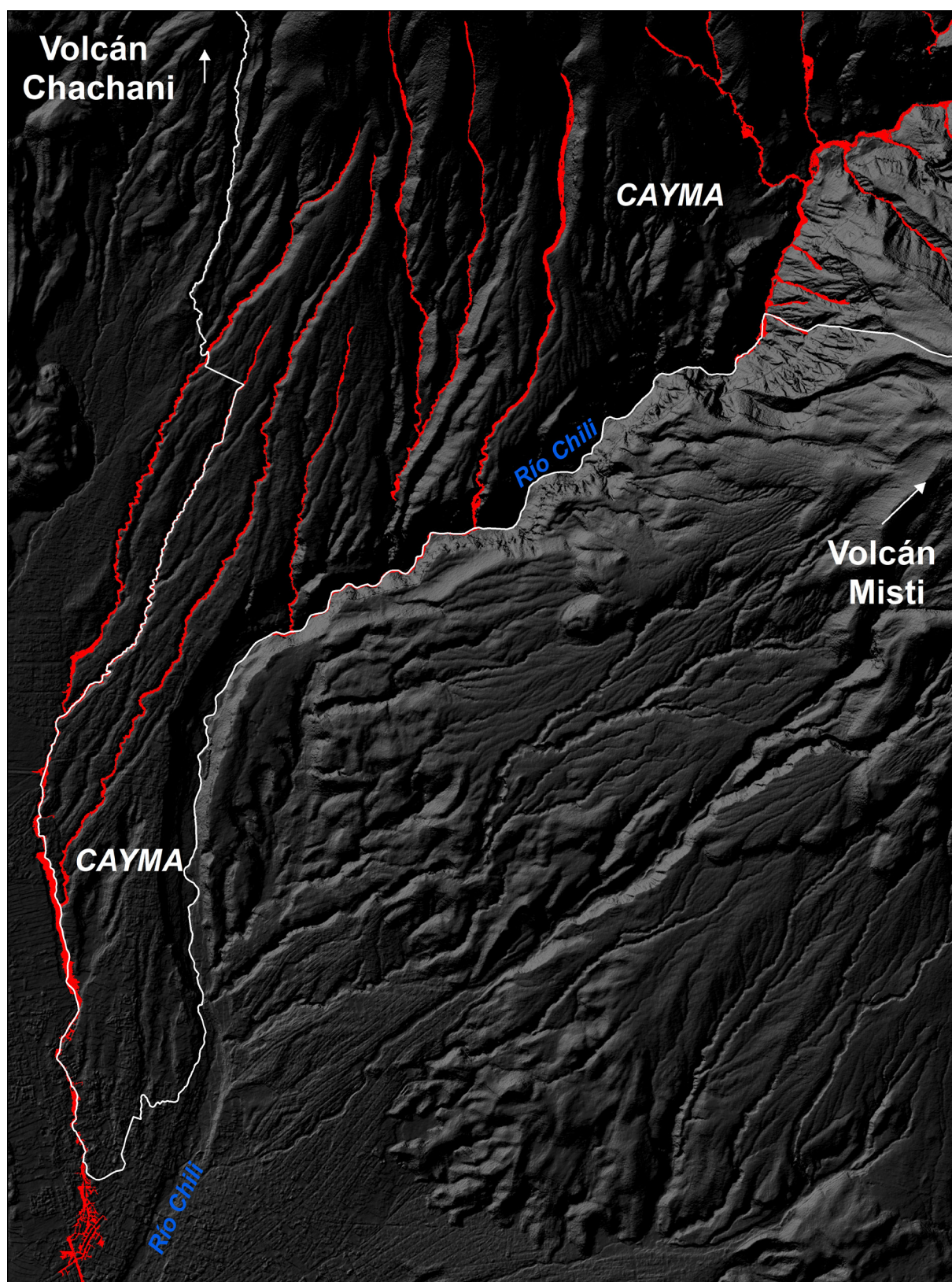
Figura 16. Resultado del modelamiento numérico de lahares.
