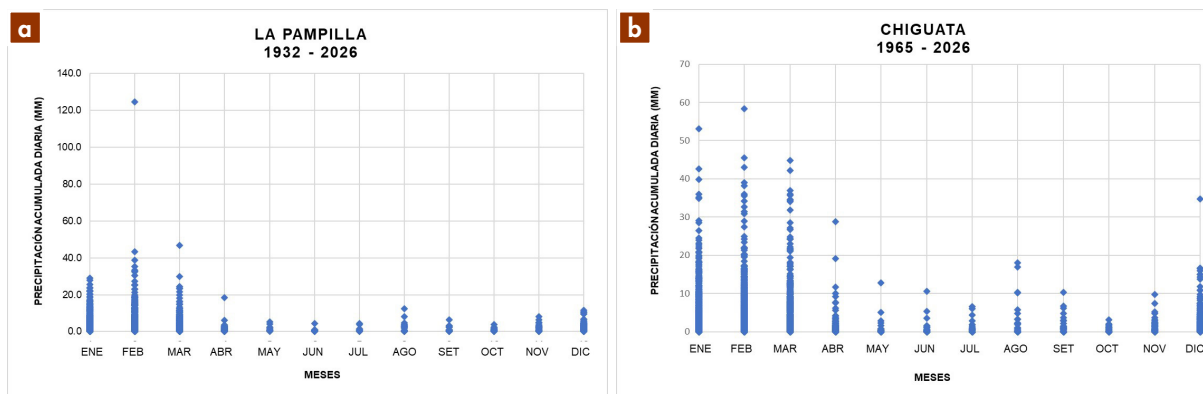
Figura 2. Precipitación acumulada diaria registrada en las estaciones meteorológicas La Pampilla (a) y Chiguata (b), utilizadas para la caracterización del régimen de precipitaciones en el área de estudio (modificado de Rivera et al., 2024).
