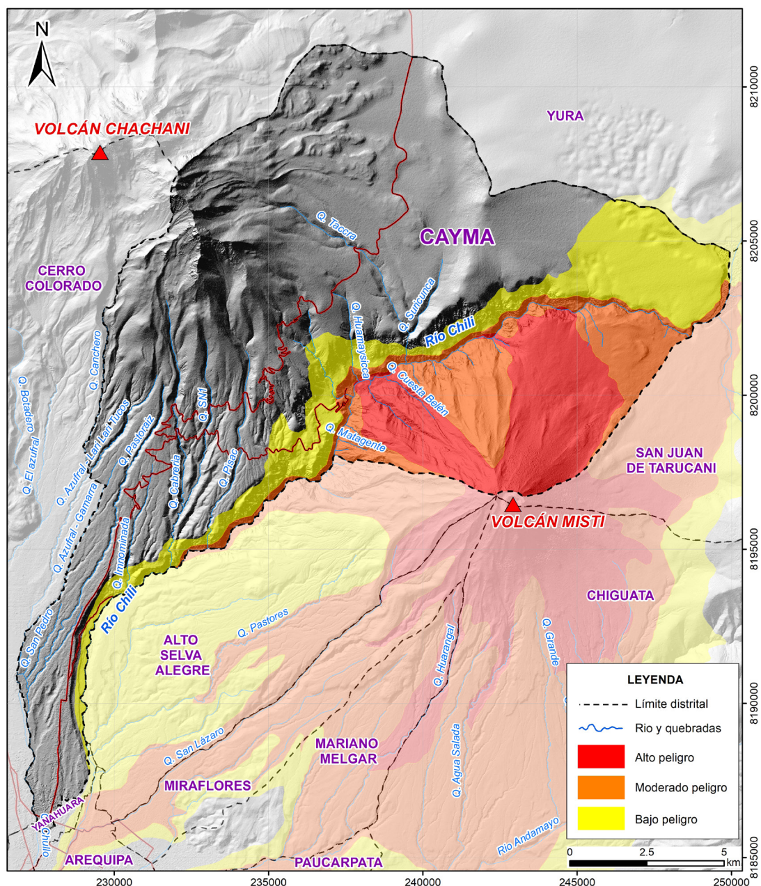
Figura 27. Mapa de peligro por descenso de flujos piroclásticos para el distrito de Cayma.
