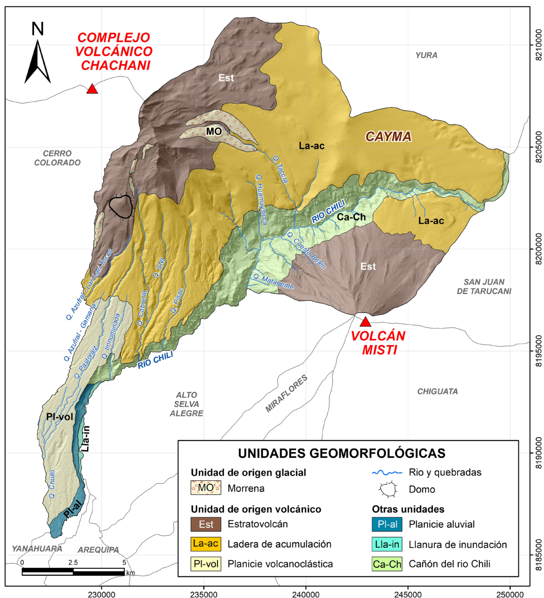
Figura 4. Mapa geomorfológico del distrito de Cayma.
