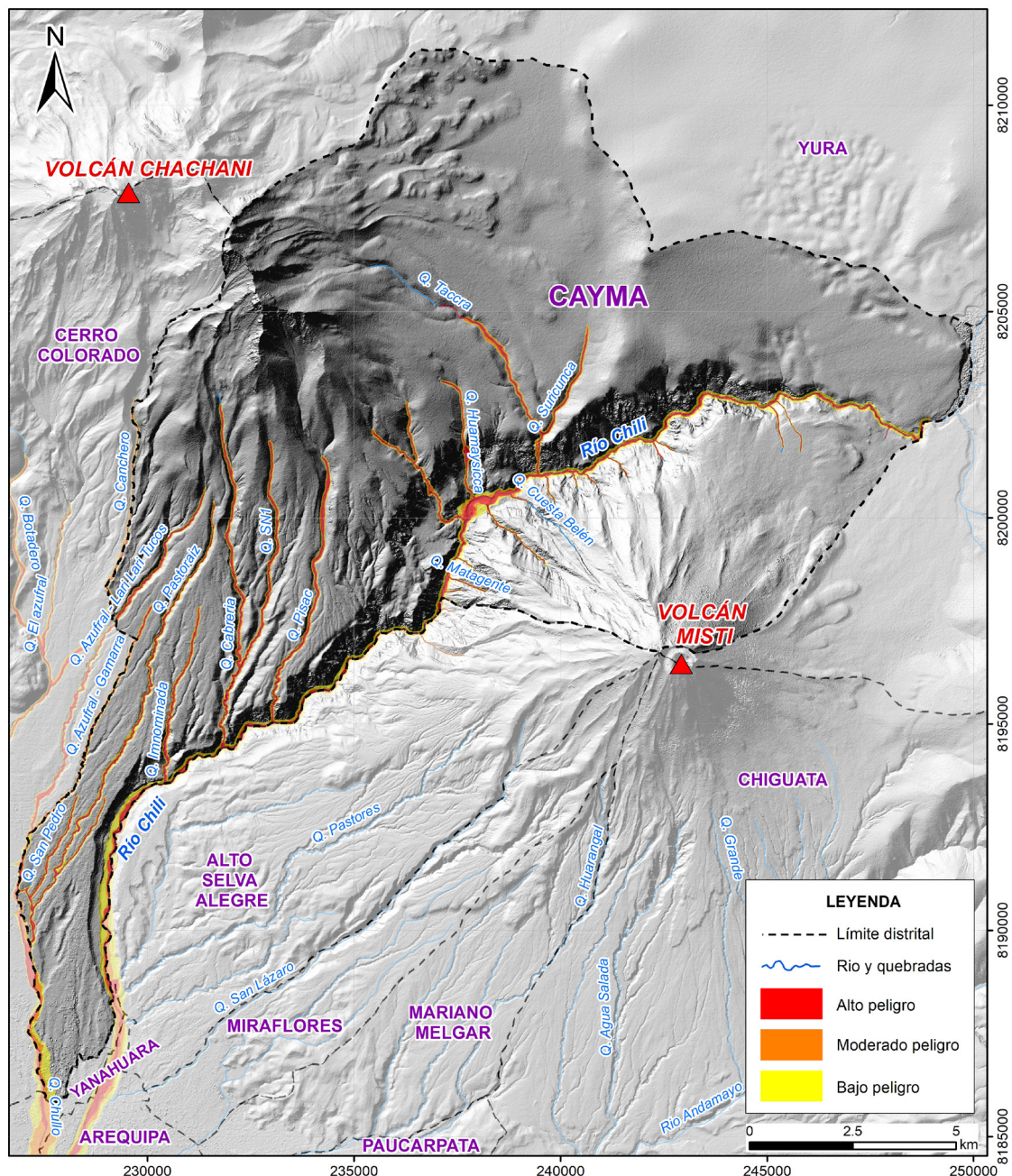
Figura 19. Mapa de peligro por descenso de lahares del distrito de Cayma.
