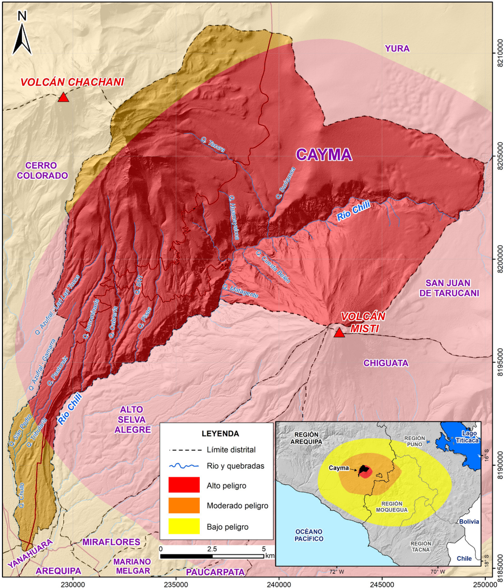
Figura 30. Mapa de peligro por caída de tefra para un escenario de erupción vulcaniana (IEV 1–2), modificado de Rivera et al. (2024).
