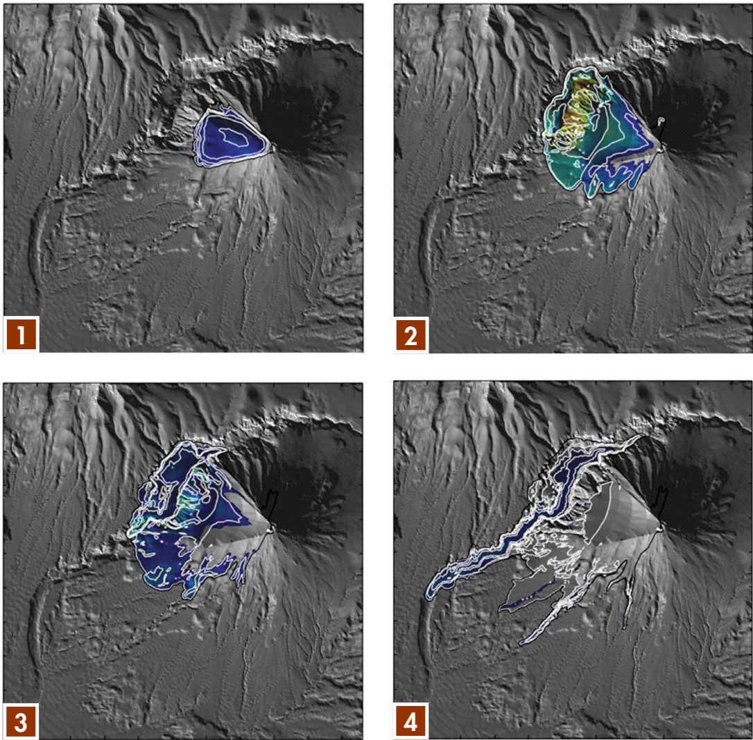
Figura 18. Proceso secuencial de simulación (1, 2, 3, 4) utilizando el código VolcFlow para las avalanchas de escombros en el sector oeste-suroeste del Misti.
