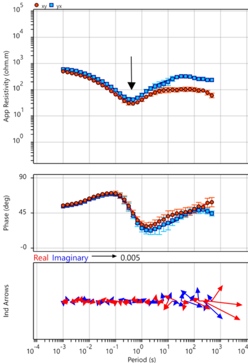
Figura 16. Los dos diagramas superiores representan las curvas de resistividad aparente y fase de la estación MT17, respectivamente. La flecha negra resalta el mínimo de resistividad de las dos polarizaciones xy e yx . El diagrama inferior muestra las variaciones de los vectores de inducción con el periodo.
