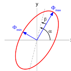
Figura 12. Representación gráfica del tensor de Fase. \phi_{max} y \phi_{min} corresponden al eje mayor y menor del elipsoide, respectivamente. \beta es el Skew y \alpha expresa la dependencia del tensor respecto al sistema de coordenadas.
