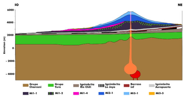
Figura 3. Corte geológico del volcán Misti, modificado de Cacya y Mamani (2009). Las abreviaciones Mi1, Mi2 y Mi3 corresponden a los edificios volcánicos Misti 1, Misti 2 y Misti 3, respectivamente.
