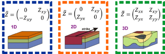
Figura 11. Representación gráfica sobre la dimensionalidad del medio y el tensor de impedancia asociado. Imagen extraída de Campanyà (2014).
