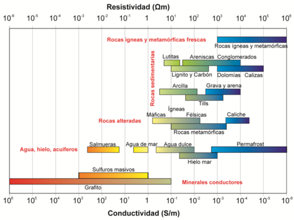
Figura 7. Rango de conductividad eléctrica de los materiales más frecuentes en la Tierra, modificado de Miensopust (2010).
