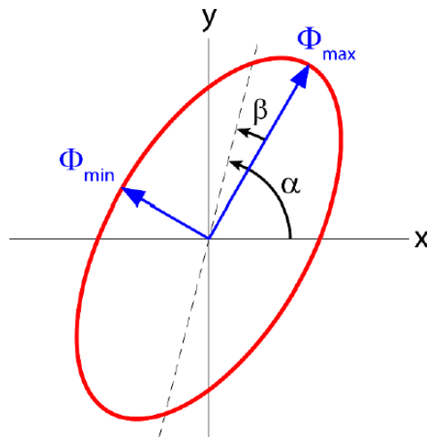
Figura 5.- Representación gráfica del tensor de fase. \varphi_{max} y \varphi_{min} corresponden al eje mayor y menor del elipsoide, respectivamente. \beta es el Skew y \alpha expresa la dependencia del tensor respecto al sistema de coordenadas (Caldwell et al., 2004).
