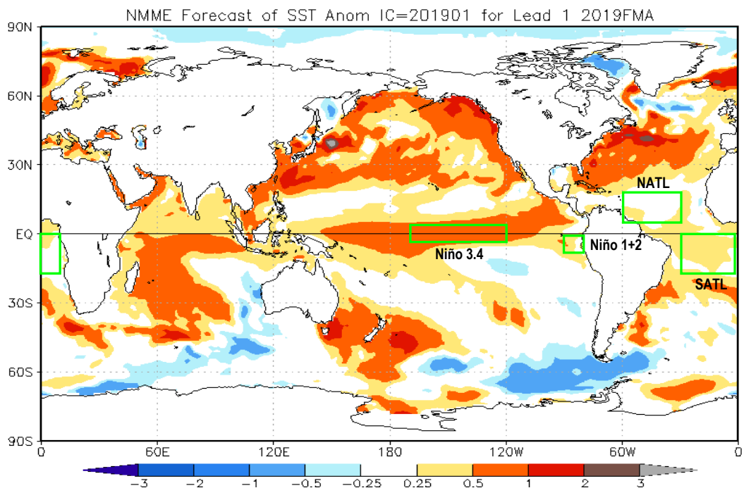
Fig. 7: Pronóstico de las anomalías de TSM (°C) a nivel global, para el trimestre febrero-abril 2019 (FMA). Rectángulos verdes indican regiones de análisis. Fuente: National Multi-Model Ensemble (NMME) .
