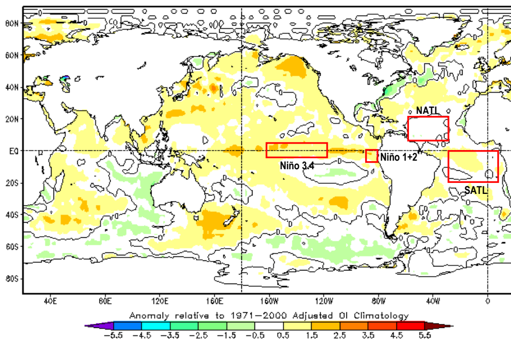
Fig. 1: Anomalías de temperatura superficial del mar (TSM) en °C del mes de diciembre de 2018. Las anomalías son calculadas utilizando la climatología del periodo base 1971-2000. Fuente CPTec/INPE/BRASIL.
