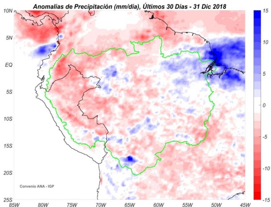
Fig. 4: Anomalías de precipitación estimadas por el TRMM-RT en mm/día hasta 31 de diciembre de 2018. Las anomalías fueron calculadas con respecto al periodo base promedio 2000-2017. Se muestra los límites de la cuenca Amazónica en líneas de color verde. Las anomalías de precipitación del TRMM-RT actualizadas a tiempo real puede verse en: http://intranet.igp.gob.pe/eventos-extremos-amazonia-peruana/ .
