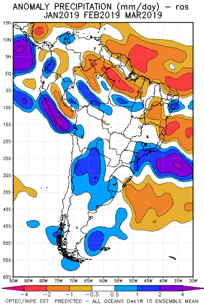
Fig. 10: Pronóstico de las anomalías de la precipitación (mm/día) método ras para el trimestre EFM del 2019 en América del Sur, con datos observados de fines del mes de diciembre de 2018. Fuente: CPTEC/INPE.
