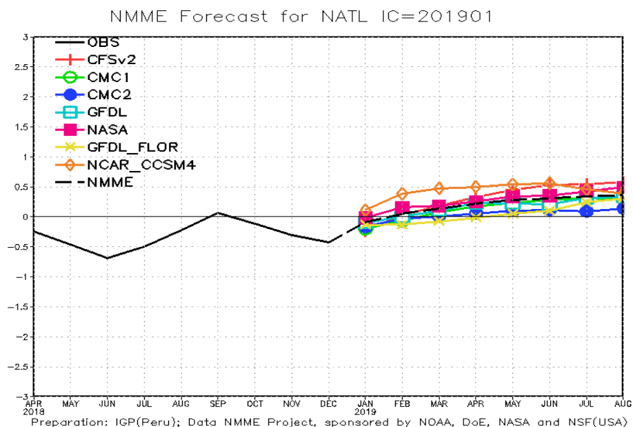
Fig. 9: Pronóstico de las anomalías de temperatura superficial del mar (TSM) para la región del Atlántico tropical Norte (NATL: 5°N-20°N, 30°W-60°W), a partir de condiciones de fines de diciembre 2018. Fuente: Instituto Geofísico del Perú (IGP) .
