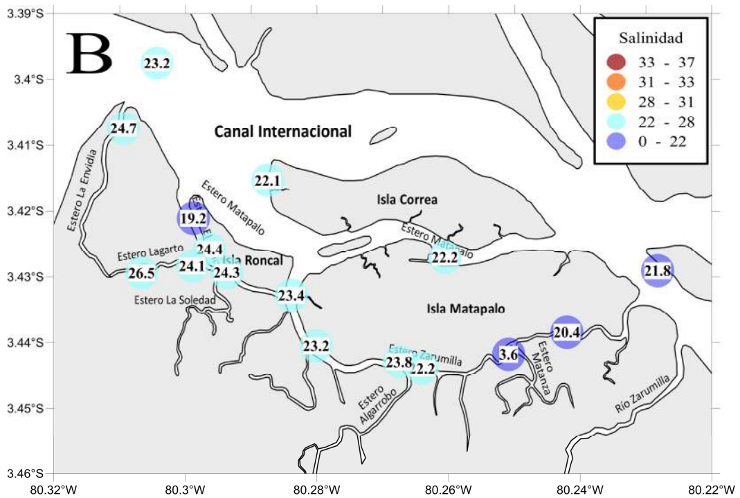
Figura 13. Salinidad en columna de agua para las estaciones de muestreo dentro del SNLMT. A. Septiembre 2012, B. Abril 2013.
