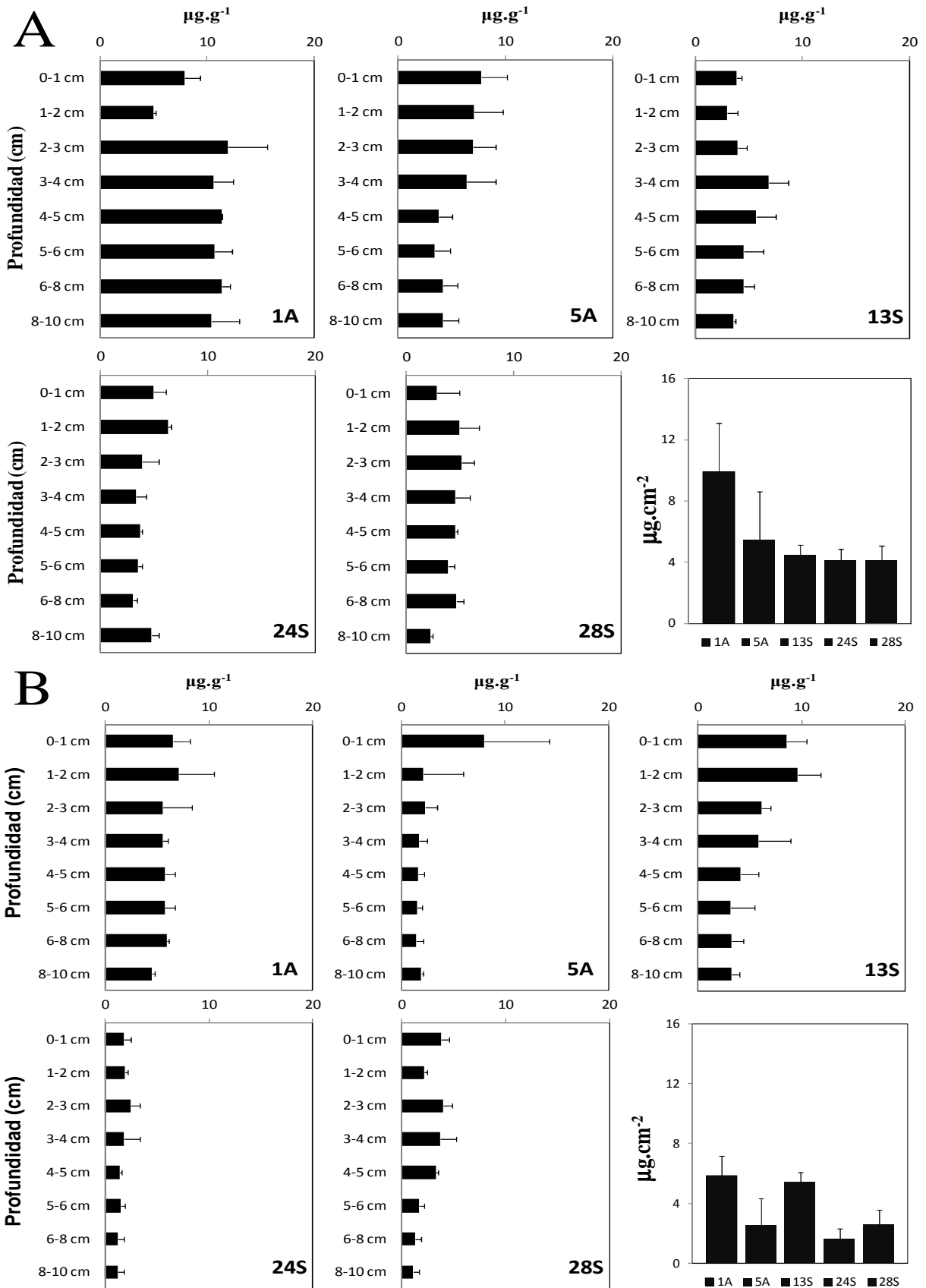
F2. Distribución vertical de la concentración de feopigmentos ( \mu\text{g}\cdot\text{g}^{-1} ) \pm SD en la columna de sedimento para las estaciones de muestreo dentro del SNLMT. A. Septiembre 2012, B. Abril 2013
