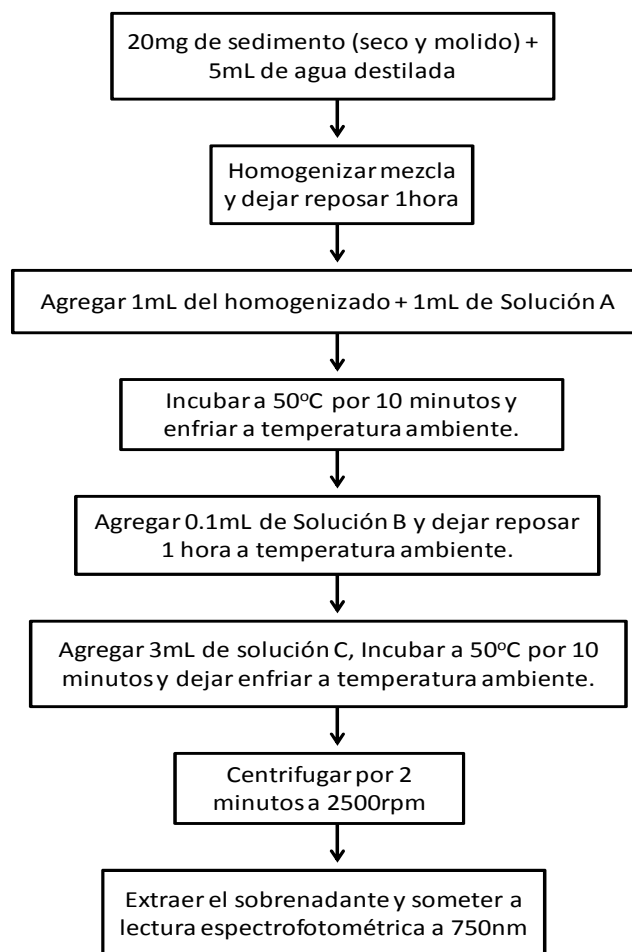
Figura 9. Cuadro de flujo para la determinación del contenido de proteínas totales en sedimento, modificado de (Lowry et al. 1951) y Rice (1982).
