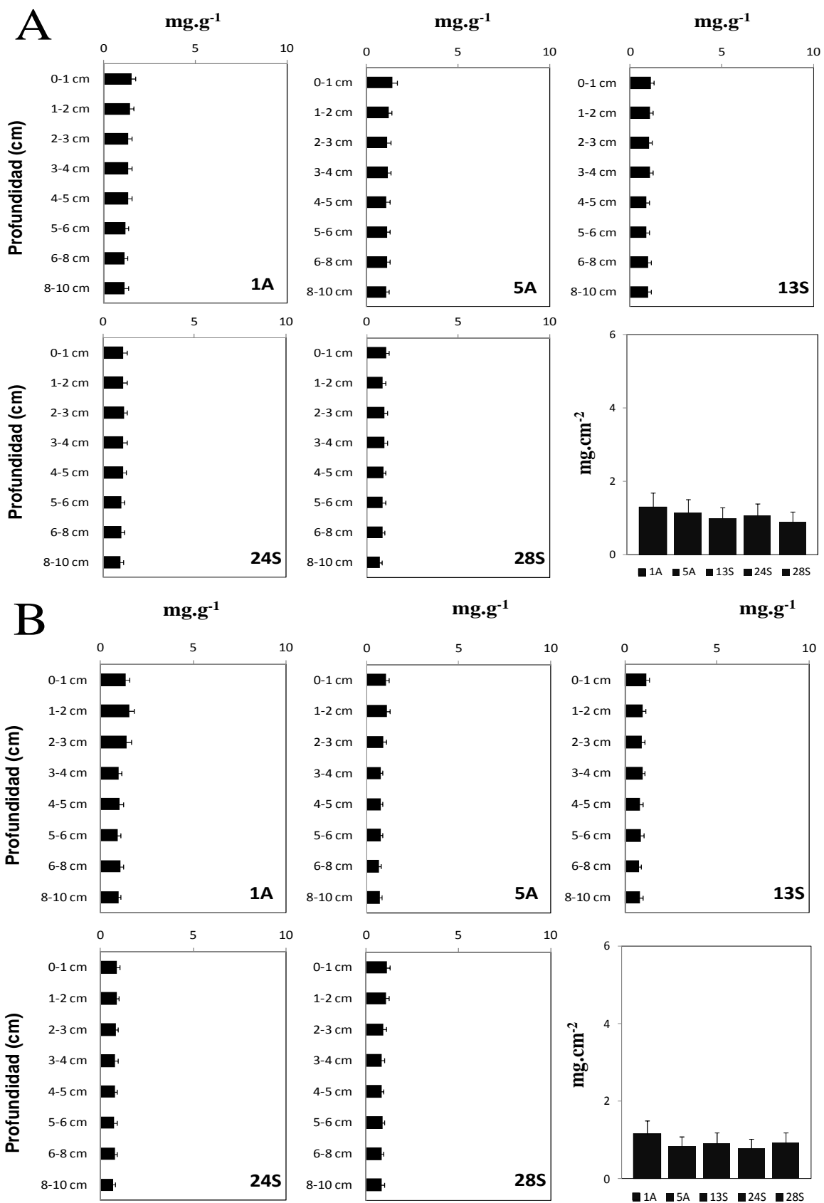
F4. Distribución vertical de la concentración de CHO ( \text{mg}\cdot\text{g}^{-1} ) \pm SD en la columna de sedimento para las estaciones de muestreo dentro del SNLMT. A. Septiembre 2012, B. Abril 2013.
