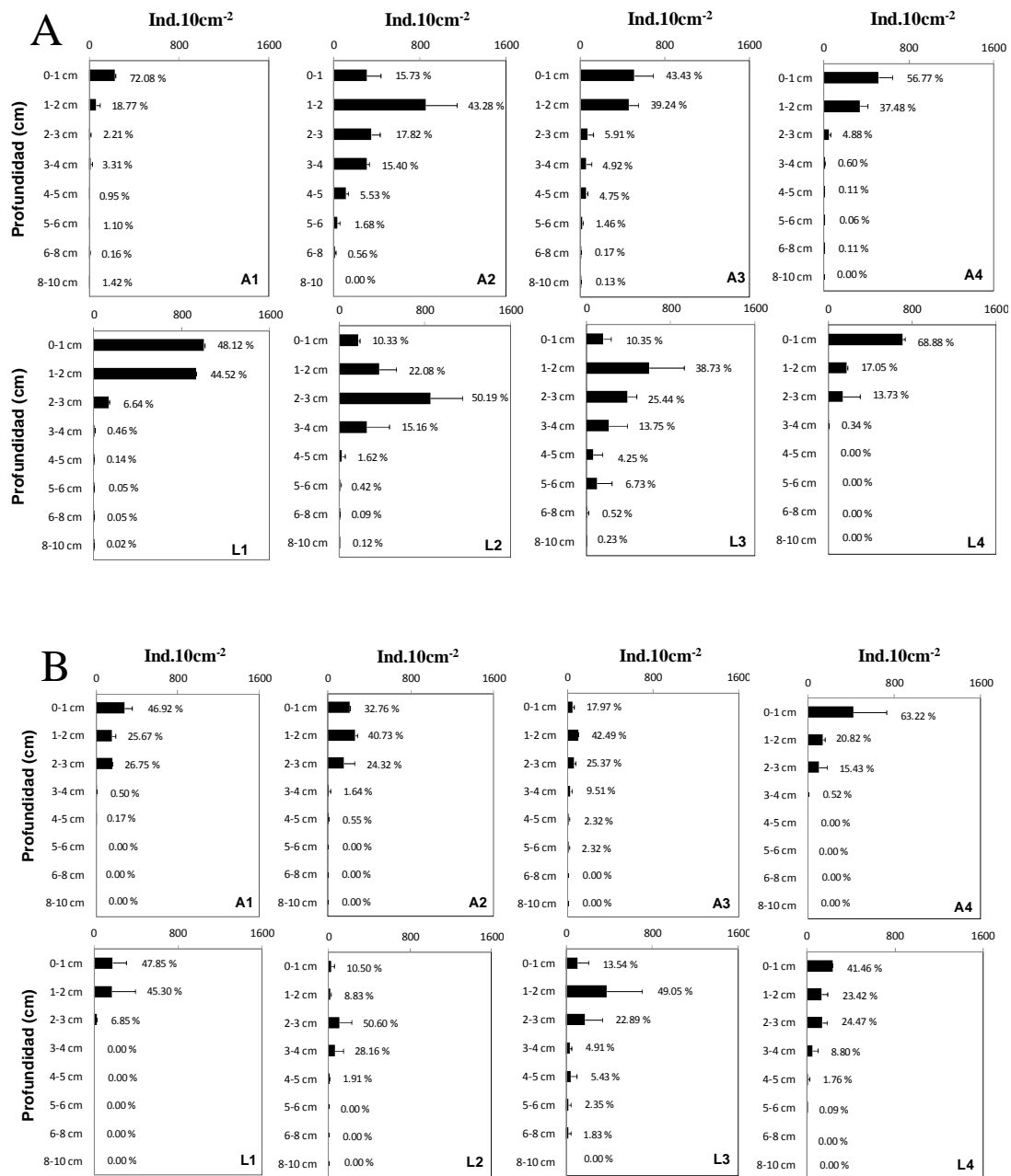
Figura 34. Concentración espacio-vertical de la abundancia del meiobentos ( Ind.10cm^{-2} ) \pm SD en la columna de sedimento para las estaciones dos estaciones de muestreo dentro del SNLMT. A. Noviembre 2012, B. Abril 2013. A: Algarrobo. L: Lagarto. 1: marea baja. 2: marea llenante. 3 marea alta. 4: marea vaciante. S: número de taxones ( Tax.10cm^{-2} ).
