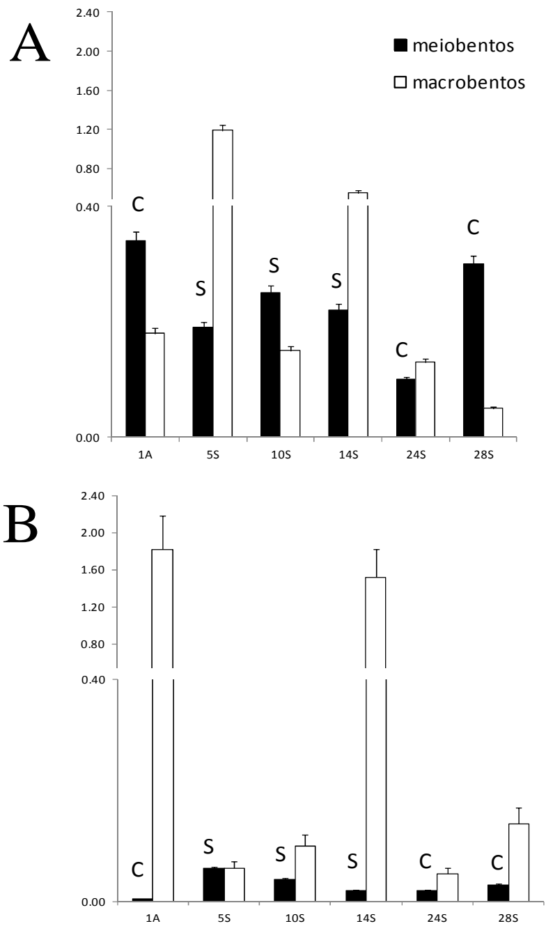
Figura 26. Biomasa del meiobentos Vs. biomasa del macrobentos (gC.m -2 ) para las seis estaciones de muestreo dentro del SNLMT. A. Septiembre 2012, B. Abril 2013. C: columna (0-10cm.). S: superficie (0-1cm).
