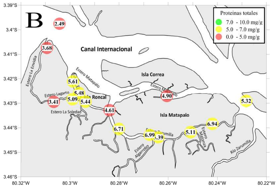
Figura 21. Concentración de PRTt en sedimento superficial (0-1cm) para las estaciones de muestreo dentro del SNLMT. A. Septiembre 2012, B. Abril 2013.
