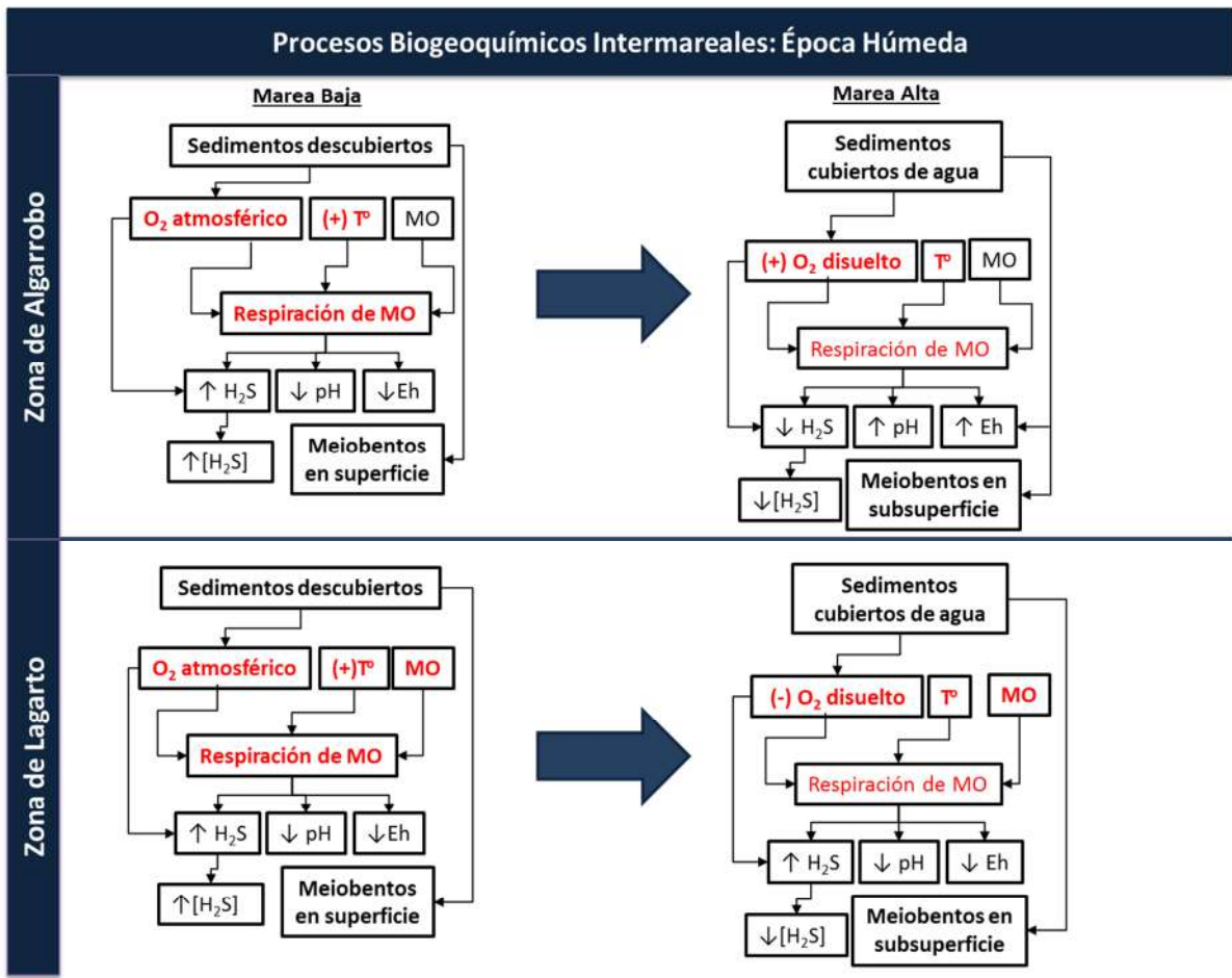
Figura 39. Diagrama conceptual que resume los procesos biogeoquímicos que afectan al ambiente sedimentario y a las comunidades meiobentónicas intermareales durante la época húmeda en el SNLMT.
