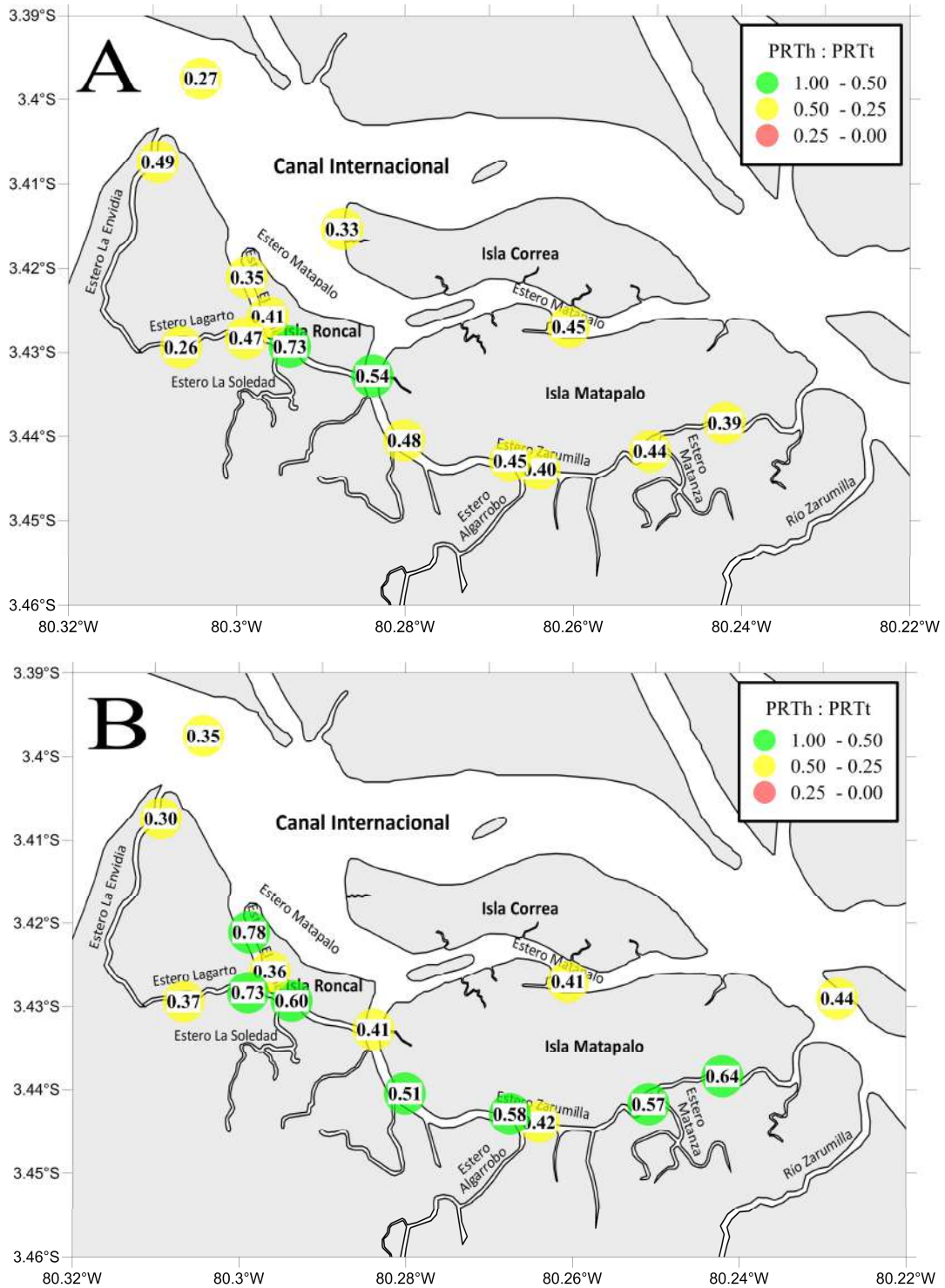
Figura 23. Cociente PR_{Th} : PR_{Tt} en sedimento superficial (0-1cm) para las estaciones de muestreo dentro del SNLMT. A. Septiembre 2012, B. Abril 2013.
