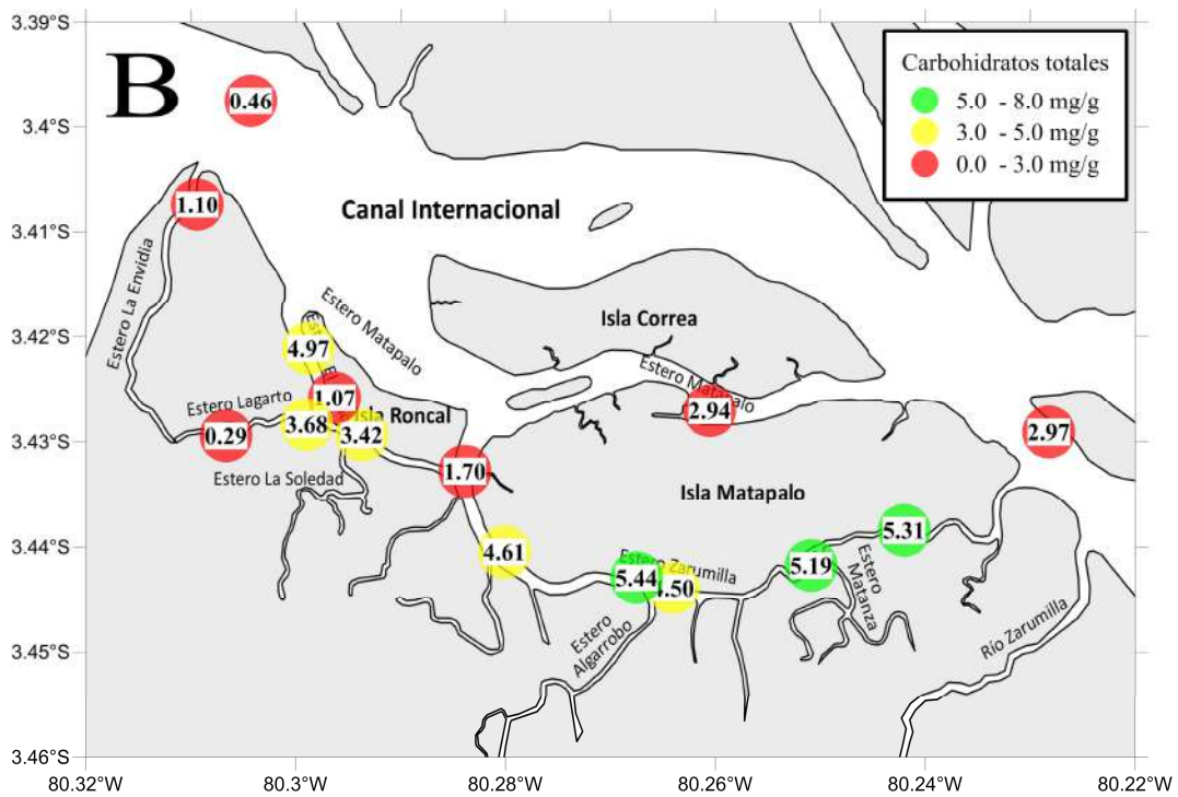
Figura 20. Concentración de CHOt en sedimento superficial (0-1cm) para las estaciones de muestreo dentro del SNLMT. A. Septiembre 2012, B. Abril 2013.
