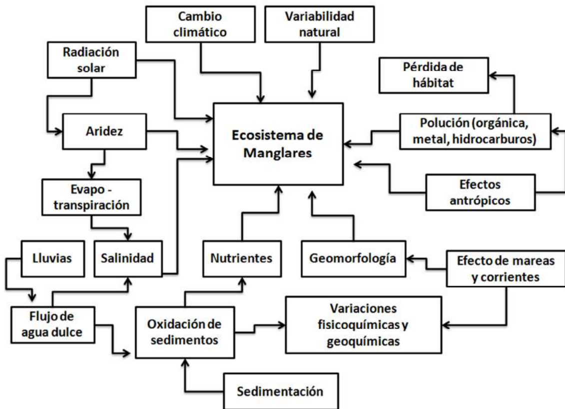
Figura 1. Factores físicos, químicos y antrópicos que impactan sobre los ecosistemas de manglares (Modificado de Kathiresan y Bingham, 2001).
