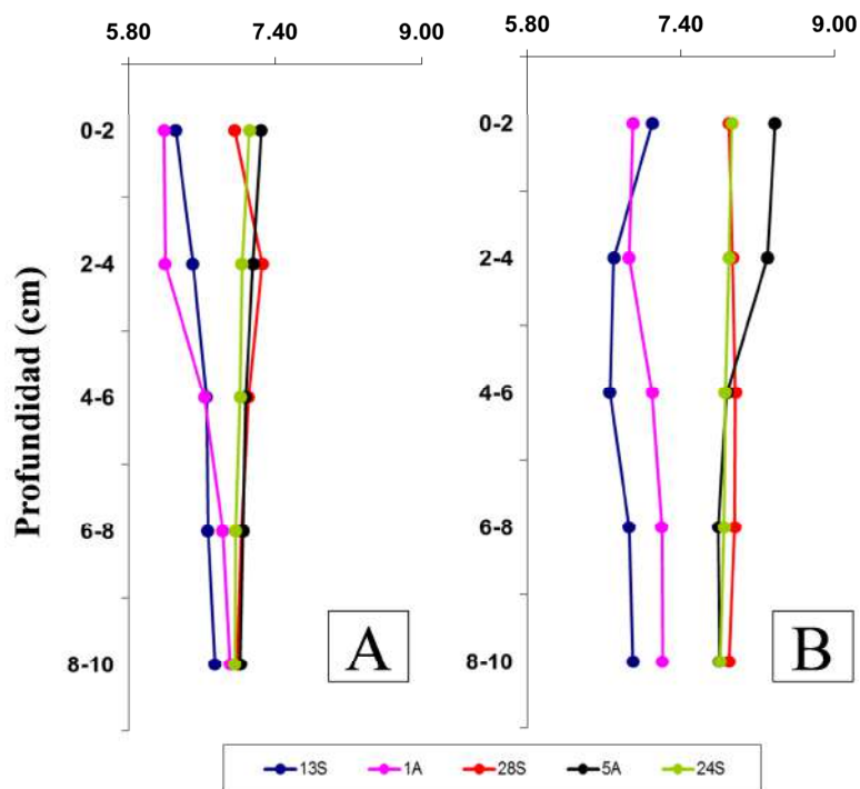
Figura 17. Perfiles verticales de pH en la columna de sedimento (0-10cm.) para las cinco estaciones de muestreo dentro del SNLMT. A. Septiembre 2012, B. Abril 2013.
