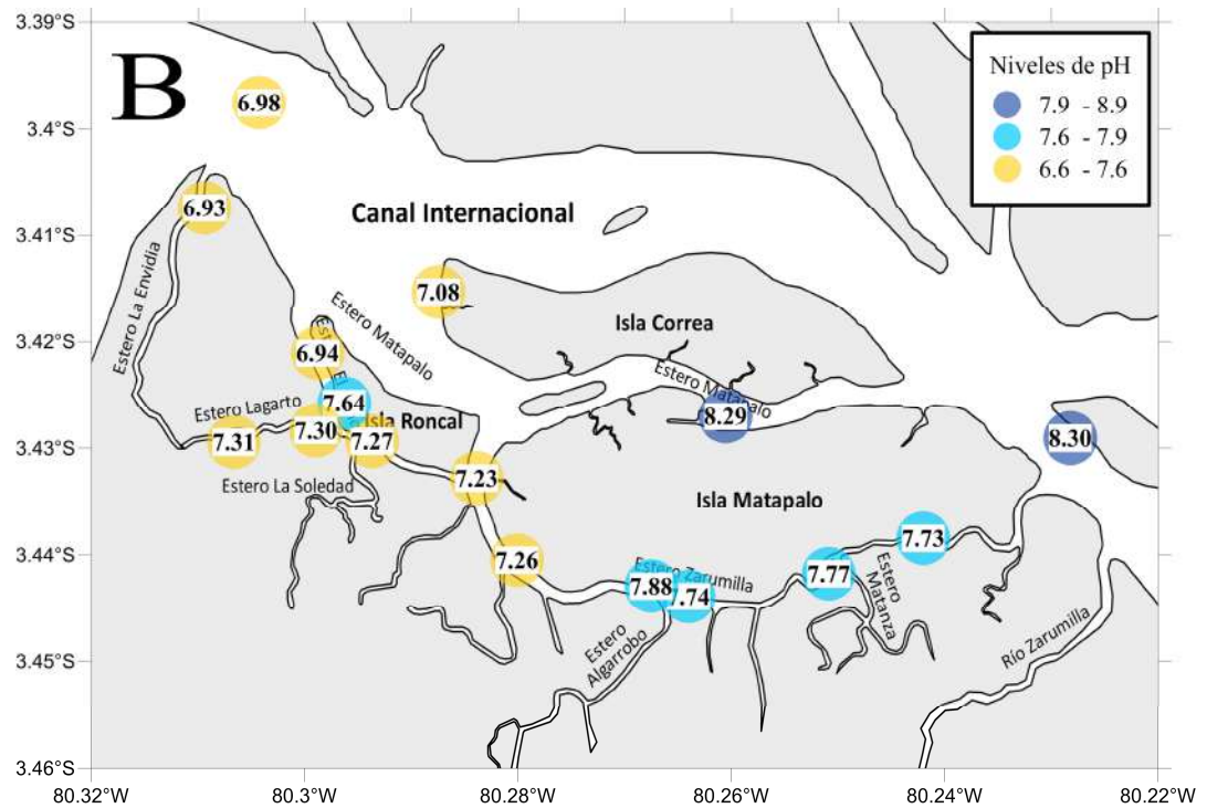
Figura 15. Niveles de pH en columna de agua para las estaciones de muestreo dentro del SNLMT. A. Septiembre 2012, B. Abril 2013.
