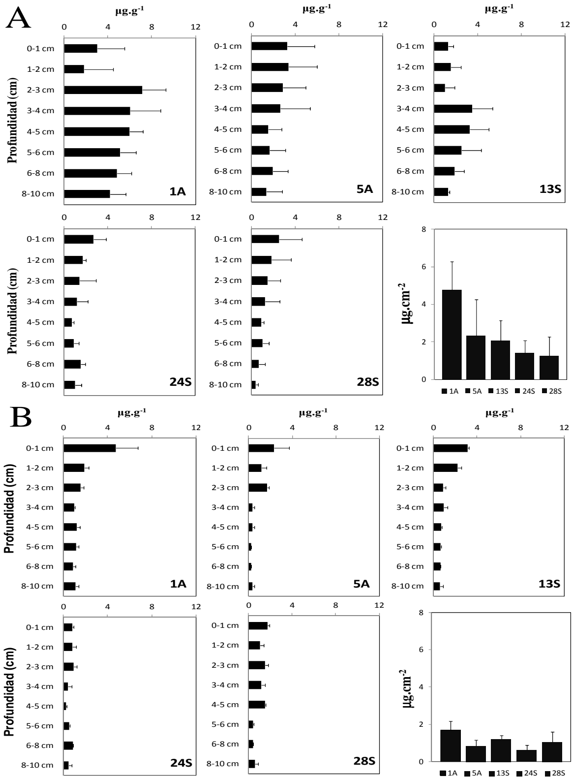
F1. Distribución espacio-vertical de la concentración de Cl-a ( \mu\text{g}\cdot\text{g}^{-1} ) \pm SD en la columna de sedimento para las estaciones de muestreo dentro del SNLMT. A. Septiembre 2012, B. Abril 2013.
