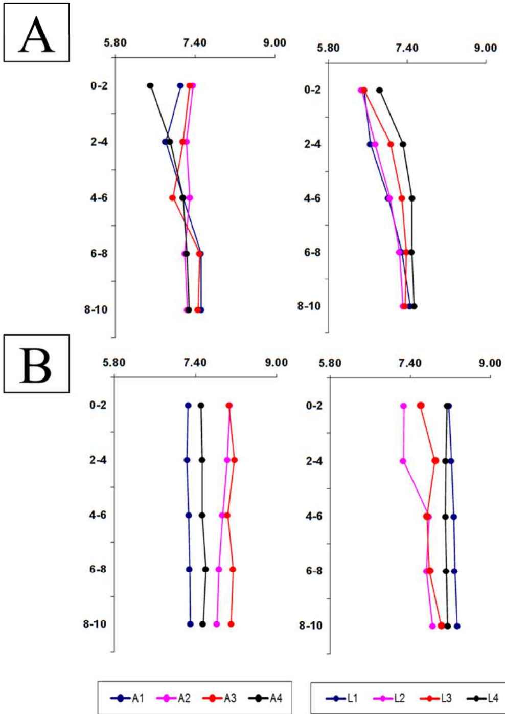
Figura 31. Registros de pH en la columna de sedimento (0-10cm.) para las dos estaciones de muestreo dentro del SNLMT. A. Noviembre 2012, B. Abril 2013. A: Algarrobo. L: Lagarto. 1: marea baja. 2: marea llenante. 3 marea alta. 4: marea vaciante.
