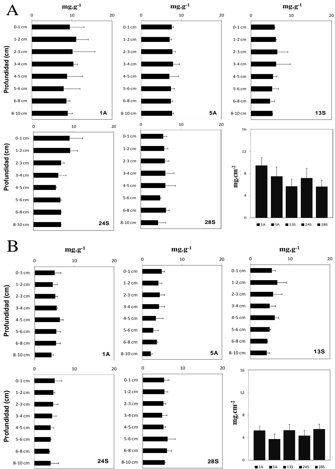
F5. Distribución vertical de la concentración de PRTt ( \text{mg.g}^{-1} ) \pm SD en la columna de sedimento para las estaciones de muestreo dentro del SNLMT. A. Septiembre 2012, B. Abril 2013.
