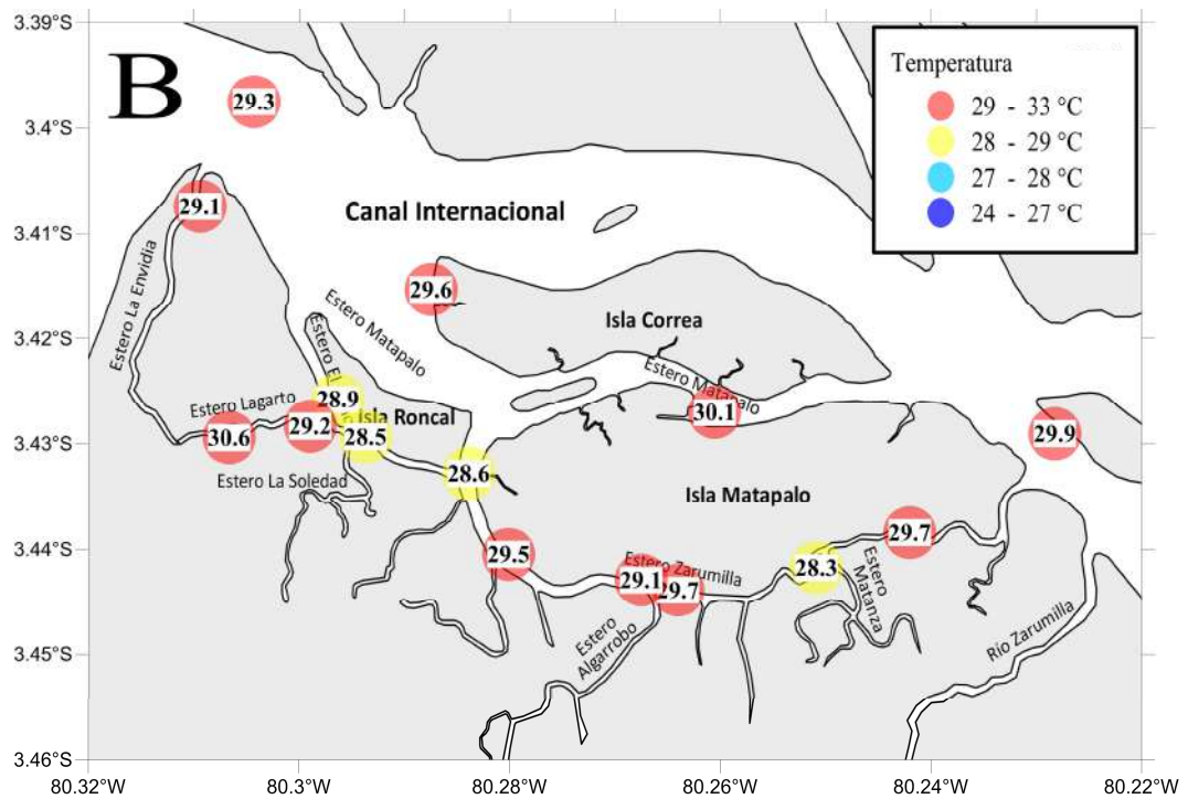
Figura 12. Temperatura en columna de agua para las estaciones de muestreo dentro del SNLMT. A. Septiembre 2012, B. Abril 2013.
