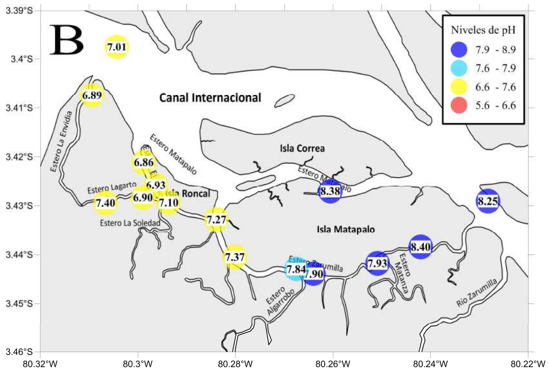
Figura 16. Niveles de pH en sedimento superficial (0-2cm.) para las estaciones de muestreo dentro del SNLMT. A. Septiembre 2012, B. Abril 2013.
