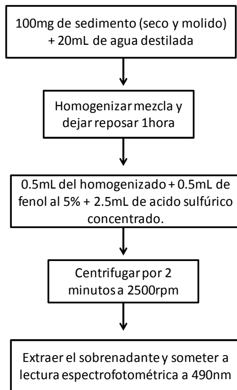
Figura 8. Cuadro de flujo para la determinación del contenido de carbohidratos totales en sedimento, modificado de Dubois et al. (1956).
