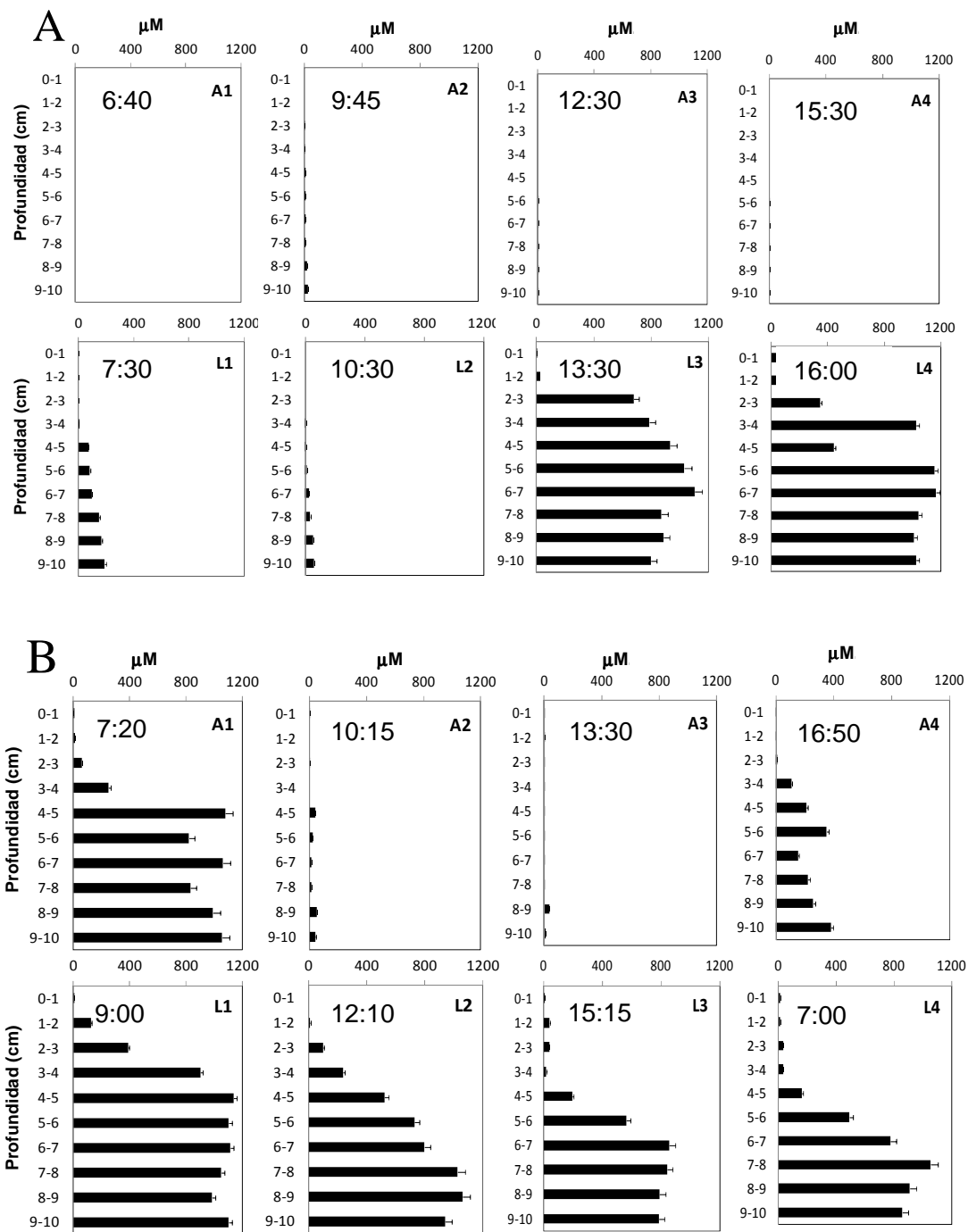
Figura 33. Concentración de sulfuro de hidrógeno ( \mu\text{M} ) en la columna de sedimento para las dos estaciones de muestreo en el SNLMT. A. Septiembre 2012, B. Abril 2013. A: Algarrobo. L: Lagarto. 1: marea baja. 2: marea llenante. 3 marea alta. 4: marea vaciante.
