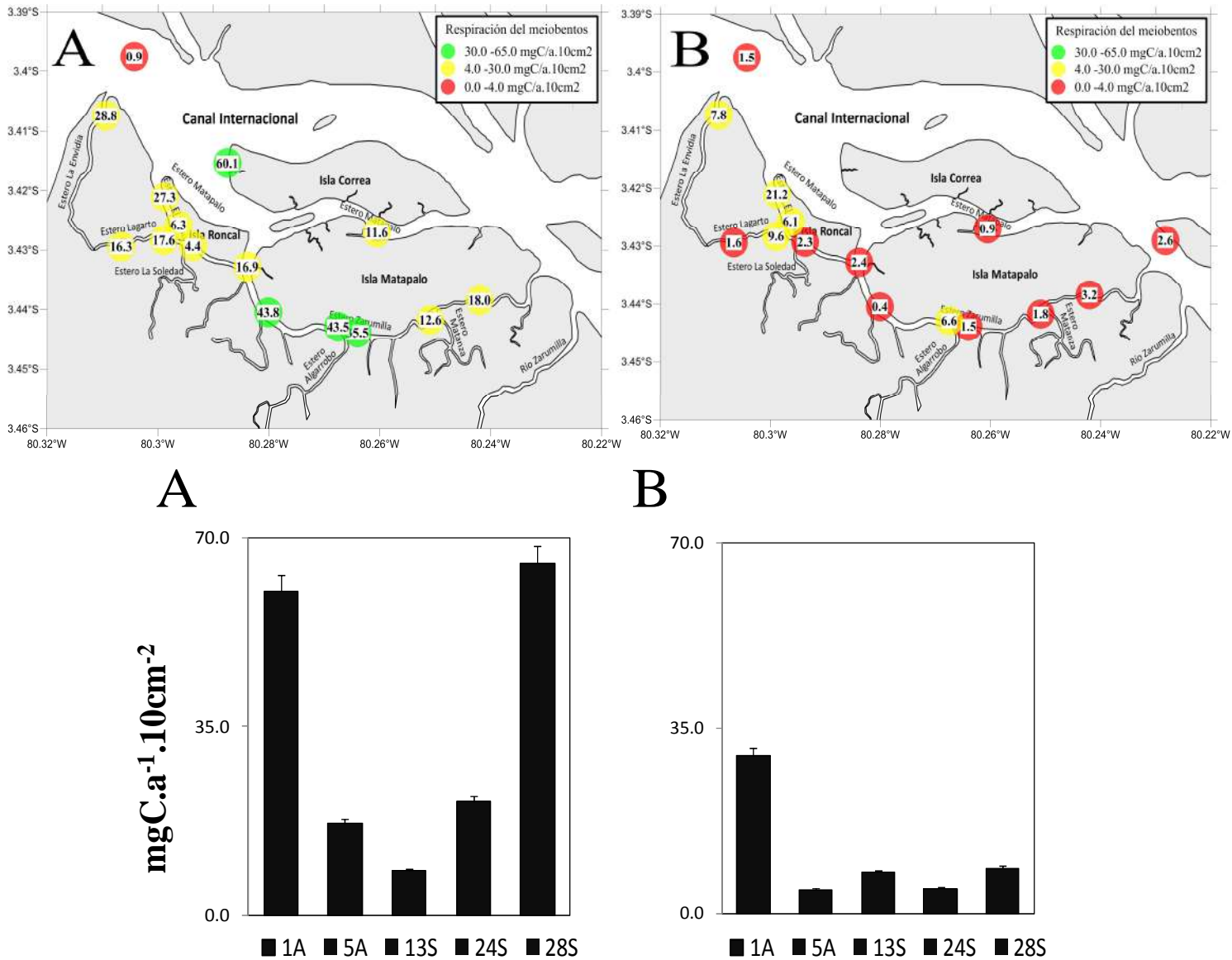
Figura 28. Distribución espacial (arriba) e integrada (abajo) de la respiración del meiobentos en la columna de sedimento (mgC.a -1 .10cm -2 ) ± SD para las estaciones de muestreo dentro del SNLMT. A. Septiembre 2012, B. Abril 2013.
