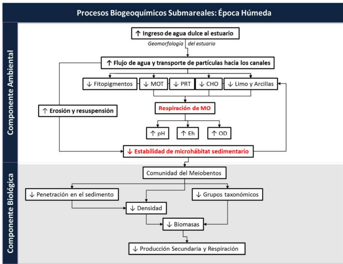
Figura 37. Diagrama conceptual que resume los procesos biogeoquímicos que afectan al ambiente sedimentario y a las comunidades meiobentónicas submareales durante la época húmeda en el SNLMT.
