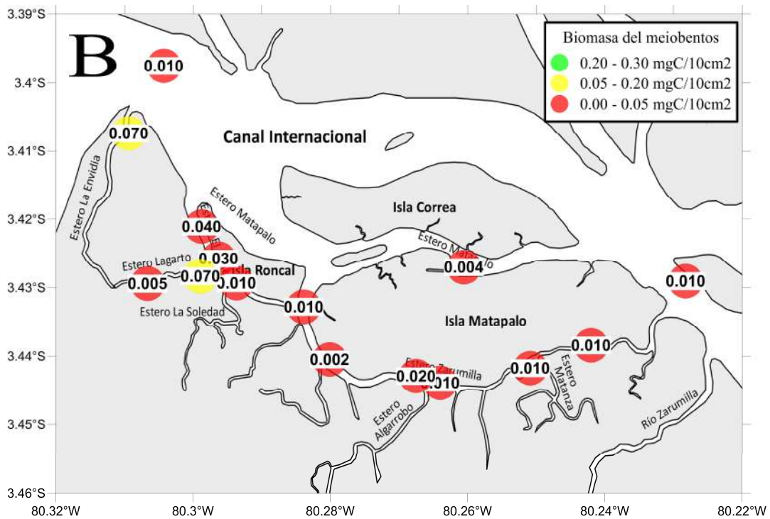
Figura 24. Biomasa del meiobentos (mgC.10cm -2 ) en sedimento superficial (0-1cm) para las estaciones de muestreo dentro del SNLMT. A. Septiembre 2012, B. Abril 2013.
