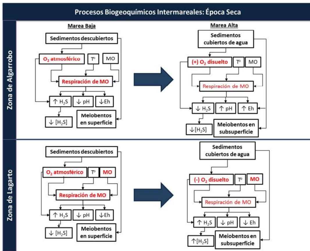
Figura 38. Diagrama conceptual que resume los procesos biogeoquímicos que afectan al ambiente sedimentario y a las comunidades meiobentónicas intermareales durante la época seca en el SNLMT.
