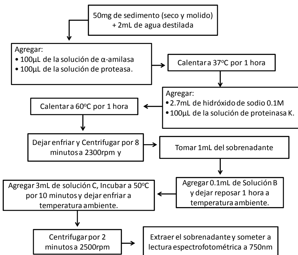
Figura 11. Cuadro de flujo para la determinación del contenido de proteínas hidrolizables en sedimento, modificado de Lowry (1956) y Mayer et al. (1986).
