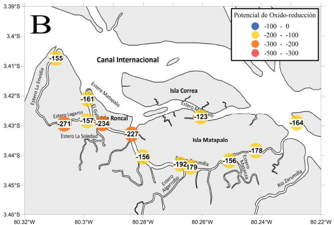
Figura 18. Potencial de óxido-reducción en sedimento superficial (0-2cm.) para las estaciones de muestreo dentro del SNLMT. A. Septiembre 2012, B. Abril 2013.
