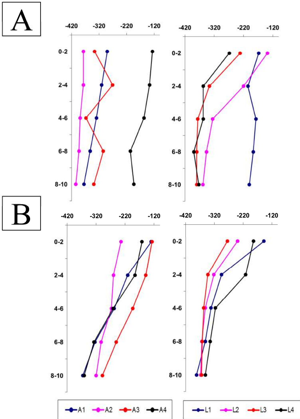
Figura 32. Valores de potencial de óxido-reducción (Eh) en mV para la columna de sedimento (0-10cm.) para las dos estaciones de muestreo dentro del SNLMT. A. Noviembre 2012, B. Abril 2013. A: Algarrobo. L: Lagarto. 1: marea baja. 2: marea llenante. 3 marea alta. 4: marea vaciante.
