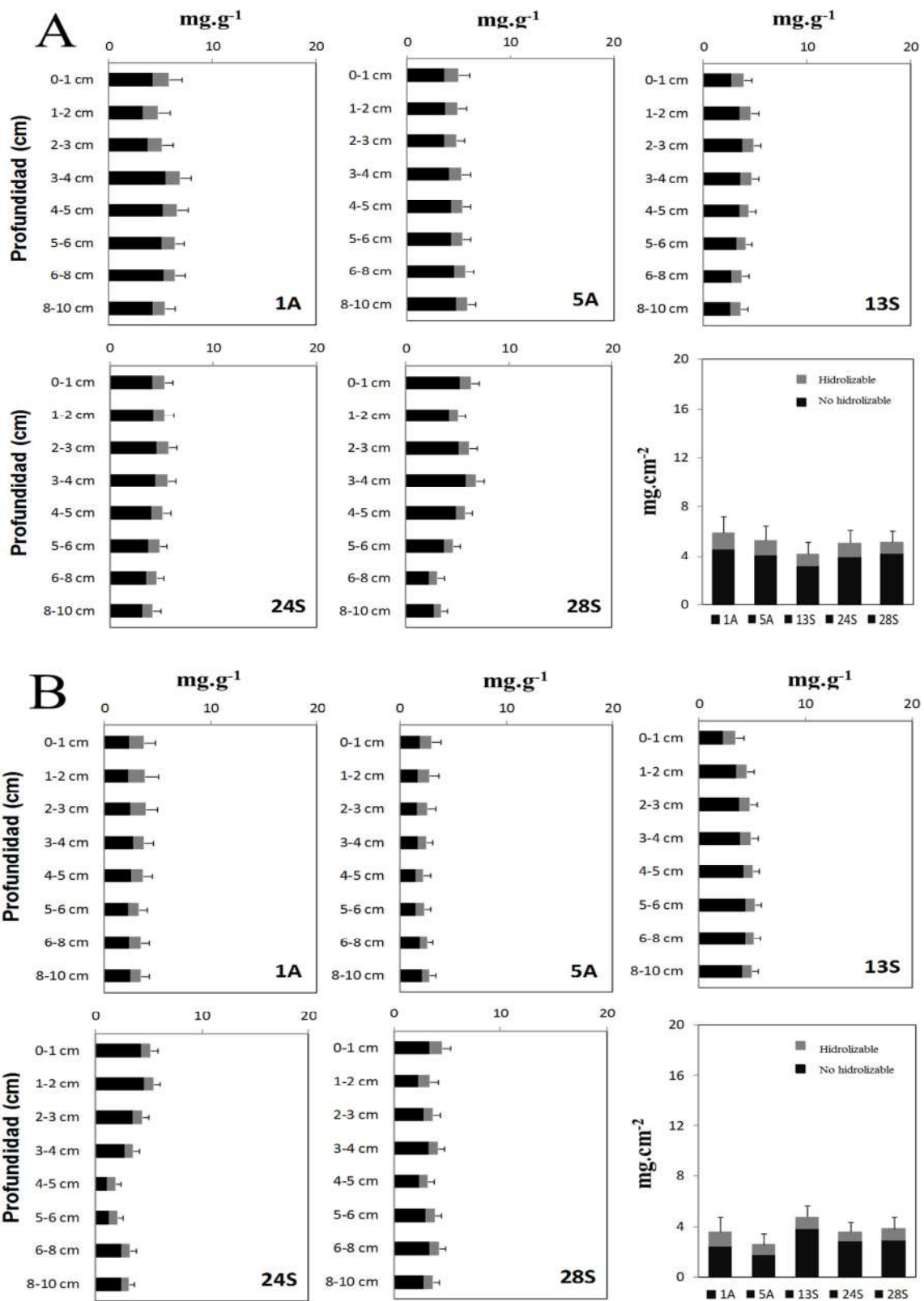
F7. Distribución vertical de las concentraciones hidrolizables y no hidrolizables de CHO ( \text{mg}\cdot\text{g}^{-1} ) \pm SD en la columna de sedimento para las estaciones de muestreo dentro del SNLMT. A. Septiembre 2012, B. Abril 2013.
