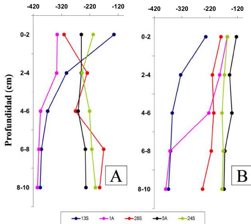
Figura 19. Perfiles verticales de potencial de óxido-reducción (mV) en columna de sedimento (0-10cm.) para las cinco estaciones de muestreo dentro del SNLMT. A. Septiembre 2012, B. Abril 2013.
