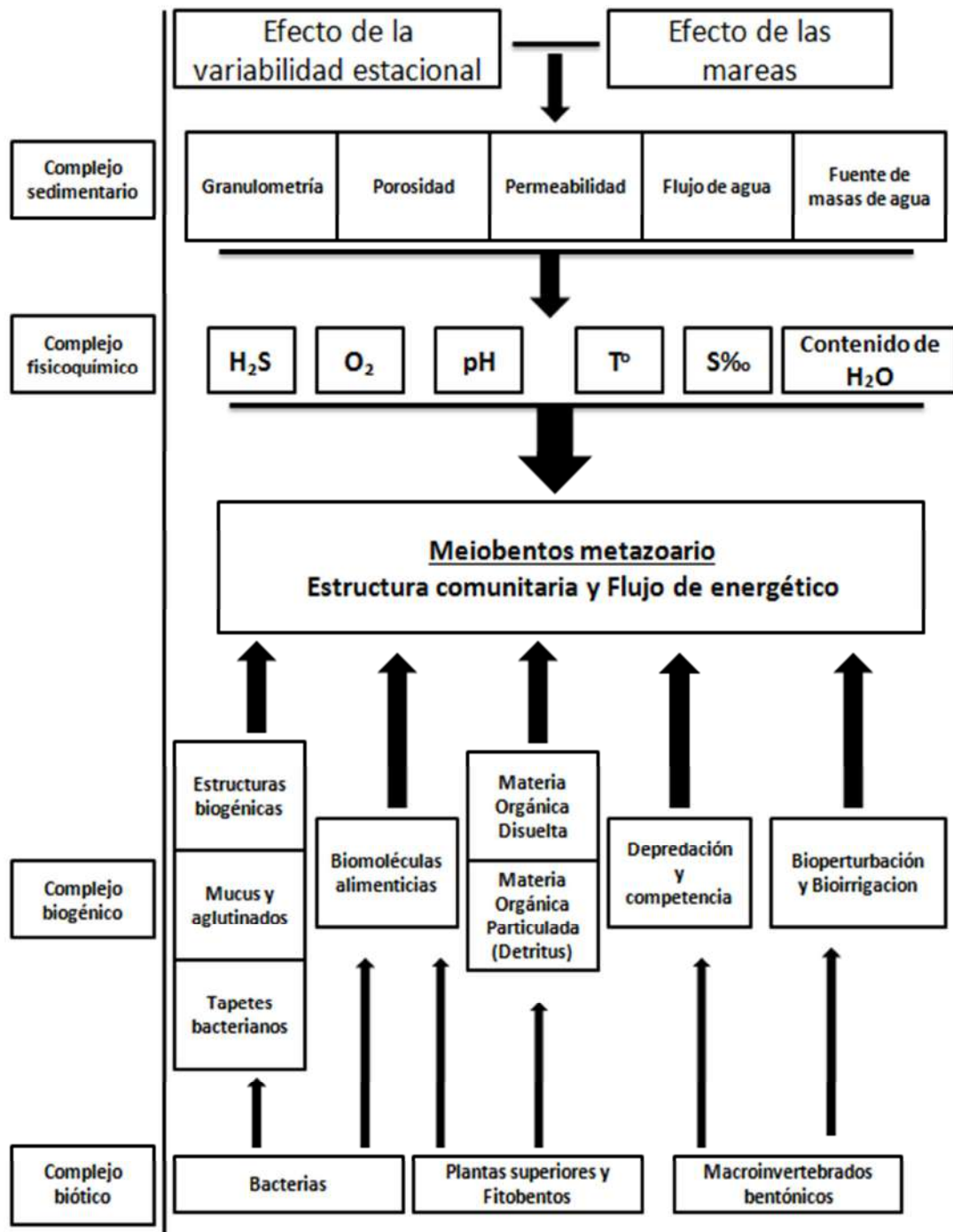
Figura 2. Factores que estructuran y modulan a la comunidad del meiobentos metazoario en el ecosistema de manglares (Modificado de Giere, 2009).
