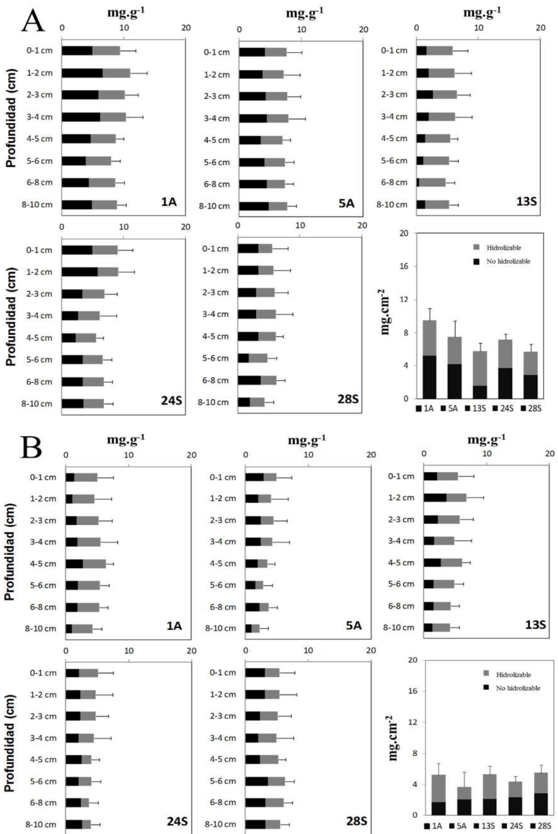
F8. Distribución vertical de las concentraciones hidrolizables y no hidrolizables de PRT (mg.g -1 ) ± SD en la columna de sedimento para las estaciones de muestreo dentro del SNLMT. A. Septiembre 2012, B. Abril 2013.
