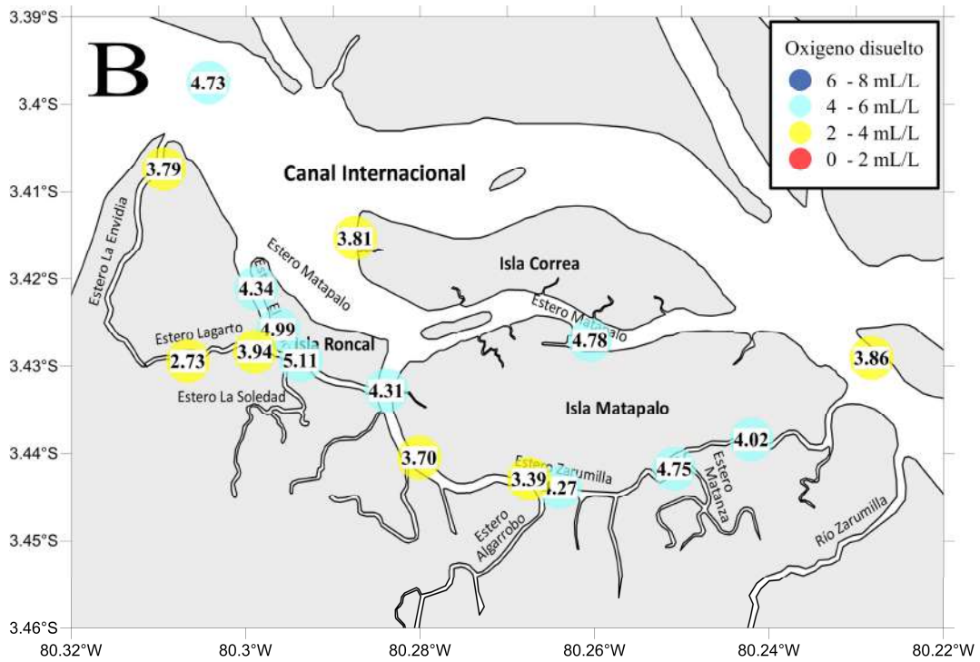
Figura 14. Oxígeno disuelto en columna de agua para las estaciones de muestreo dentro del SNLMT. A. Septiembre 2012, B. Abril 2013.
