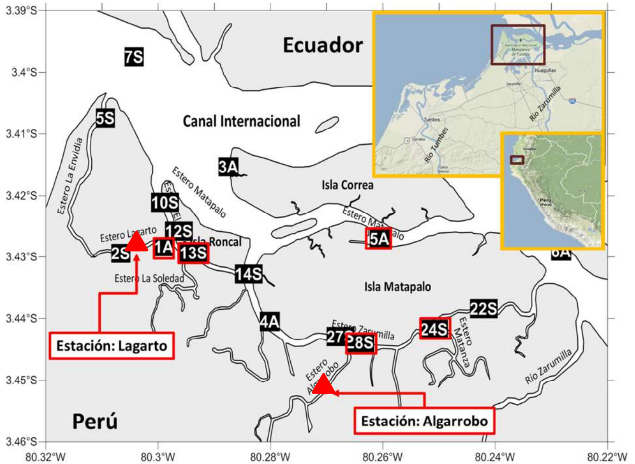
Figura 4. Extensión geográfica del Santuario Nacional “Manglares de Tumbes” (INRENA, 2011). Distribución de las estaciones de muestreo estacional (n= 16) determinadas en función al gradiente salino en el Santuario. Recuadros rojos: muestreo intensivo. Distribución de las estaciones del estudio de mareas. Triángulos rojos: Estero Lagarto y Algarrobo.
