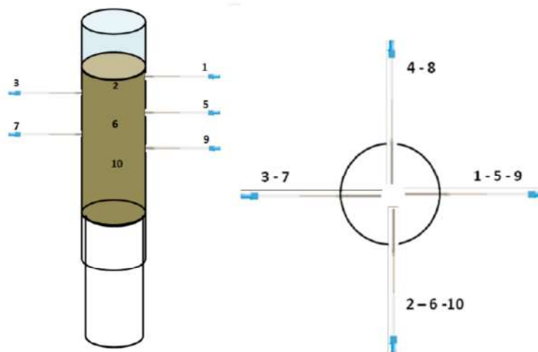
Figura 6. Secuencia de muestreo de agua intersticial mediante el uso de capilares micro porosos a partir de la columna de sedimento.
