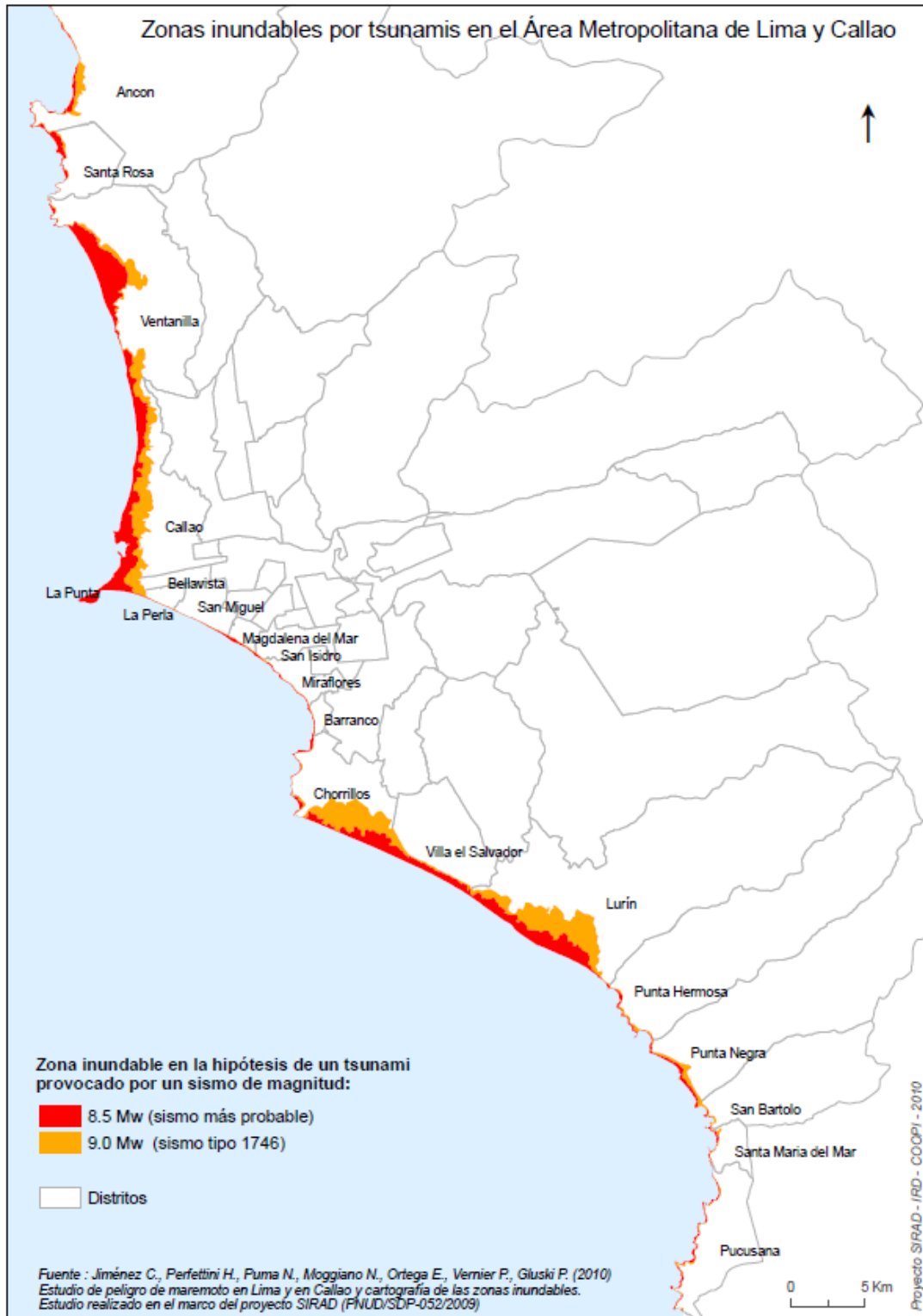
Figura 10.- Mapa de escenario de inundación por tsunami para la zona costera de Lima Metropolitana y El Callao considerando la ocurrencia de sismos de magnitud 8,5 y 9,0 Mw (COOPI, 2010).
