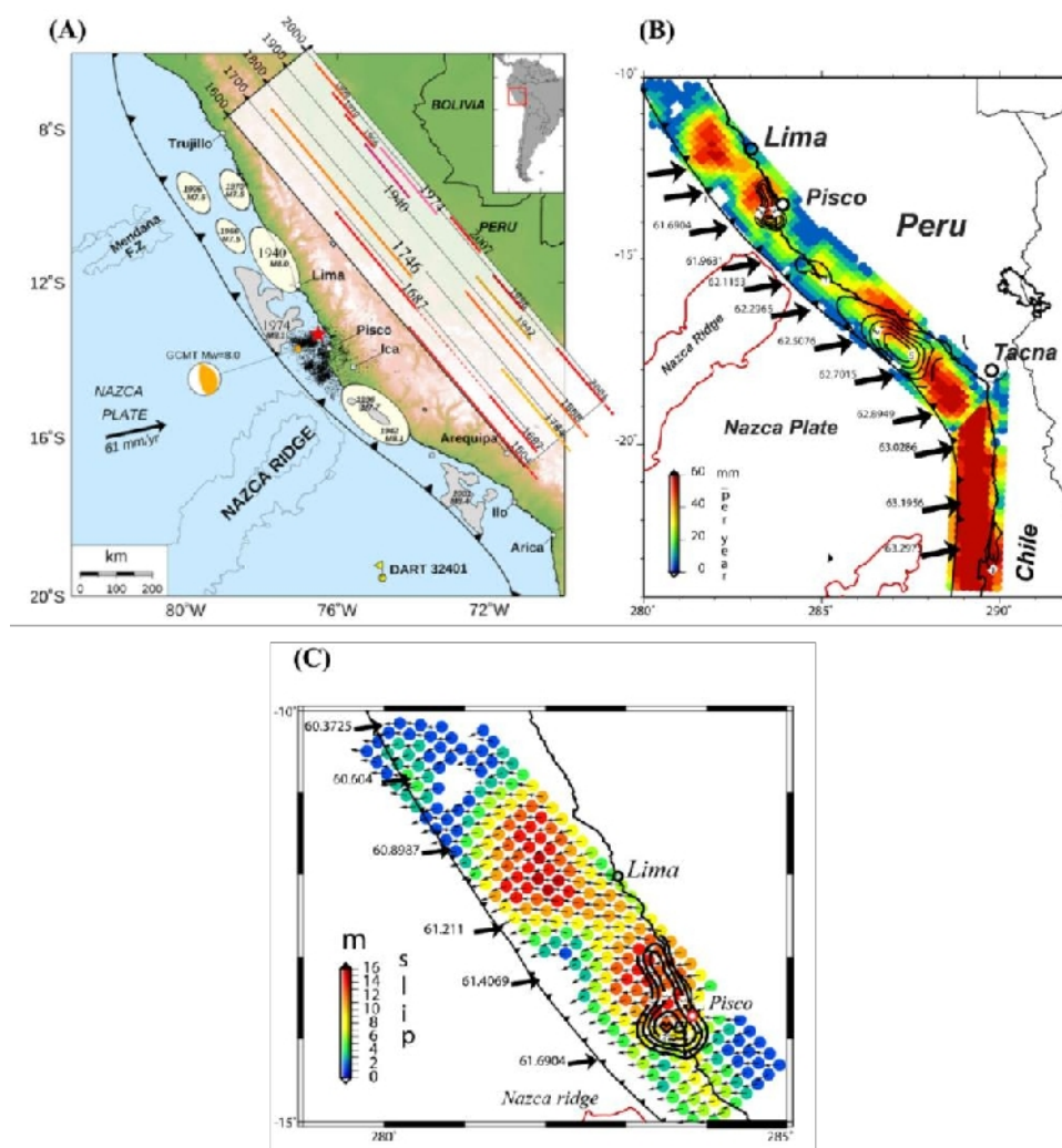
Figura 7: A) Sismos históricos en el borde occidental de Perú (Sladen et al., 2010). B) Modelo de déficit de deslizamiento en Perú y Chile. C) Distribución del vector deslizamiento obtenido al combinar la tasa de déficit de deslizamiento con un período intersísmico de 265 años correspondiente al terremoto de 1746 (Pulido et al, 2012).
