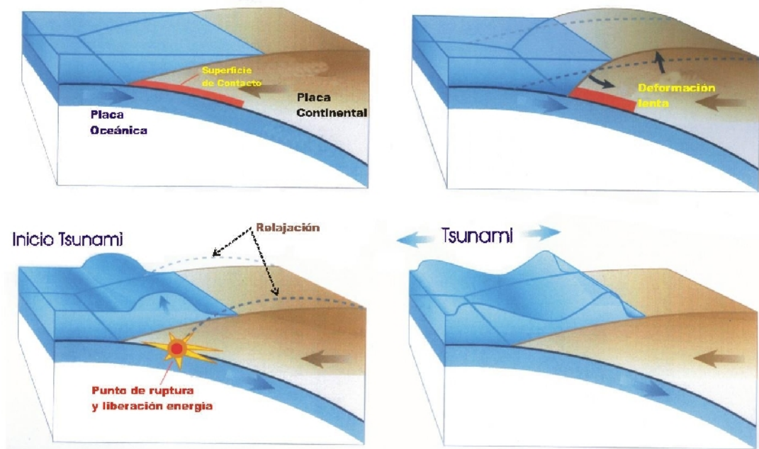
Figura 5: Esquema que muestra la convergencia de placas en el borde occidental del Perú y el proceso de generación de sismos y tsunamis. La línea en rojo representa al área de acoplamiento sísmico o de acumulación de energía. El proceso de subducción deforma el borde continental hasta un máximo de acumulación de energía que luego es liberada produciendo el sismo y tsunami.
