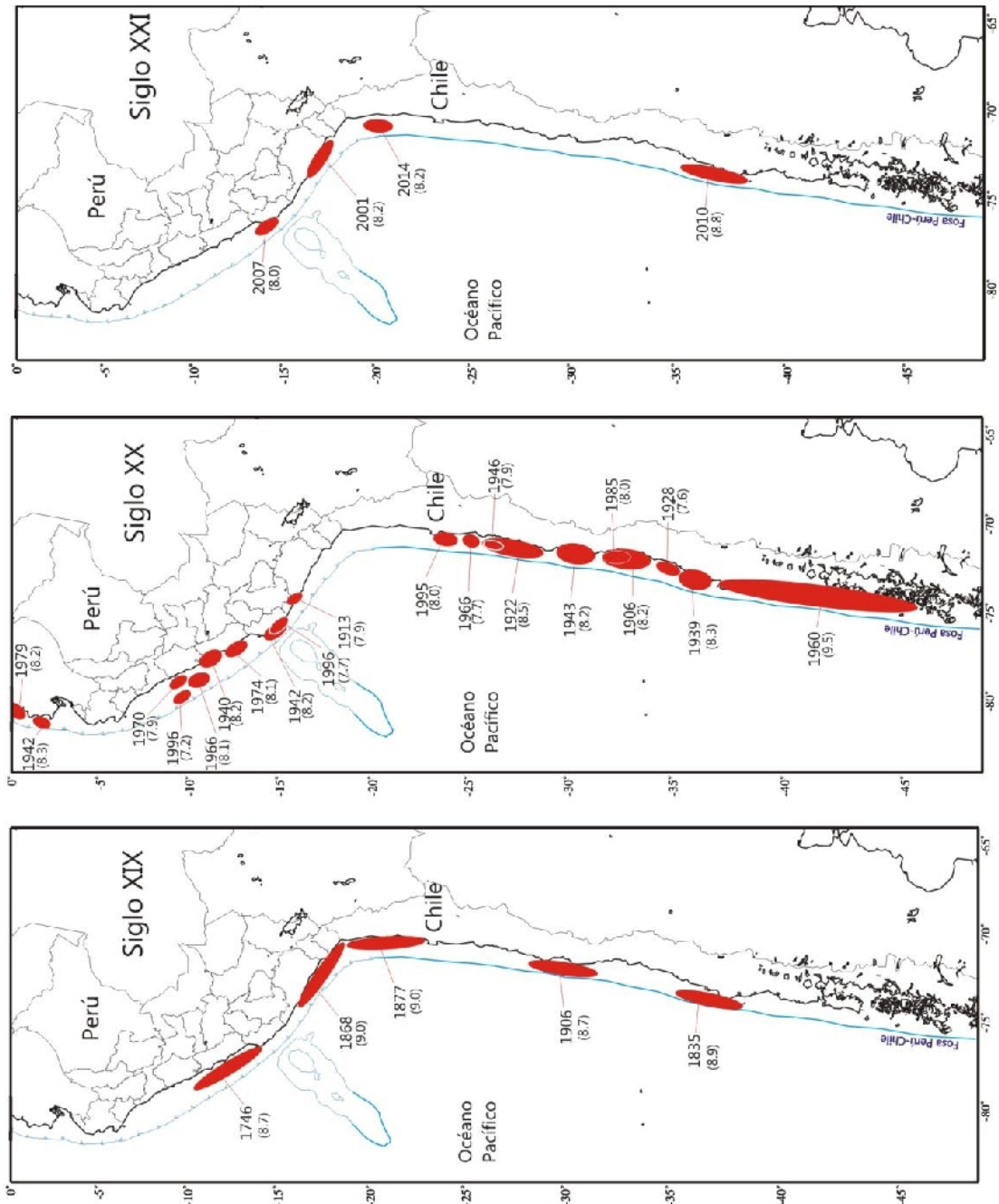
Figura 3: Bordo occidental de Perú y Chile, y distribución de áreas de ruptura y lagunas sísmicas durante los siglos XIX, XX y XXI. La magnitud de los sismos está expresada en la escala de magnitud momento (Mw). (Tavera y Bernal, 2005).
