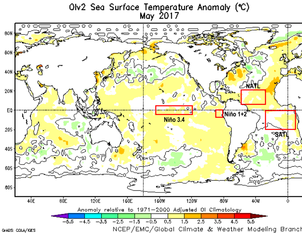
Fig. 1: Anomalías de temperatura superficial del mar (TSM) en °C del mes de mayo de 2017. Las anomalías son calculadas utilizando la climatología del periodo base 1971-2000. Fuente NOAA/NCEP.
