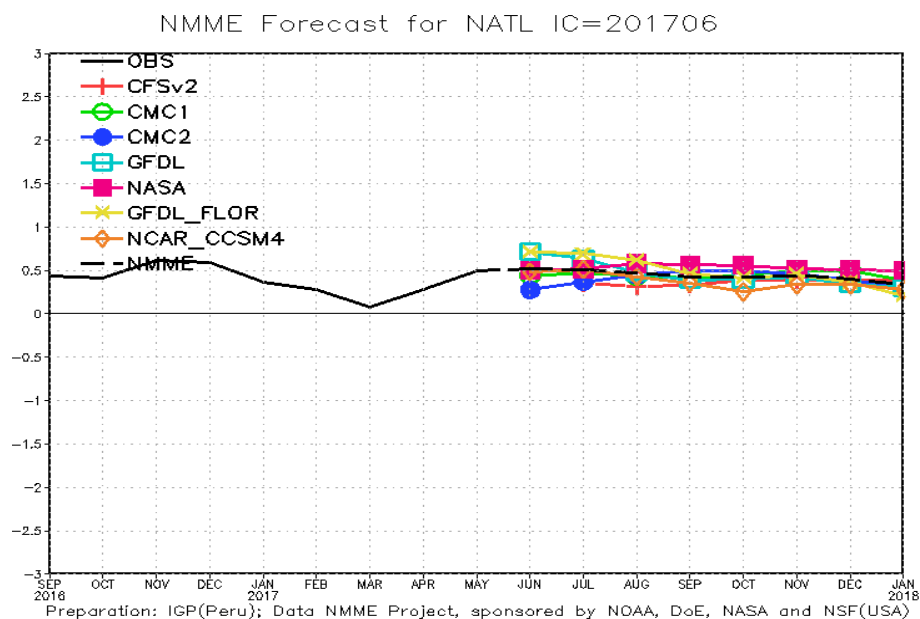
Fig. 9: Pronóstico de las anomalías de temperatura superficial del mar (TSM) para la región del Atlántico tropical Norte (NATL: 5°N-20°N, 30°W-60°W), a partir de condiciones de fines de mayo 2017. Fuente: Instituto Geofísico del Perú (IGP).
