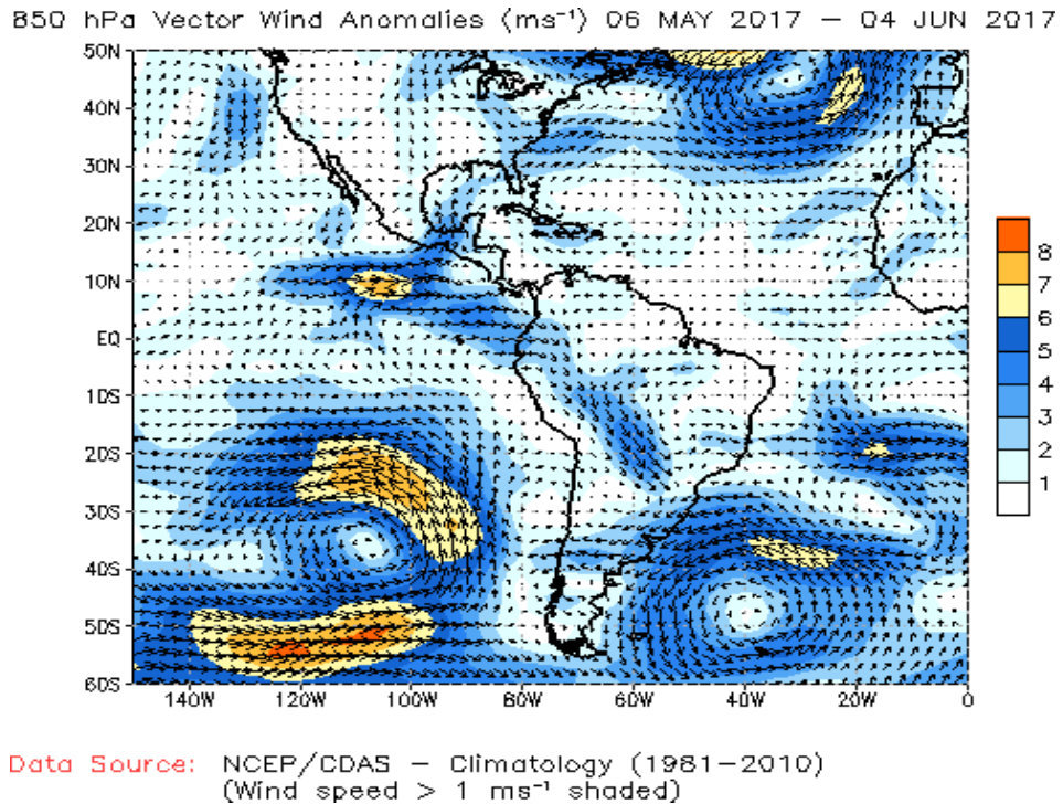
Fig. 2: Anomalia de vientos en niveles bajos (850 hPa) de la atmósfera, (del 06 de mayo al 04 de junio de 2017). Las anomalías fueron calculadas utilizando el periodo base los promedios entre 1981 y 2010. Fuente: NOAA/NCEP.
