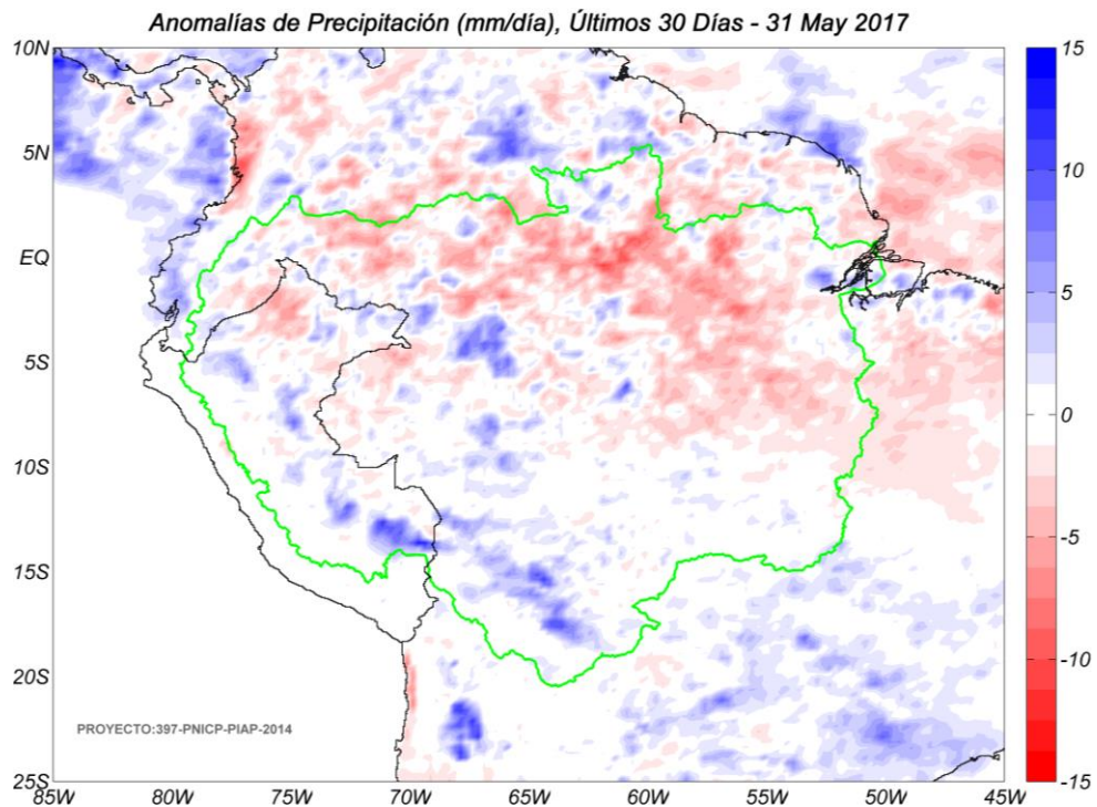
Fig. 4: Anomalías de precipitación estimadas por el TRMM-RT en mm/día hasta 31 de mayo de 2017. Las anomalías fueron calculadas con respecto al periodo base promedio 2000-2016. Se muestra los límites de la cuenca Amazónica en líneas de color verde. Las anomalías de precipitación del TRMM-RT actualizadas a tiempo real puede verse en: http://intranet.igp.gob.pe/eventos-extremos-amazonia-peruana/ .
