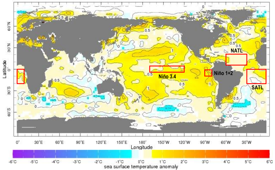
Fig. 7: Pronóstico de las anomalías de TSM (°C) a nivel global, para el trimestre junio-agosto (JJA) 2017. Rectángulos rojos indican regiones de análisis. Fuente: International Research Institute for Climate and Society (IRI) .
