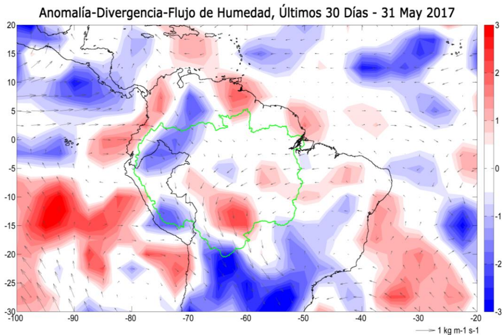
Fig. 3: Anomalías de flujo de humedad integrado en los niveles de 1000 hPa a 300 hPa de la atmósfera y su divergencia. El periodo corresponde de 01 al 31 de mayo 2017. Las anomalías son calculadas utilizando el periodo base de 1970 a 2016. Los límites de la cuenca Amazónica se muestran en línea verde.
