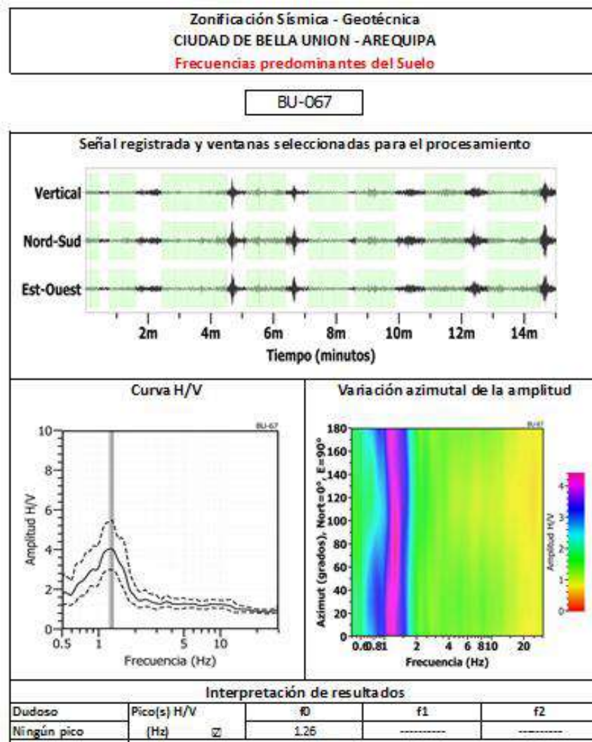
Figura 35: Ejemplo de la ficha H/V para el punto AC-46 en la cual se recopila la información registrada y analizada. Arriba, señal registrada; Medio; razón espectral (H/V) en línea gruesa y su desviación estándar en línea discontinua. Espectrograma y Abajo: resultados.
