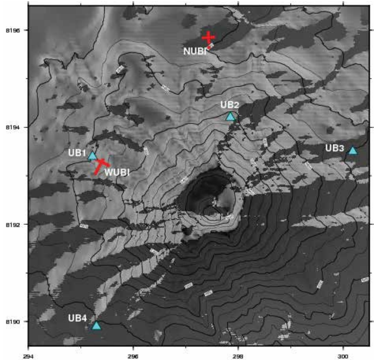
Figura 1. Topografía del volcán Ubinas, los puntos rojos son los sismómetros 3C del arreglo sísmico NUBI y WUBI instalados en el experimento del 2009, los triangulos verdes corresponden a las estaciones permanentes del IGP que viene funcionando desde el 2006.
