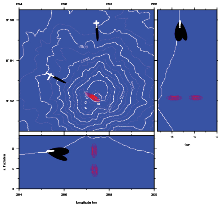
Figura 2. Localización de la explosiones vulcanianas en Ubinas, resultado de MUSIC-3C con los datos registrados en el experimento Ubinas 2009.
