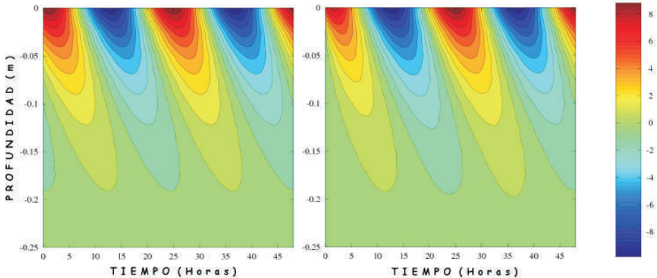
Figura 2. En la derecha se muestra la distribución de temperatura que se obtiene mediante el modelo numérico, y a la izquierda, la distribución de temperatura dada por la solución analítica. Ambas distribuciones corresponden al agua, donde no se considera las corrientes o flujos de este.
