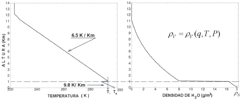
Figura 4. Perfiles estándar de temperatura ( ^\circ\text{K} ) y densidad de vapor de agua ( \text{g}/\text{m}^3 ) para las pruebas de sensibilidad de LW-I
