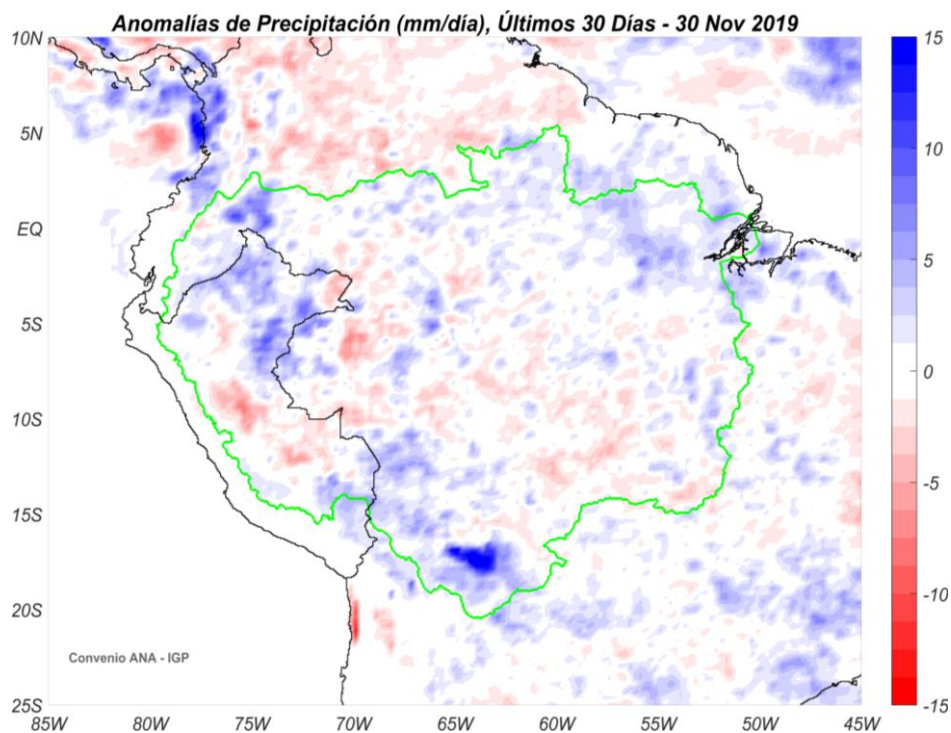
Fig. 4: Anomalías de precipitación estimadas por el TRMM-RT en mm/día hasta 30 de noviembre de 2019. Las anomalías fueron calculadas con respecto al periodo base promedio 2000-2018. Se muestra los límites de la cuenca Amazónica en líneas de color verde. Las anomalías de precipitación del TRMM-RT actualizadas a tiempo real puede verse en: http://intranet.igp.gob.pe/eventos-extremos-amazonia-peruana/ .
