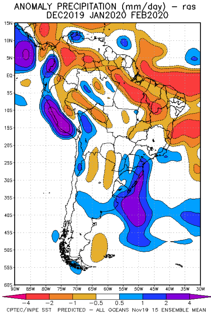
Fig. 10: Pronóstico de las anomalías de la precipitación (mm/día) método ras para el trimestre DEF del 2019-20 en América del Sur, con datos observados de fines del mes de noviembre de 2019. Fuente: CPTEC/INPE.
