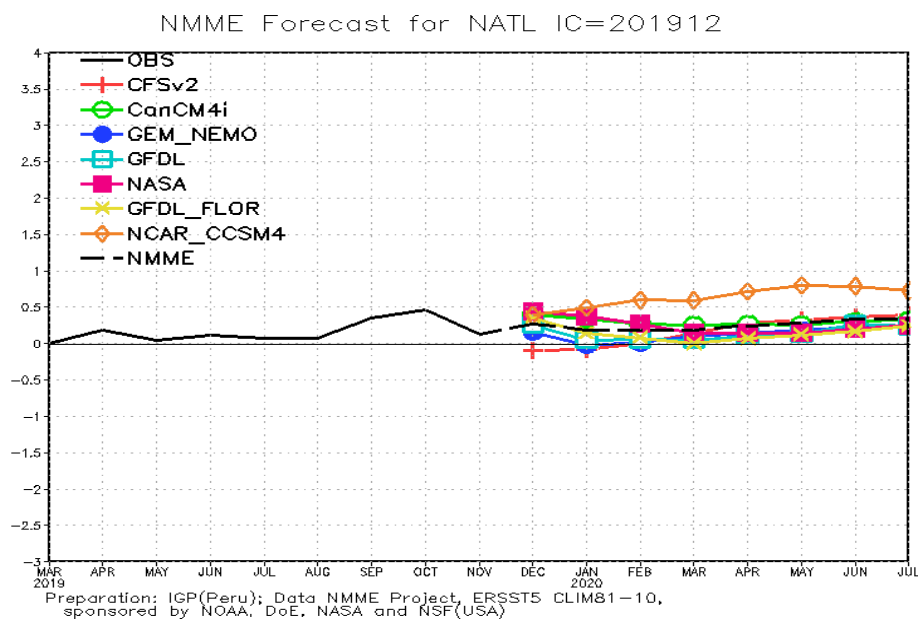
Fig. 9: Pronóstico de las anomalías de temperatura superficial del mar (TSM) para la región del Atlántico tropical Norte (NATL: 5°N-20°N, 30°W-60°W), a partir de condiciones de fines de noviembre 2019. Fuente: Instituto Geofísico del Perú (IGP) .
