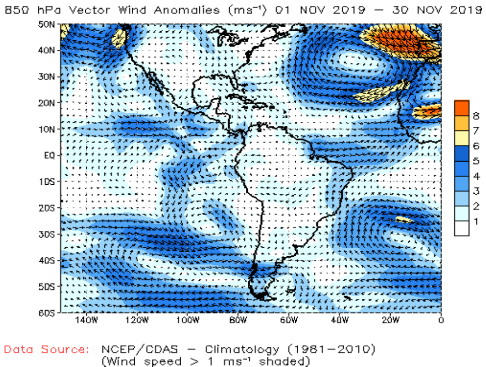
Fig. 2: Vectores de Anomalías de viento en niveles bajos (850 hPa) de la atmósfera, (del 01 noviembre al 30 de noviembre de 2019). Las anomalías fueron calculadas utilizando el periodo base los promedios entre 1981 y 2010. Fuente: NOAA/NCEP.
