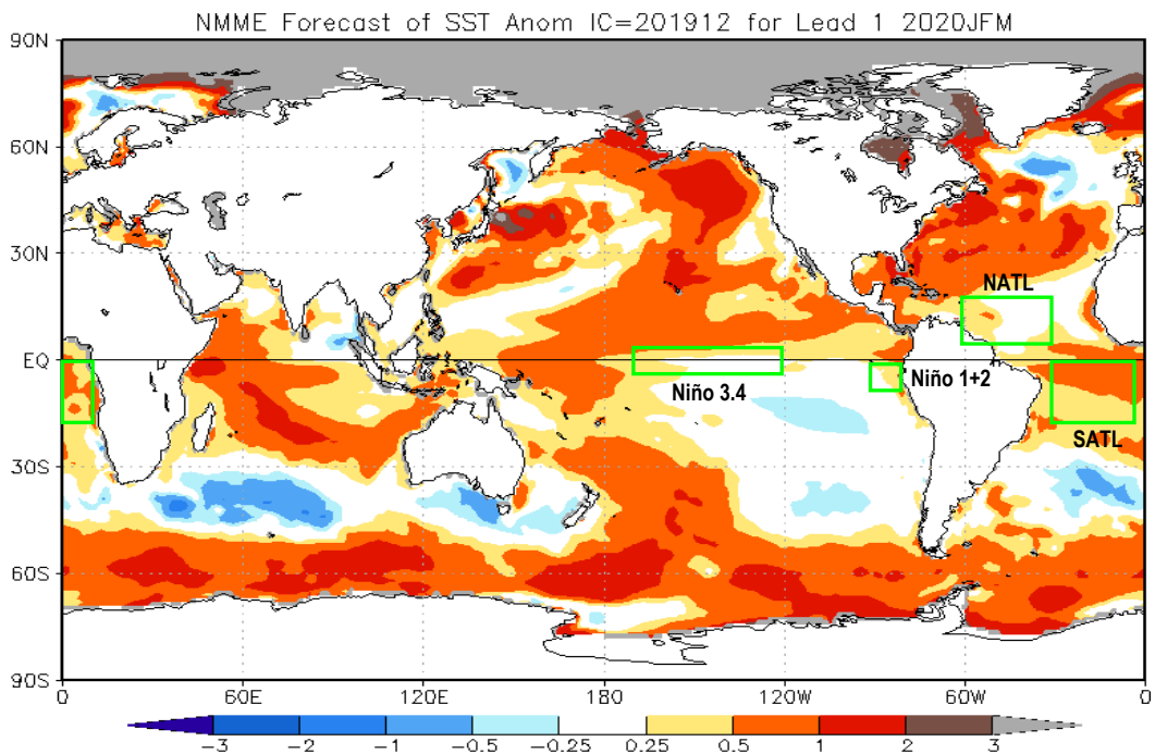
Fig. 7: Pronóstico de las anomalías de TSM (°C) a nivel global, para el trimestre enero-febrero-marzo 2020 (EFM). Rectángulos verdes indican regiones de análisis. Fuente: National Multi-Model Ensemble (NMME) .
