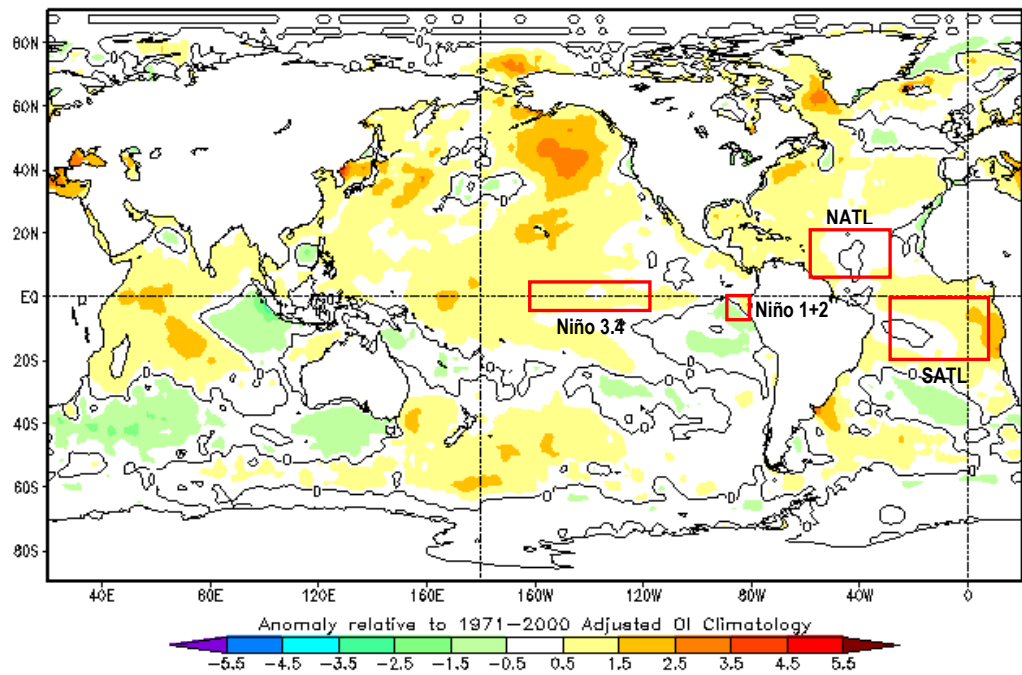
Fig. 1: Anomalías de temperatura superficial del mar (TSM) en °C del mes de noviembre de 2019. Las anomalías son calculadas utilizando la climatología del periodo base 1971-2000. Fuente CPTEC/INPE/BRASIL.
