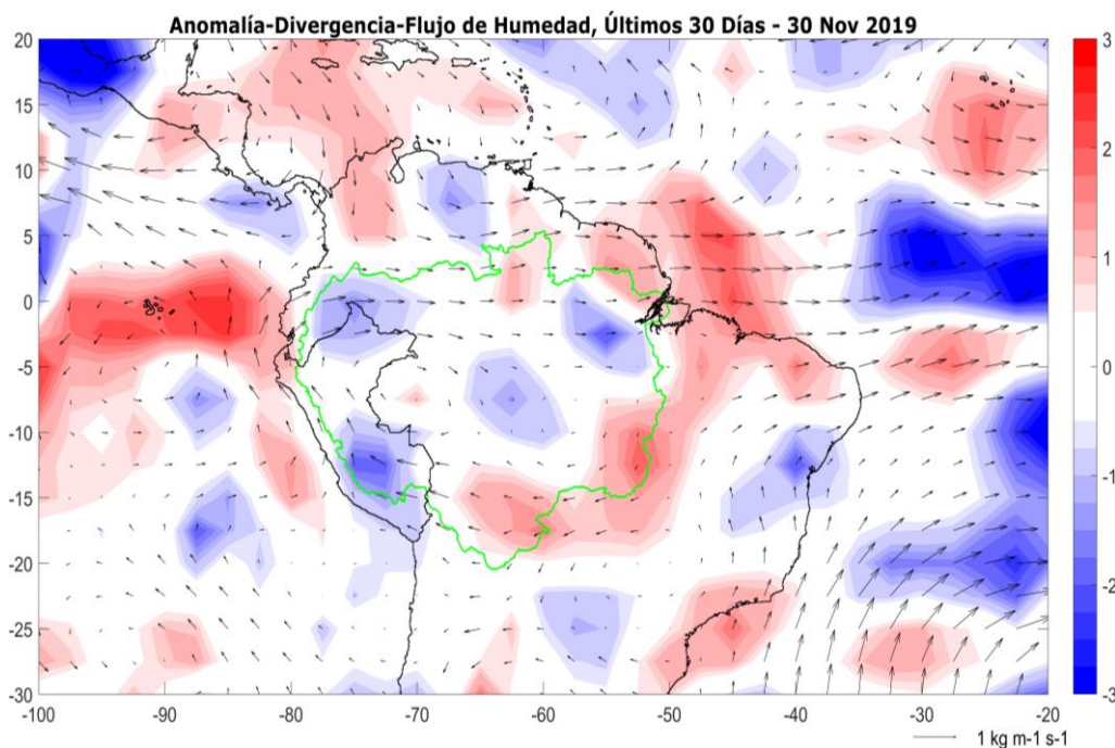
Fig. 3: Anomalías de flujo de humedad integrado en los niveles de 1000 hPa a 300 hPa de la atmósfera (vectores) y su divergencia (colores). El periodo corresponde del 01 al 30 de noviembre 2019. Las anomalías son calculadas utilizando el periodo base de 1970 a 2018. Los límites de la cuenca Amazónica se muestran en línea verde.
