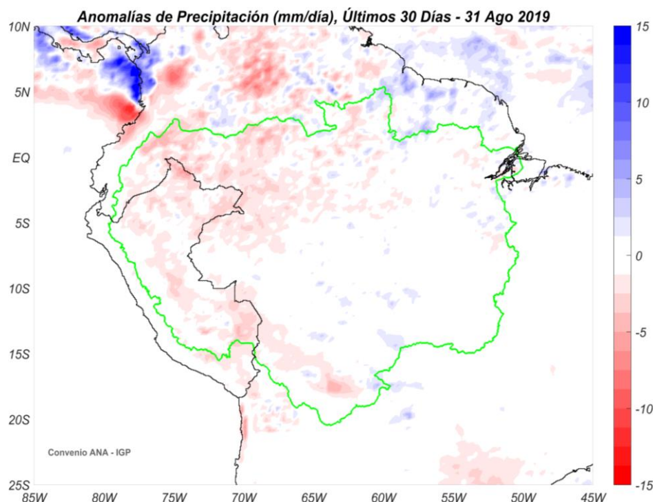
Fig. 4: Anomalías de precipitación estimadas por el TRMM-RT en mm/día hasta 31 de agosto de 2019. Las anomalías fueron calculadas con respecto al periodo base promedio 2000-2018. Se muestra los límites de la cuenca Amazónica en líneas de color verde. Las anomalías de precipitación del TRMM-RT actualizadas a tiempo real puede verse en: http://intranet.igp.gob.pe/eventos-extremos-amazonia-peruana/ .
