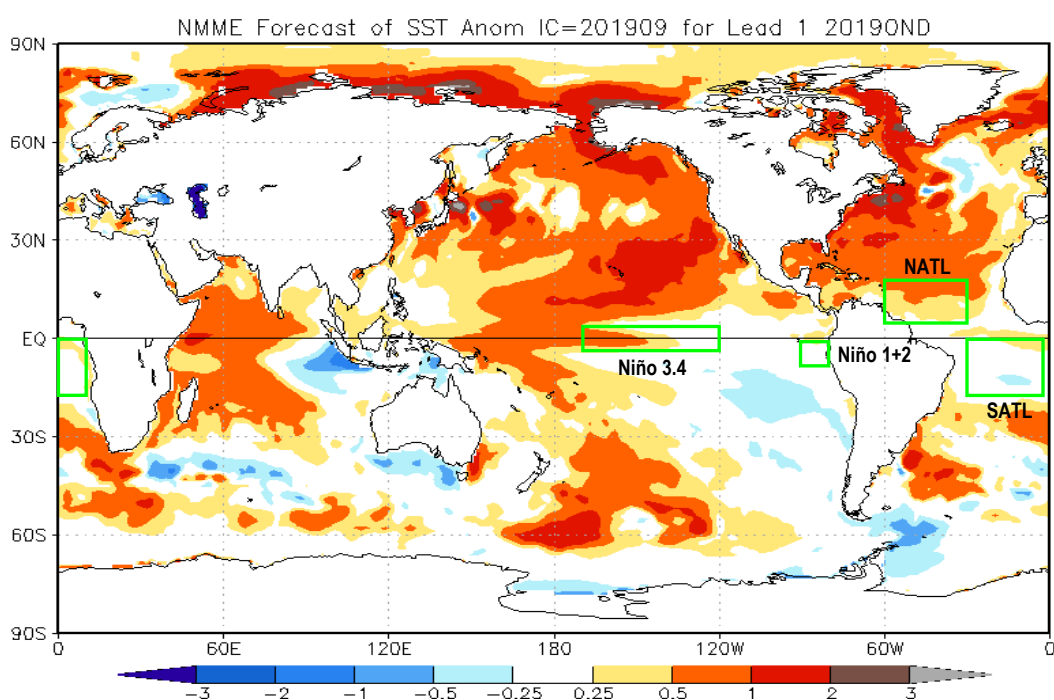
Fig. 7: Pronóstico de las anomalías de TSM (°C) a nivel global, para el trimestre octubre-noviembre-diciembre 2019 (OND). Rectángulos verdes indican regiones de análisis. Fuente: National Multi-Model Ensemble (NMME) .
