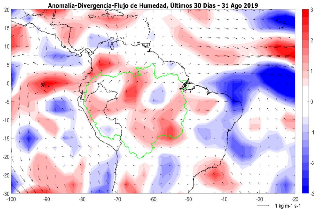
Fig. 3: Anomalías de flujo de humedad integrado en los niveles de 1000 hPa a 300 hPa de la atmósfera (vectores) y su divergencia (colores). El periodo corresponde del 01 hasta el 31 de agosto 2019. Las anomalías son calculadas utilizando el periodo base de 1970 a 2018. Los límites de la cuenca Amazónica se muestran en línea verde.
