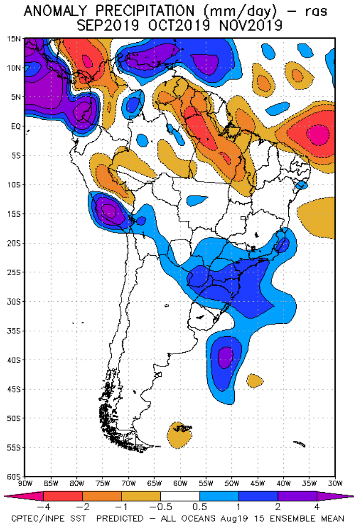
Fig. 10: Pronóstico de las anomalías de la precipitación (mm/día) método ras para el trimestre SON del 2019 en América del Sur, con datos observados de fines del mes de agosto de 2019. Fuente: CPTEC/INPE.
