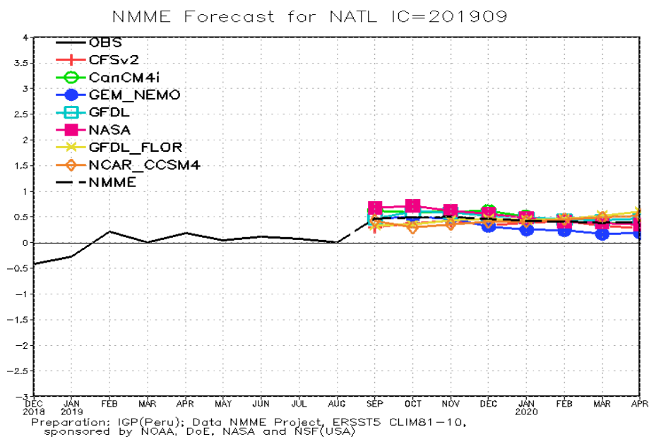
Fig. 9: Pronóstico de las anomalías de temperatura superficial del mar (TSM) para la región del Atlántico tropical Norte (NATL: 5°N-20°N, 30°W-60°W), a partir de condiciones de fines de agosto 2019. Fuente: Instituto Geofísico del Perú (IGP) .
