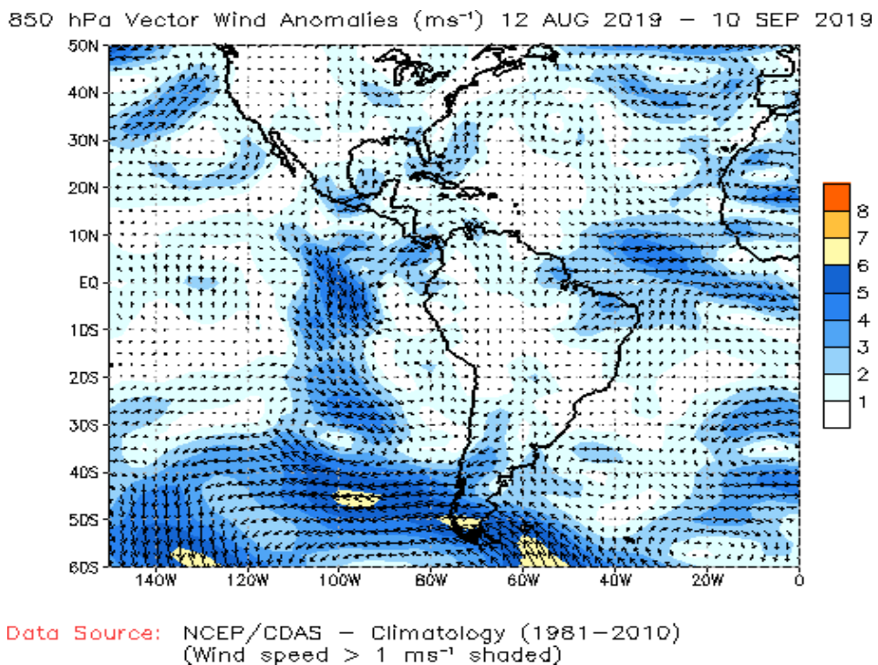
Fig. 2: Vectores de Anomalías de viento en niveles bajos (850 hPa) de la atmósfera, (del 12 de agosto al 10 de setiembre de 2019). Las anomalías fueron calculadas utilizando el periodo base los promedios entre 1981 y 2010. Fuente: NOAA/NCEP.
