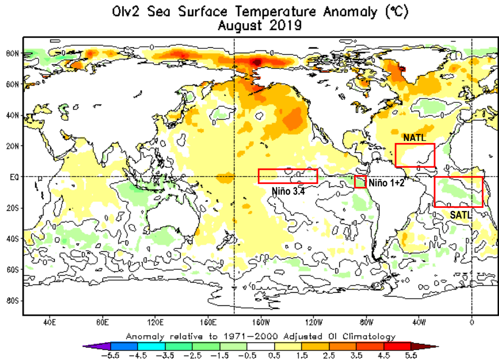
Fig. 1: Anomalías de temperatura superficial del mar (TSM) en °C del mes de agosto de 2019. Las anomalías son calculadas utilizando la climatología del periodo base 1971-2000. Fuente CPTEC/INPE/BRASIL.
