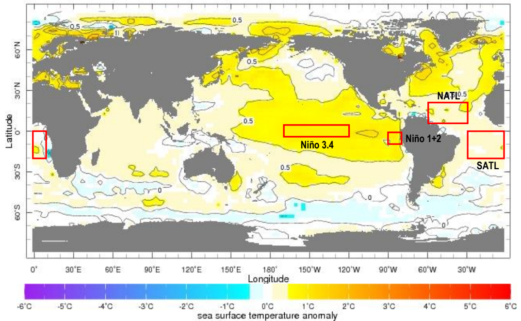
Fig. 7: Pronóstico de las anomalías de TSM (°C) a nivel global, para el trimestre octubre-diciembre (OND) 2017. Rectángulos rojos indican regiones de análisis. Fuente: International Research Institute for Climate and Society (IRI) .
