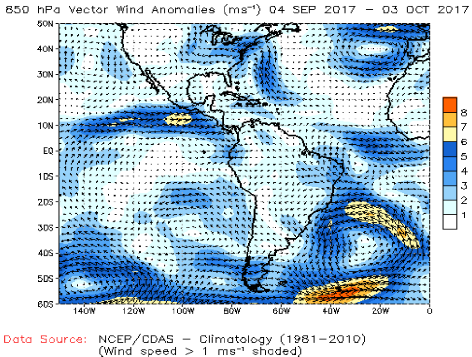
Fig. 2: Vectores de Anomalías de viento en niveles bajos (850 hPa) de la atmósfera, (del 04 de setiembre al 03 de octubre de 2017). Las anomalías fueron calculadas utilizando el periodo base los promedios entre 1981 y 2010. Fuente: NOAA/NCEP.
