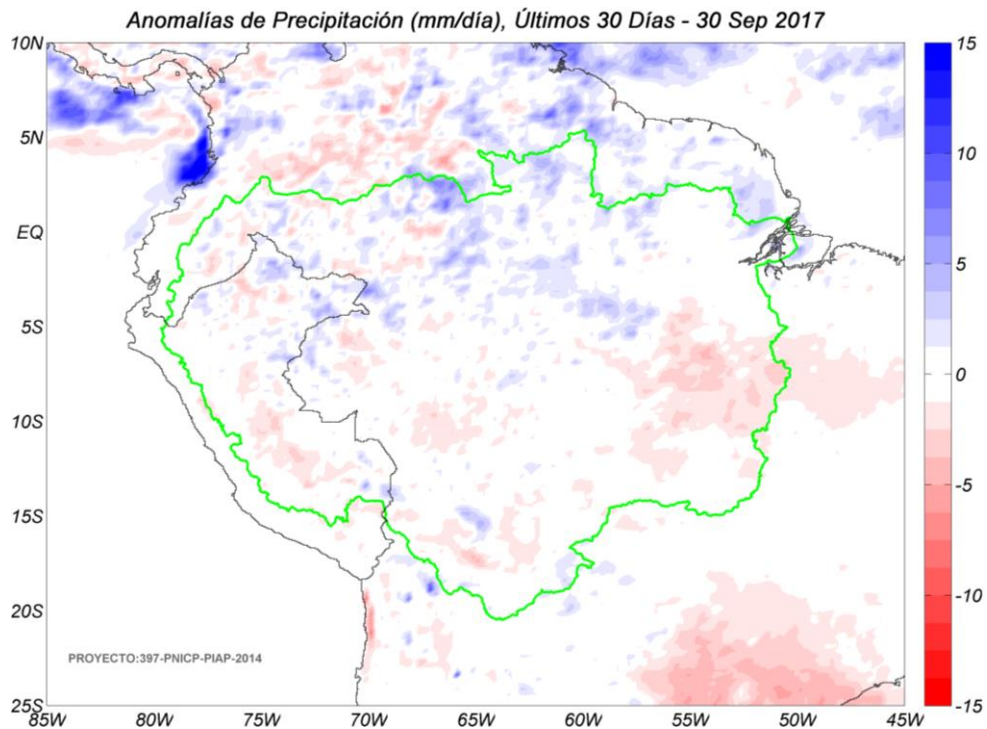
Fig. 4: Anomalías de precipitación estimadas por el TRMM-RT en mm/día hasta 30 de setiembre de 2017. Las anomalías fueron calculadas con respecto al periodo base promedio 2000-2016. Se muestra los límites de la cuenca Amazónica en líneas de color verde. Las anomalías de precipitación del TRMM-RT actualizadas a tiempo real puede verse en: http://intranet.igp.gob.pe/eventos-extremos-amazonia-peruana/ .
