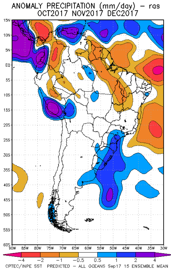
Fig. 10: Pronóstico de las anomalías de la precipitación (mm/día) método ras para el trimestre OND del 2017 en América del Sur, con datos observados del mes de setiembre. Fuente: CPTEC/INPE.
