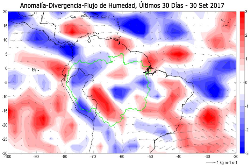
Fig. 3: Anomalías de flujo de humedad integrado en los niveles de 1000 hPa a 300 hPa de la atmósfera (vectores) y su divergencia (colores). El periodo corresponde de 01 al 30 de setiembre 2017. Las anomalías son calculadas utilizando el periodo base de 1970 a 2016. Los límites de la cuenca Amazónica se muestran en línea verde.
