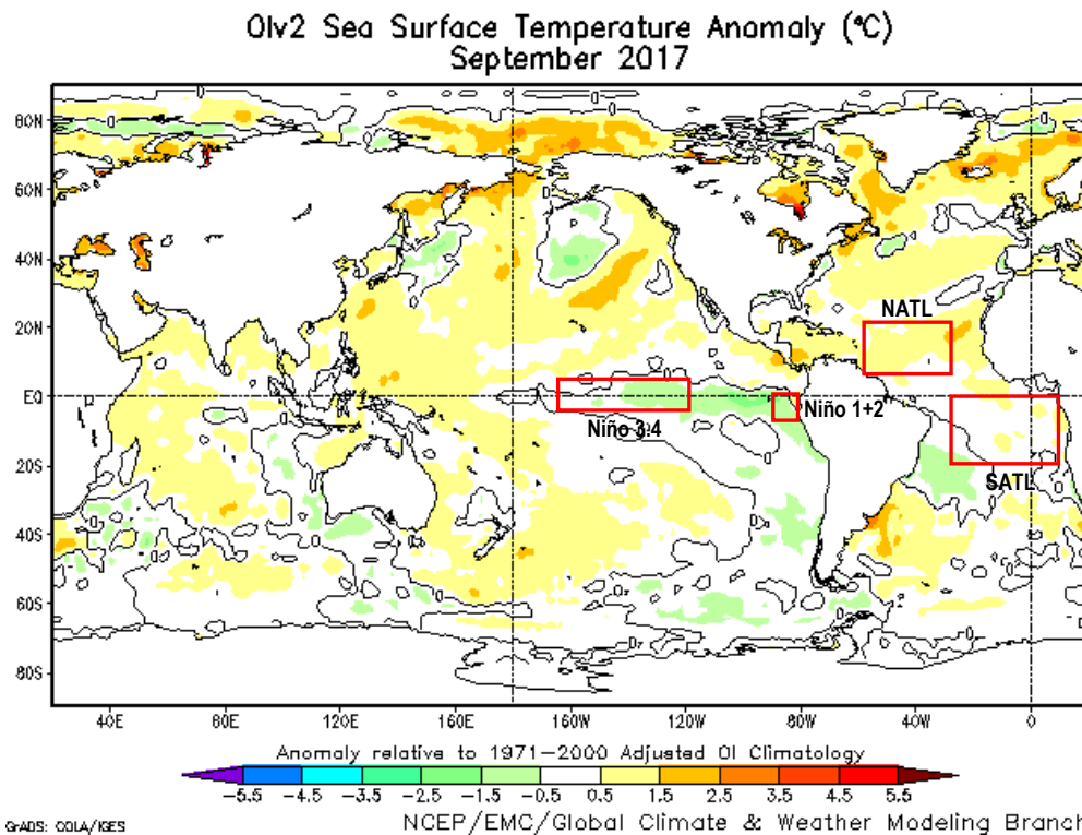
Fig. 1: Anomalías de temperatura superficial del mar (TSM) en °C del mes de setiembre de 2017. Las anomalías son calculadas utilizando la climatología del periodo base 1971-2000. Fuente NOAA/NCEP.
