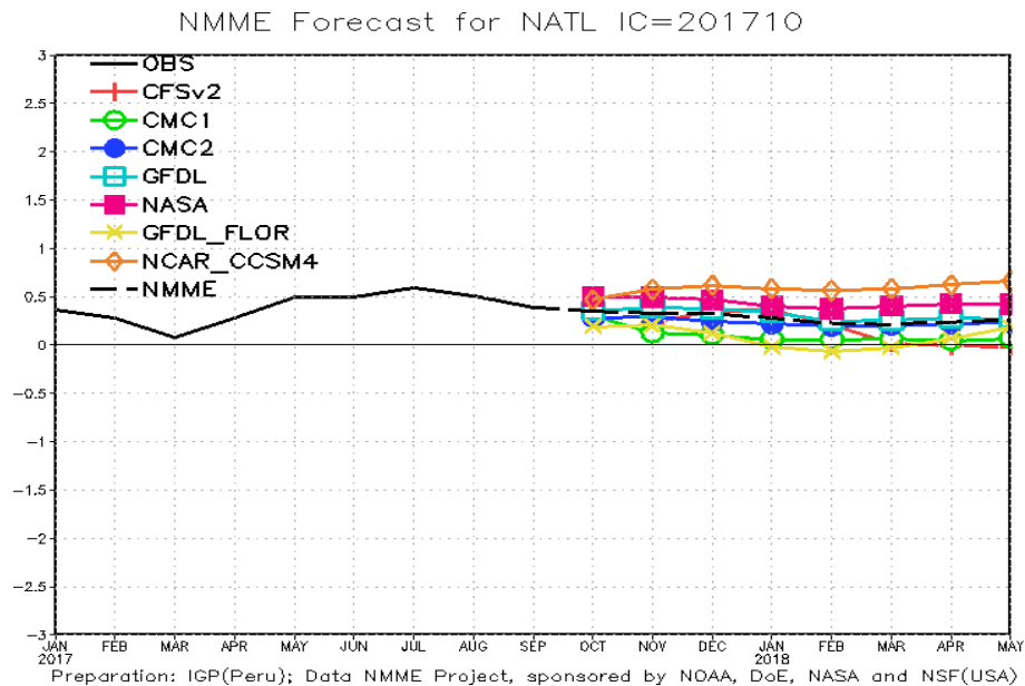
Fig. 9: Pronóstico de las anomalías de temperatura superficial del mar (TSM) para la región del Atlántico tropical Norte (NATL: 5°N-20°N, 30°W-60°W), a partir de condiciones de fines de setiembre 2017. Fuente: Instituto Geofísico del Perú (IGP).
