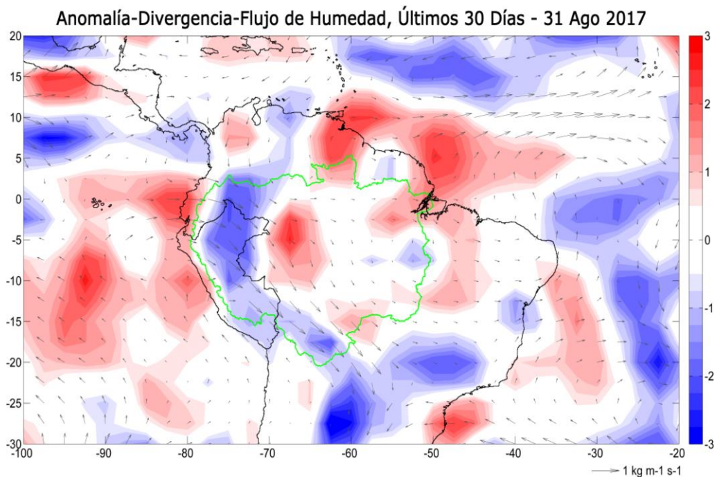
Fig. 3: Anomalías de flujo de humedad integrado en los niveles de 1000 hPa a 300 hPa de la atmósfera y su divergencia. El periodo corresponde de 01 al 31 de agosto 2017. Las anomalías son calculadas utilizando el periodo base de 1970 a 2016. Los límites de la cuenca Amazónica se muestran en línea verde.
