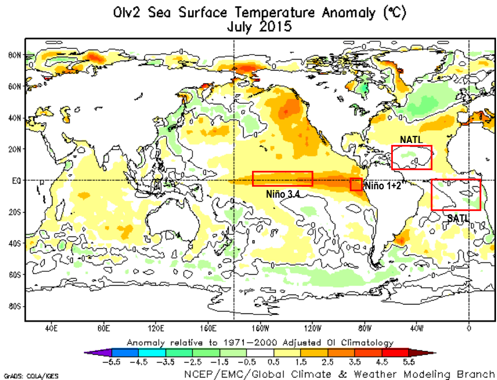
Fig. 1: Anomalías de temperatura superficial del mar (TSM) en °C del mes de julio de 2015. Las anomalías son calculadas utilizando la climatología del periodo base 1971-2000. Fuente NOAA/NCEP.
