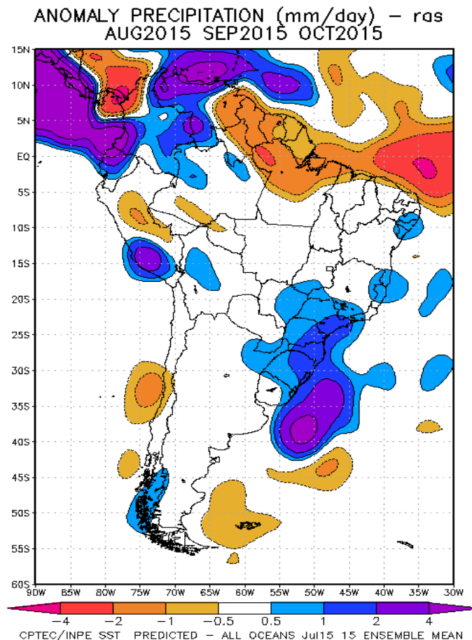
Fig. 10: Pronóstico de las anomalías de la precipitación (mm/día) método ras para el trimestre ASO del 2015 en América del Sur, con datos observados del mes de julio. Fuente: CPTEC/INPE.
