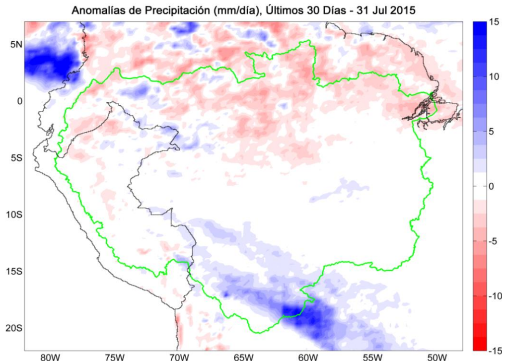
Fig. 4: Anomalías de precipitación estimadas por el TRMM-RT en mm/día para julio de 2015. Las anomalías fueron calculadas con respecto al periodo base promedio 2000-2014. Se muestra límites de la cuenca Amazónica en línea verde. Las anomalías de precipitación del TRMM-RT actualizadas a tiempo real puede verse en: http://www.igp.gob.pe/eventos-extremos-amazonia-peruana/
