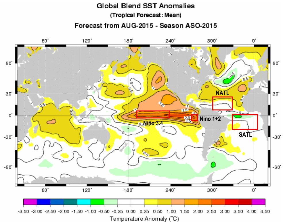
Fig. 7: Pronóstico de las anomalías de temperatura superficial del mar ( ^{\circ}\text{C} ) a nivel global, para el trimestre agosto-octubre (ASO). Rectángulos rojos indican regiones de análisis. Fuente: International Research Institute for Climate and Society (IRI).
