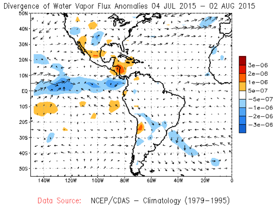
Fig. 3: Anomalías de flujo de humedad integrado en los niveles de 1000 hPa a 300 hPa de la atmósfera y su divergencia. El periodo corresponde de 04 de julio al 02 de agosto 2015. Las anomalías son calculadas utilizando el periodo base de 1979 a 1995. Fuente: NOAA/NCEP.
