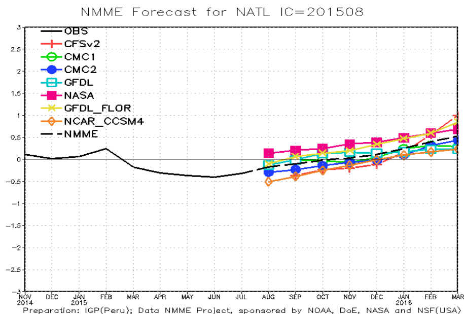
Fig. 9: Pronóstico de las anomalías de temperatura superficial del mar (TSM) para la región del Atlántico tropical Norte (NATL: 5°N-20°N, 30°W-60°W), a partir de condiciones de fines de julio 2015. Fuente: Instituto Geofísico del Perú (IGP).
