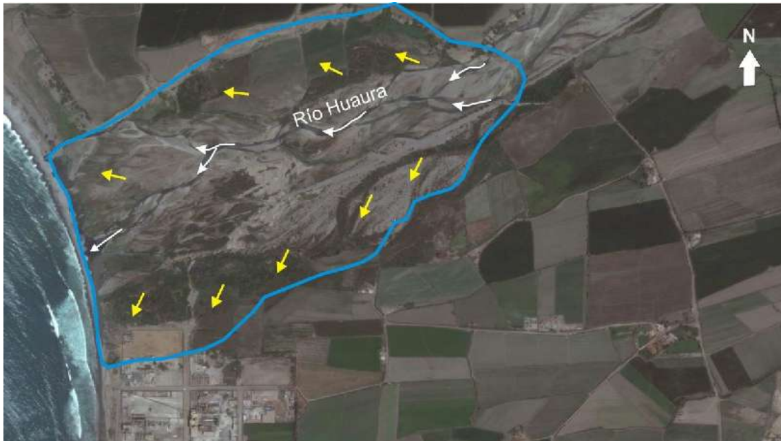
Figura 47: El polígono de color celeste indica el área susceptible a inundaciones por desborde del río Huaura. Las flechas en blanco indican la dirección natural del agua y las amarillas, la dirección preferente del desborde.
