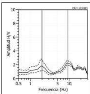
Figura 60: ...Continuación/ Ejemplos de razones espectrales (H/V) en el rango de las frecuencias predominantes F1 ( F > 3.0\text{Hz} ) obtenidas para los puntos ubicados en el centro de la ciudad de Huacho, próximos a la línea de costa.
