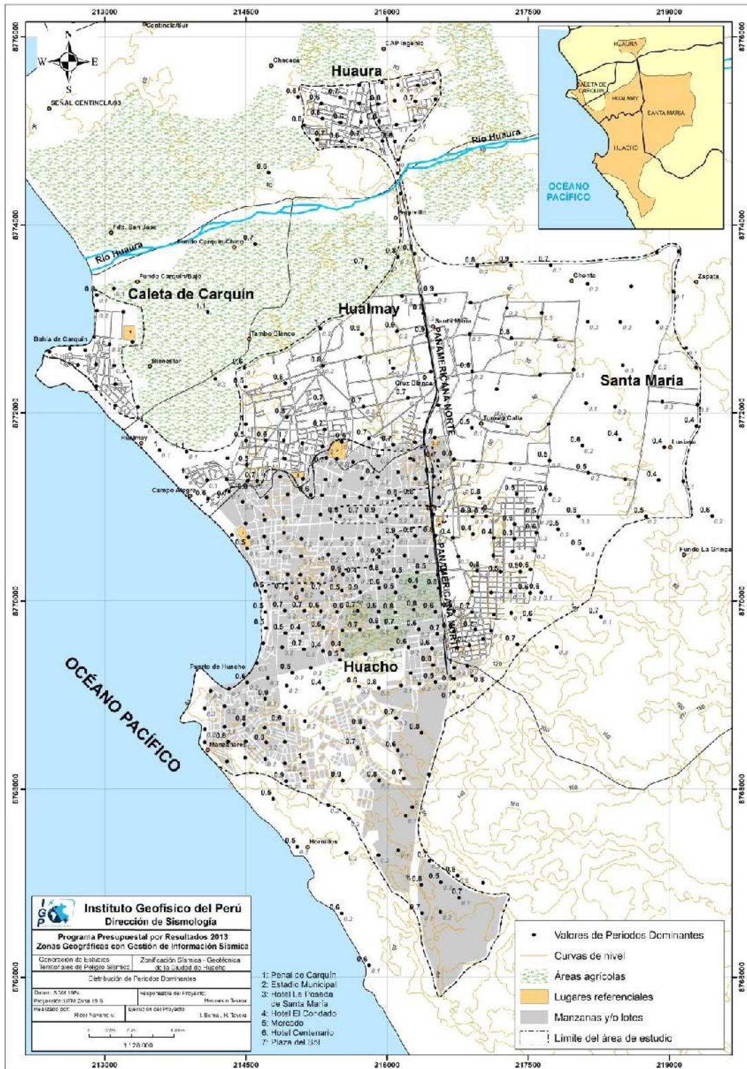
Figura 61: Mapa del área de estudio (ciudad de Huacho) y distribución espacial de los valores de periodos dominantes. La línea discontinua delimita a los puntos con periodos menores o iguales a 0.2 segundos y A_{max} \leq 2 veces
