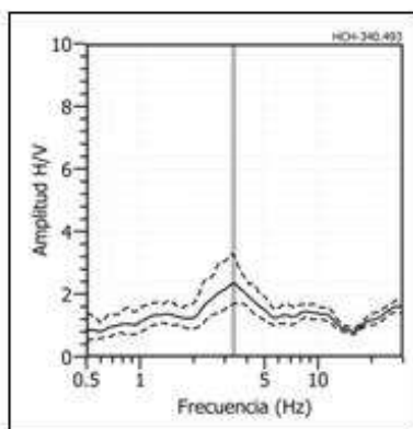
Figura 60: ...Continuación/ Ejemplos de razones espectrales (H/V) en el rango de las frecuencias predominantes F1 ( F > 3.0\text{Hz} ) obtenidas para los puntos ubicados en Huaura.
