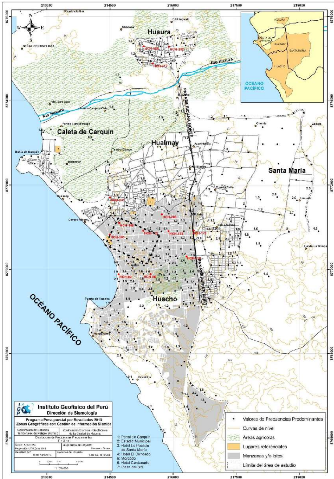
Figura 57: Mapa de la ciudad de Huacho y distribución espacial de las frecuencias predominantes F < 3.0 Hz). Los puntos rojos corresponden a ejemplos de H/V de la Figura 58. La línea discontinua delimita el área con mínimas amplificaciones.
