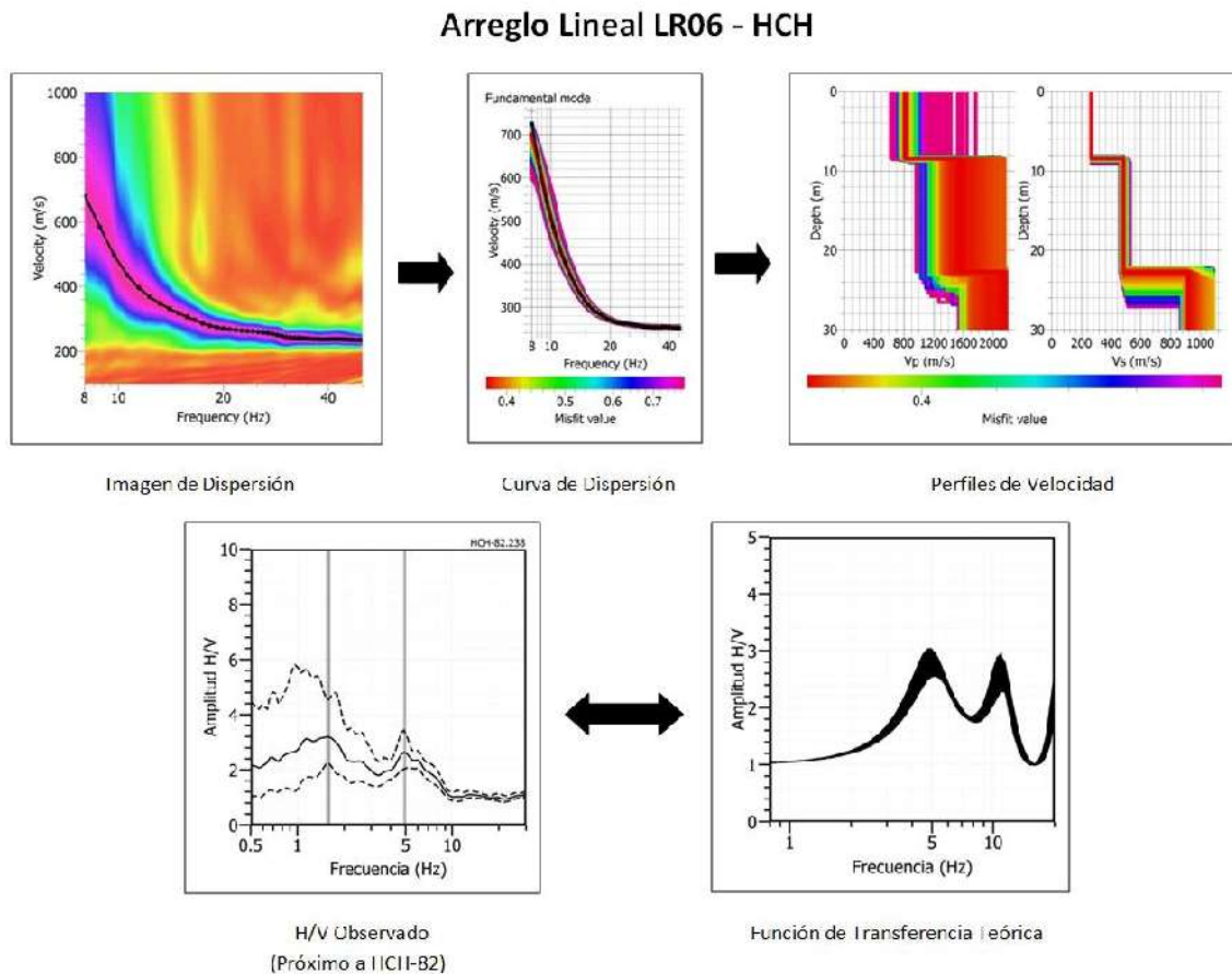
Figura 64d: Análisis e interpretación geofísica obtenido con el método MASW para el arreglo LR06–HCH (ver Figura 62)
