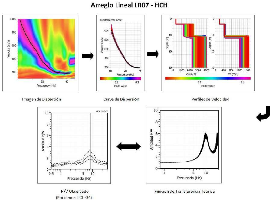
Figura 64g: Análisis e interpretación geofísica obtenido con el método MASW para el arreglo LR07–HCH (ver Figura 62)
