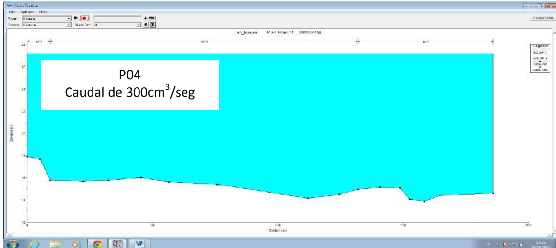
Figura 50: Modelado de inundación en el río Huaura considerando un caudal máximo de 300 \text{ m}^3/\text{seg} .
