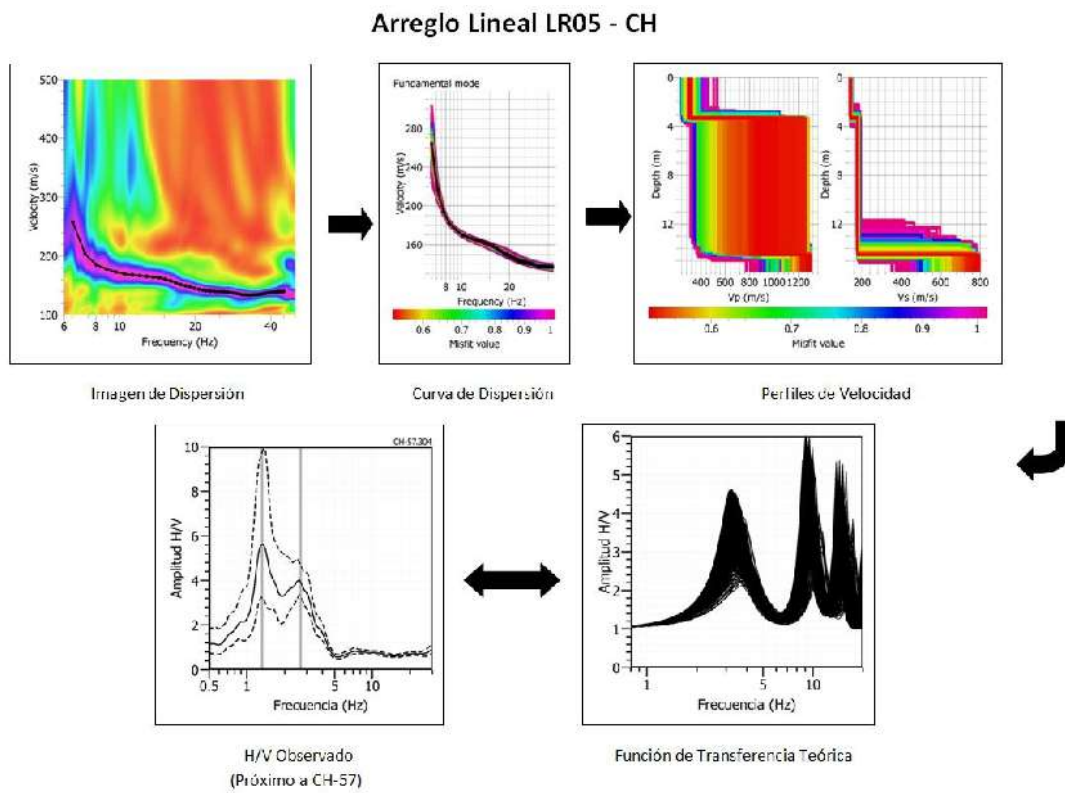
Figura 72d: Análisis e interpretación geofísica obtenida con el método MASW para el arreglo LR05-CH.
