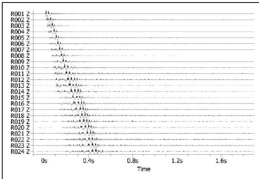
Figura 71: Disposición del equipo de refracción sísmica y registros obtenidos en la ciudad de Chimbote
