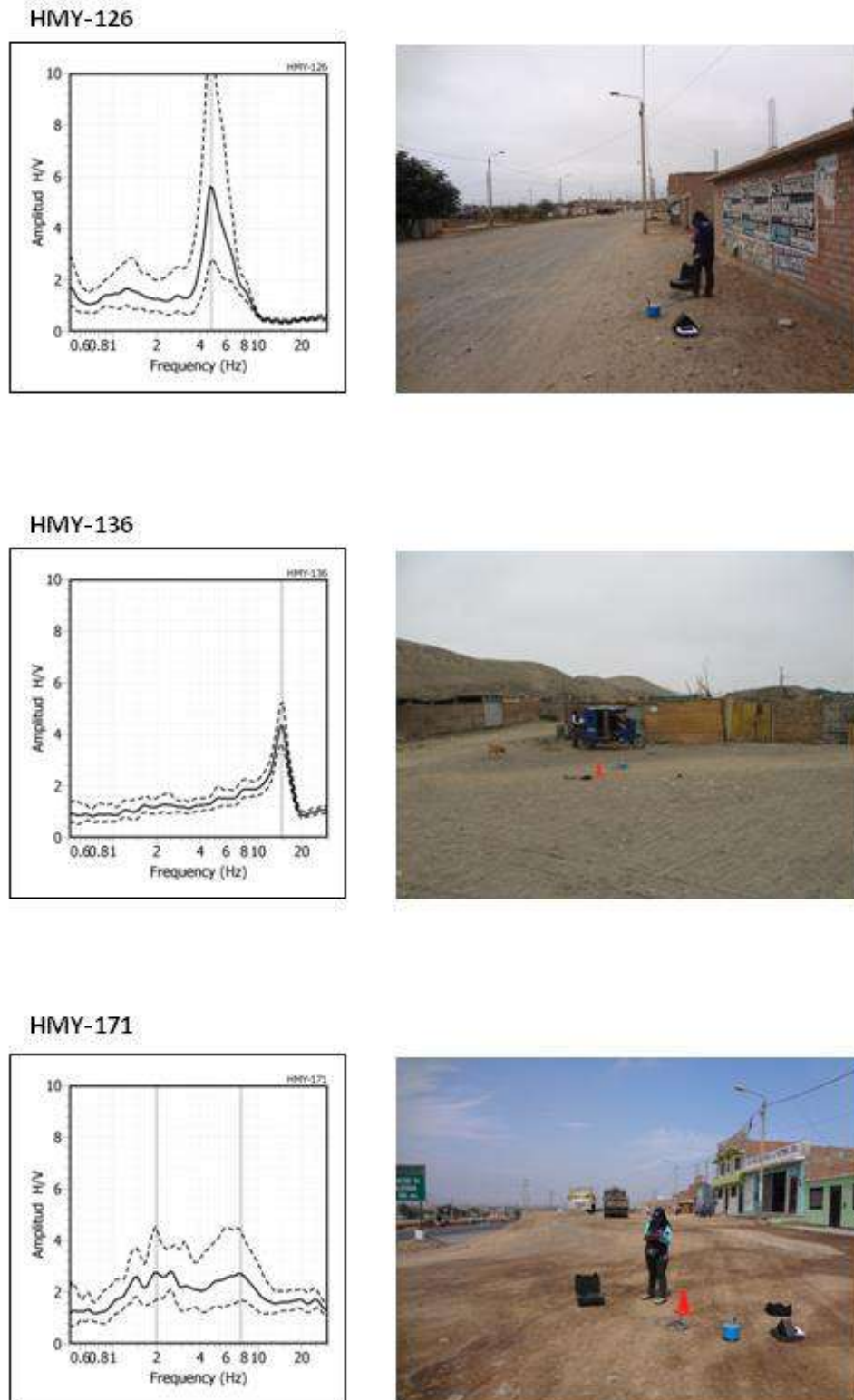
Figura 51: Continuación.../ Ejemplos de razones espectrales (H/V) para puntos ubicados en el extremo NO de la ciudad de Huarmey. Las líneas continuas representan la razón espectral y las discontinuas su desviación estándar. Las barras grises, definen la frecuencia predominante.
